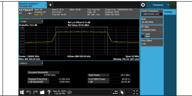
Band2-10MHz-16QAM-18900-50RB#0-PASS
