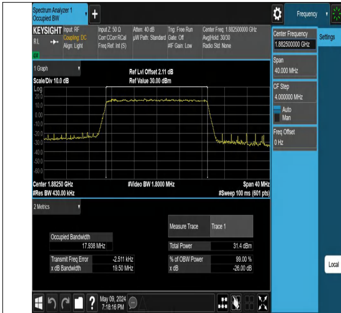
Band25-20MHz-QPSK-26365-100RB#0-PASS
