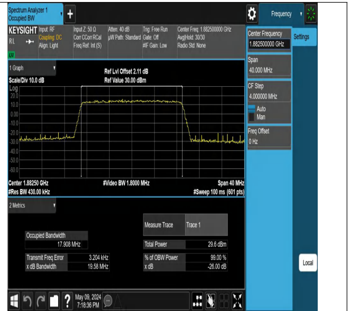
Band25-20MHz-64QAM-26365-100RB#0-PASS
