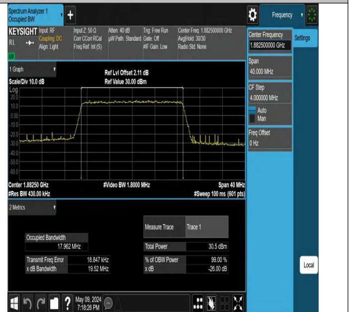
Band25-20MHz-16QAM-26365-100RB#0-PASS
