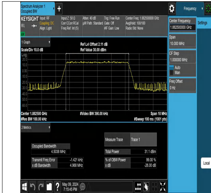
Band25-5MHz-QPSK-26365-25RB#0-PASS
