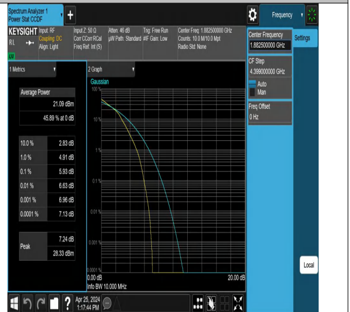
Band25-10MHz-16QAM-26365-50RB#0-PASS
