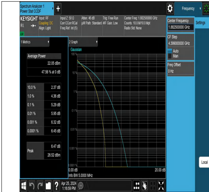
Band25-5MHz-QPSK-26365-25RB#0-PASS
