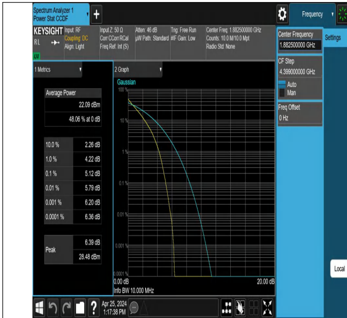
Band25-10MHz-QPSK-26365-50RB#0-PASS
