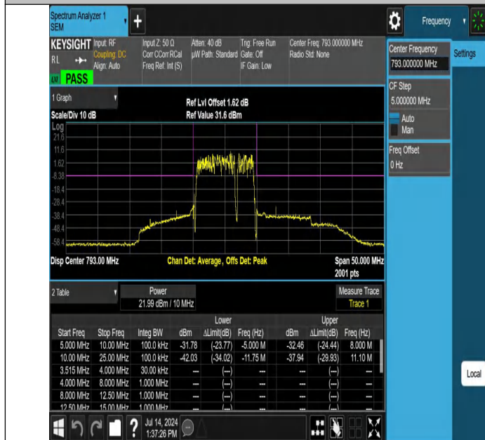
NTNV-Band14-10MHz-QPSK-23330-50RB#0--25.00--10.00-PASS
