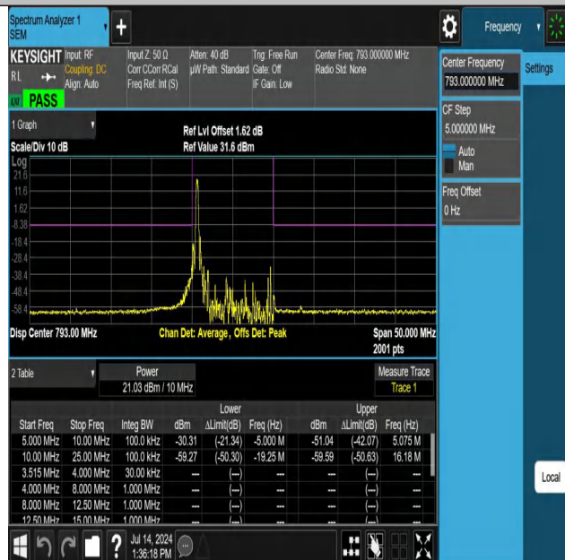
NTNV-Band14-10MHz-QPSK-23330-1RB#0--25.00--10.00-PASS
