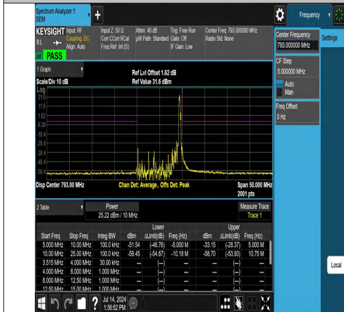
NTNV-Band14-10MHz-QPSK-23330-1RB#49--25.00--10.00-PASS
