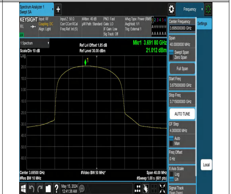
Band48-10MHz-QPSK-56690-25RB#0-PASS
