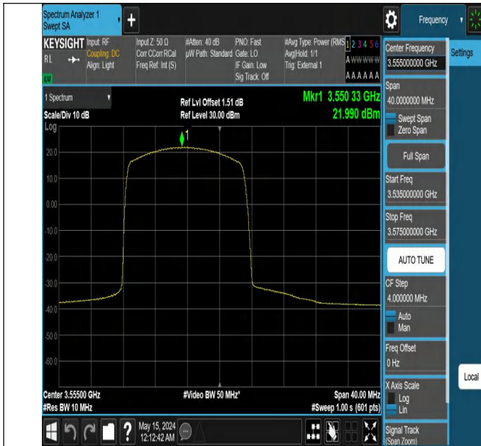
Band48-10MHz-QPSK-55290-1RB#0-PASS
