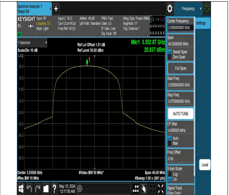
Band48-10MHz-QPSK-55290-25RB#0-PASS
