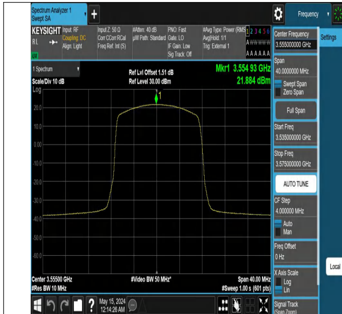
Band48-10MHz-QPSK-55290-1RB#24-PASS
