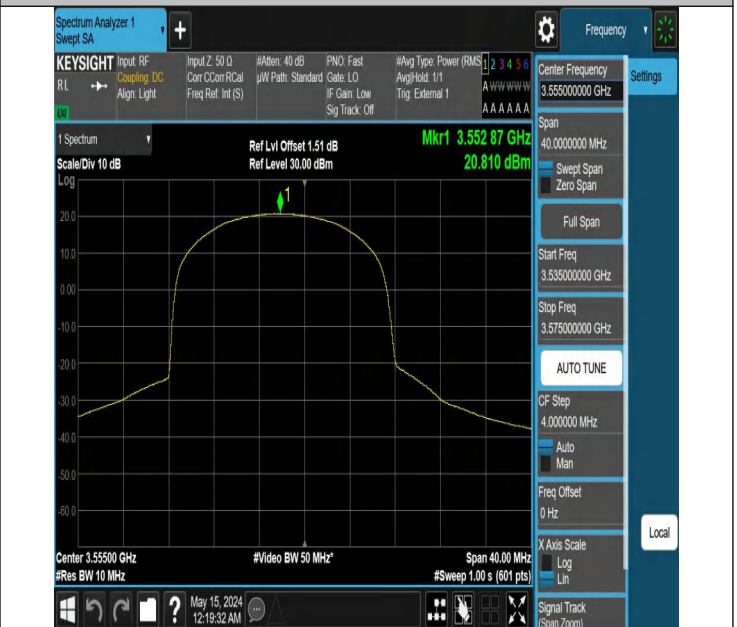
Band48-10MHz-QPSK-55290-25RB#12-PASS
