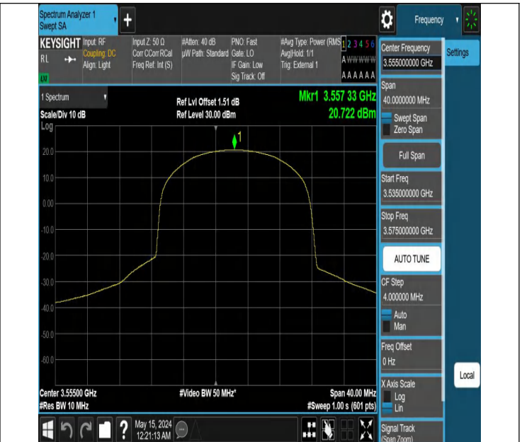
Band48-10MHz-QPSK-55290-25RB#25-PASS
