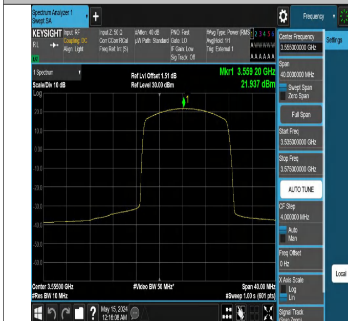
Band48-10MHz-QPSK-55290-1RB#49-PASS
