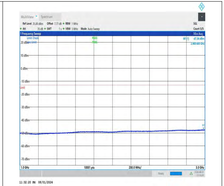
NTNV-DC_26A-n78A(3700-3800)-PC3-30-5+60-M+L-QPSK-IDLE -DFT-QPSK-Edge_1RB_Left-1000-3000-PASS
