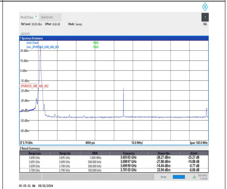
NTNV-DC_26A-n78A(3700-3800)-PC3-30-5+90-M+L-QPSK-IDLE -DFT-BPSK-Edge_1RB_Left-PASS
