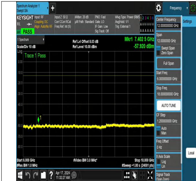
NTNV_N78-3700-3800_PC2_30_100_M_TID5_NS_01_6000_18
