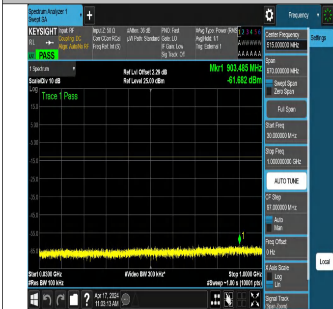
NTNV_N78-3700-3800_PC2_30_100_L_TID2_NS_01_30_1000
