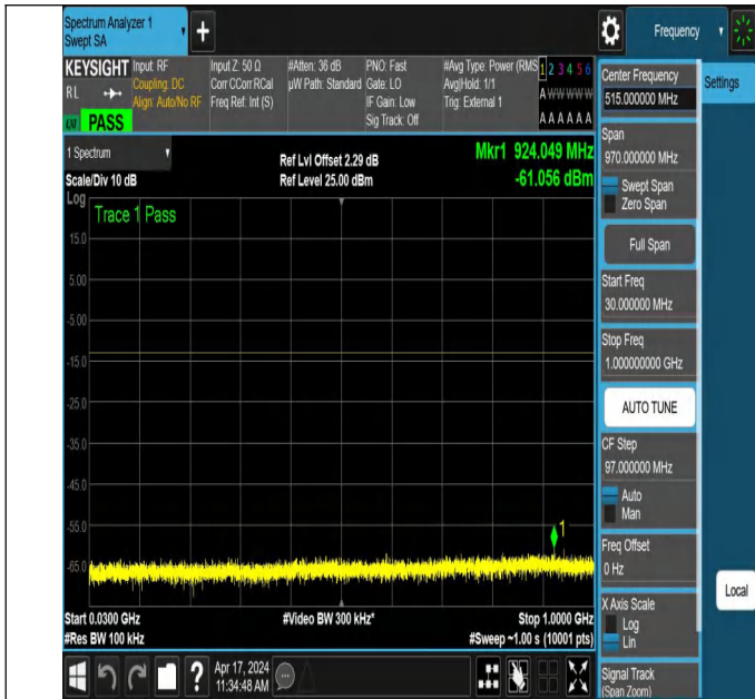
NTNV_N78-3700-3800_PC2_30_100_M_TID6_NS_01_30_1000
