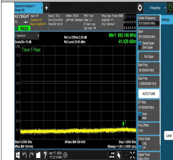
NTNV_N78-3700-3800_PC2_30_100_L_TID5_NS_01_30_1000
