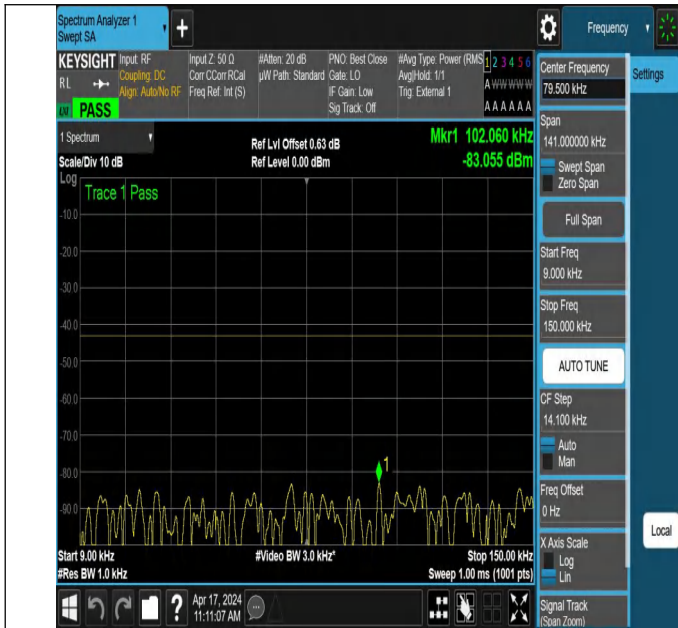
NTNV_N78-3700-3800_PC2_30_100_L_TID5_NS_01_0.009_0.
