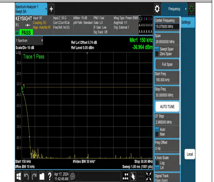
NTNV_N78-3700-3800_PC2_30_100_H_TID3_NS_01_0.15_30_#
