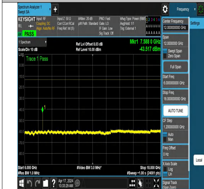
NTNV_N78-3700-3800_PC2_30_90_M_TID3_NS_01_6000_180
