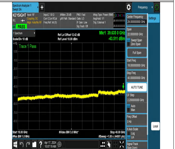
NTNV_N78-3700-3800_PC2_30_80_H_TID6_NS_01_18000_40000_#1
