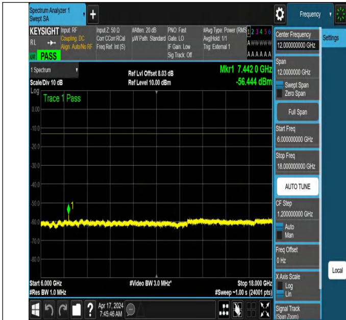
NTNV_N78-3700-3800_PC2_30_60_M_TID2_NS_01_6000_180
