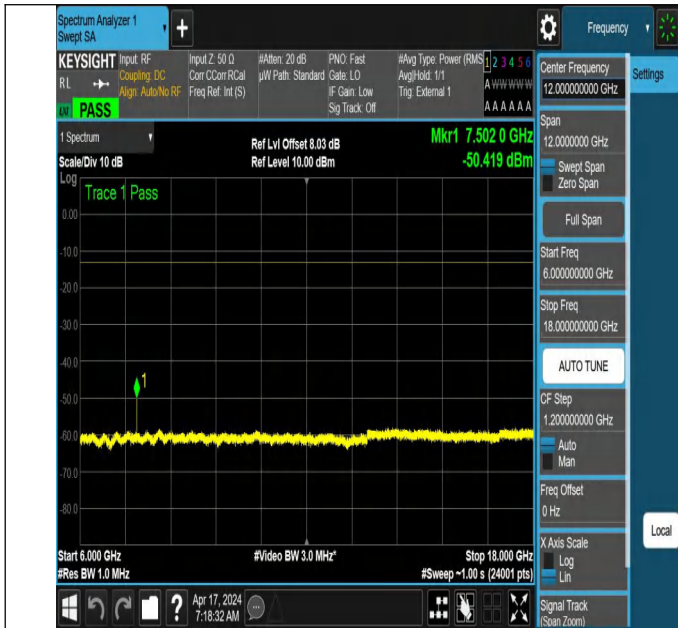
NTNV_N78-3700-3800_PC2_30_50_H_TID5_NS_01_6000_180
