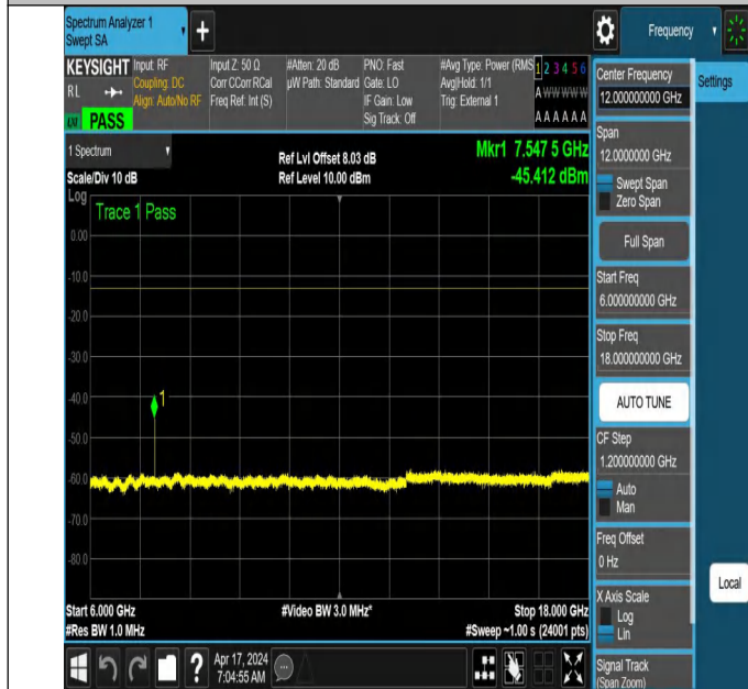
NTNV_N78-3700-3800_PC2_30_50_M_TID6_NS_01_6000_18000_#1
