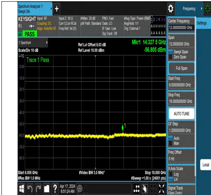
NTNV_N78-3700-3800_PC2_30_50_M_TID2_NS_01_6000_180
