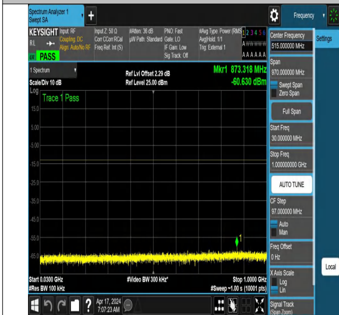
NTNV_N78-3700-3800_PC2_30_50_H_TID2_NS_01_30_1000_ #1
