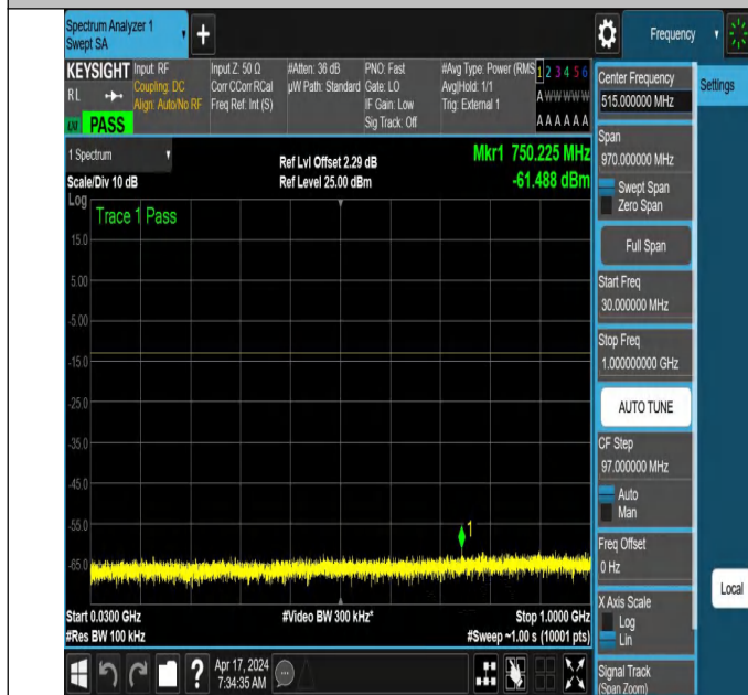
NTNV_N78-3700-3800_PC2_30_60_L_TID5_NS_01_30_1000_
