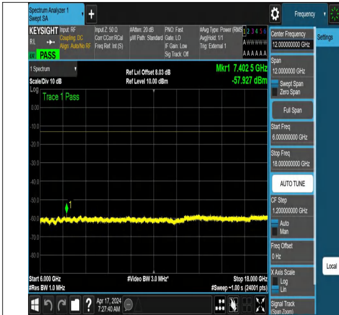
NTNV_N78-3700-3800_PC2_30_60_L_TID2_NS_01_6000_180
