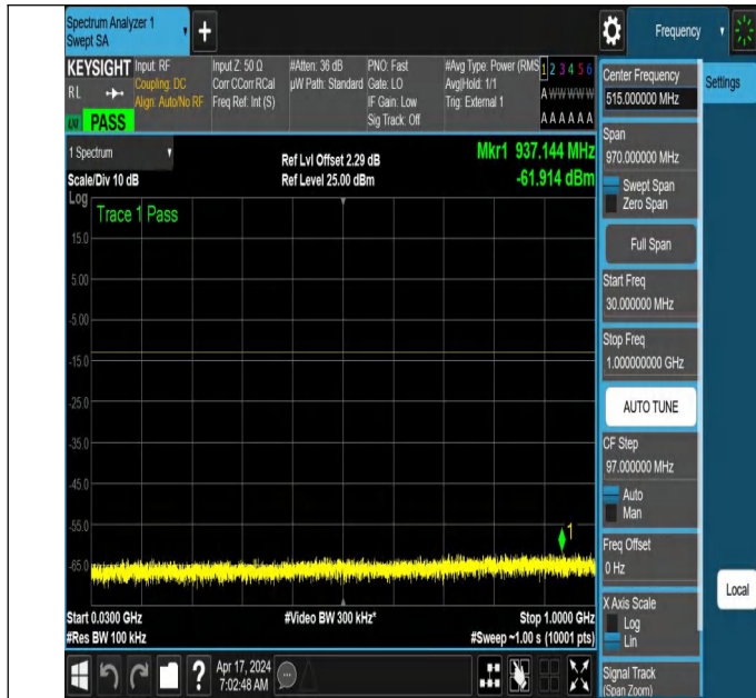
NTNV_N78-3700-3800_PC2_30_50_M_TID6_NS_01_30_1000_#1
