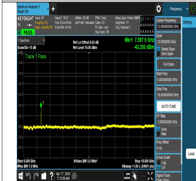
NTNV_N78-3700-3800_PC2_30_50_H_TID3_NS_01_6000_18000_#1
