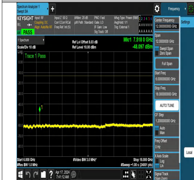
NTNV_N78-3700-3800_PC2_30_60_L_TID6_NS_01_6000_180
