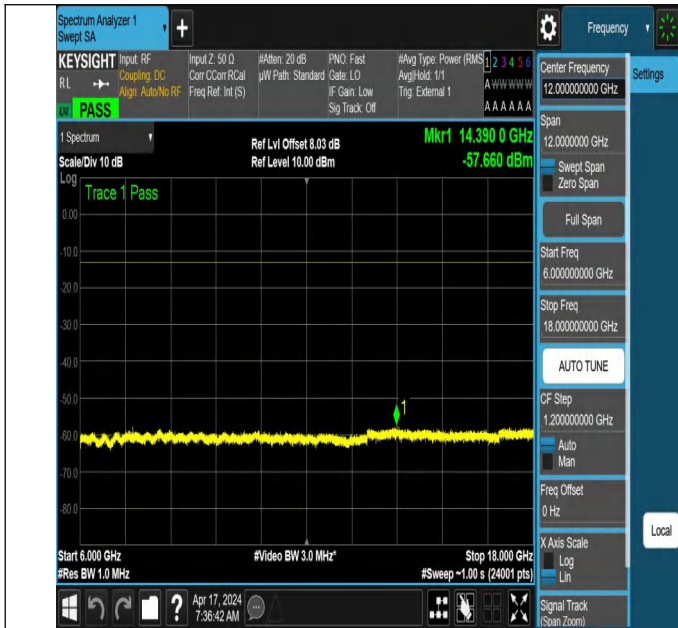
NTNV_N78-3700-3800_PC2_30_60_L_TID5_NS_01_6000_180
