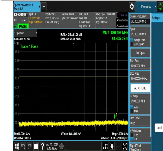
NTNV_N78-3700-3800_PC2_30_60_M_TID2_NS_01_30_1000_
