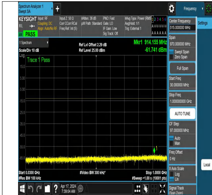
NTNV_N78-3700-3800_PC2_30_60_L_TID6_NS_01_30_1000_
