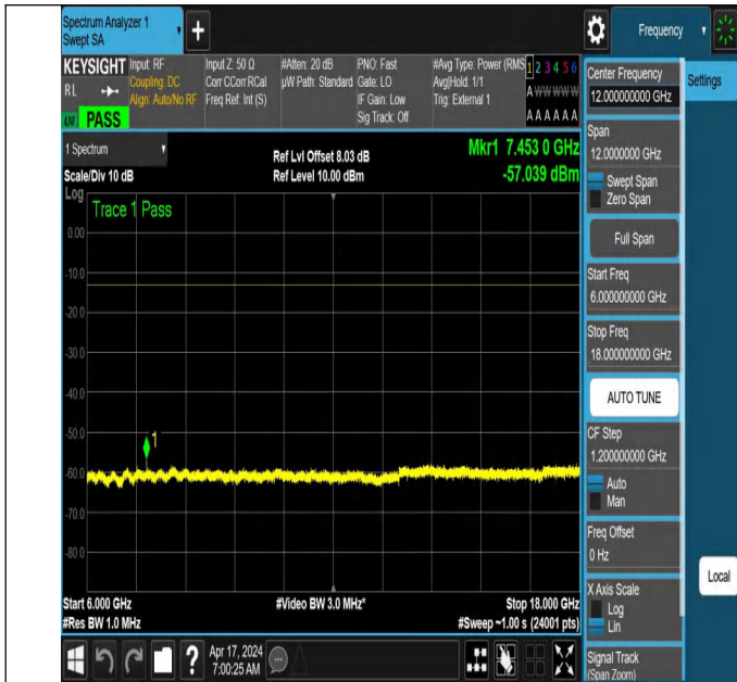
NTNV_N78-3700-3800_PC2_30_50_M_TID5_NS_01_6000_180
