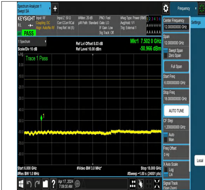
NTNV_N78-3700-3800_PC2_30_50_H_TID2_NS_01_6000_18000_#1
