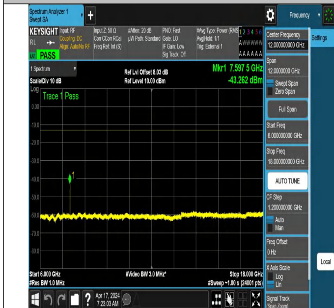
NTNV_N78-3700-3800_PC2_30_50_H_TID6_NS_01_6000_18000_#1
