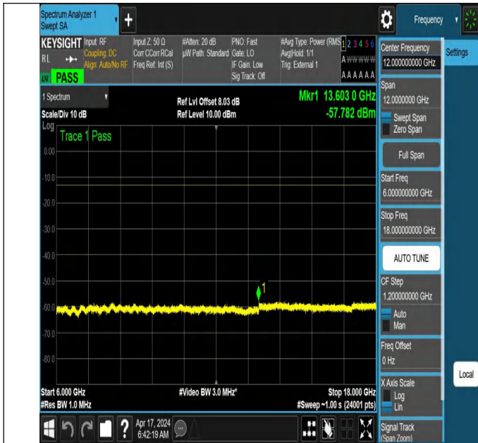
NTNV_N78-3700-3800_PC2_30_50_L_TID5_NS_01_6000_180
