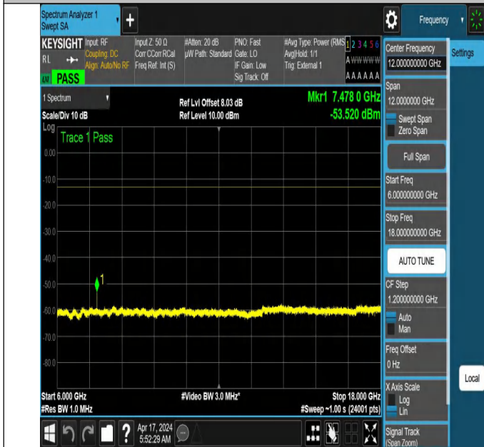
NTNV_N78-3700-3800_PC2_30_40_L_TID6_NS_01_6000_18000_#1
