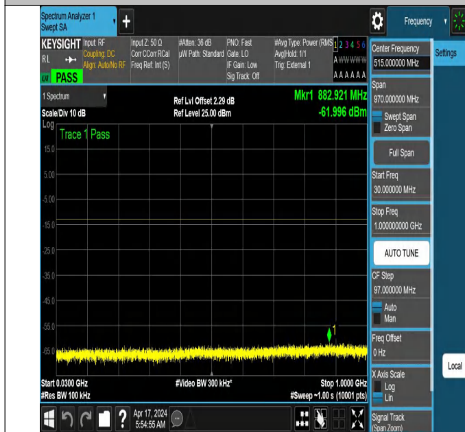
NTNV_N78-3700-3800_PC2_30_40_M_TID2_NS_01_30_1000_
