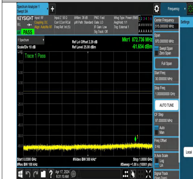
NTNV_N78-3700-3800_PC2_30_50_L_TID2_NS_01_30_1000_#1
