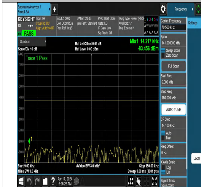
NTNV_N78-3700-3800_PC2_30_40_H_TID6_NS_01_0.009_0.15_#1
