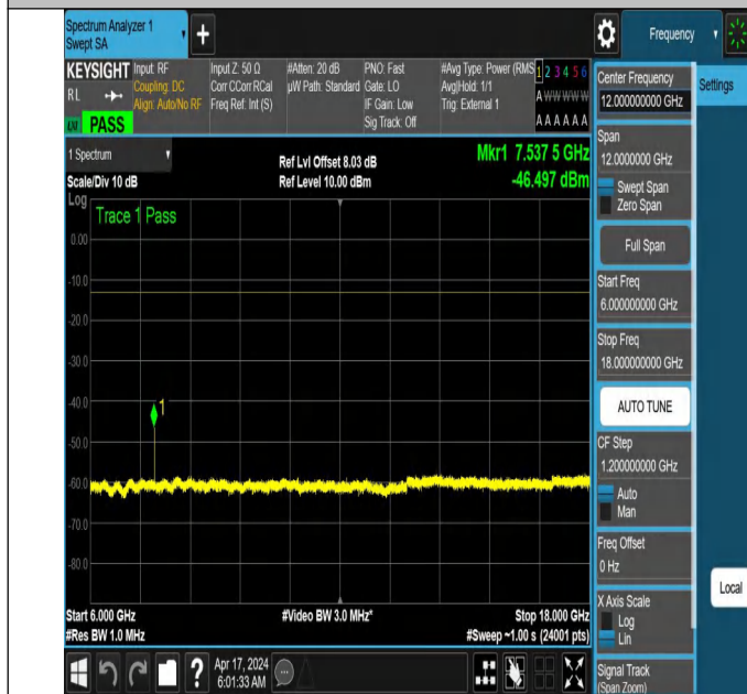
NTNV_N78-3700-3800_PC2_30_40_M_TID3_NS_01_6000_18000_#1
