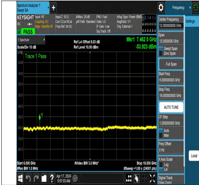
NTNV_N78-3700-3800_PC2_30_40_M_TID2_NS_01_6000_180
