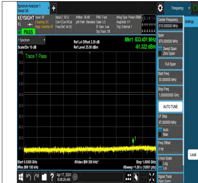
NTNV_N78-3700-3800_PC2_30_40_M_TID6_NS_01_30_1000_#1
