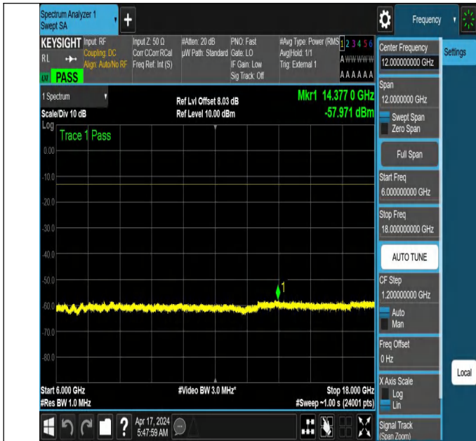
NTNV_N78-3700-3800_PC2_30_40_L_TID5_NS_01_6000_180
