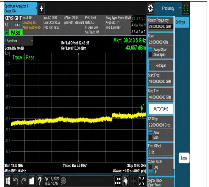
NTNV_N78-3700-3800_PC2_30_40_M_TID5_NS_01_18000_400
