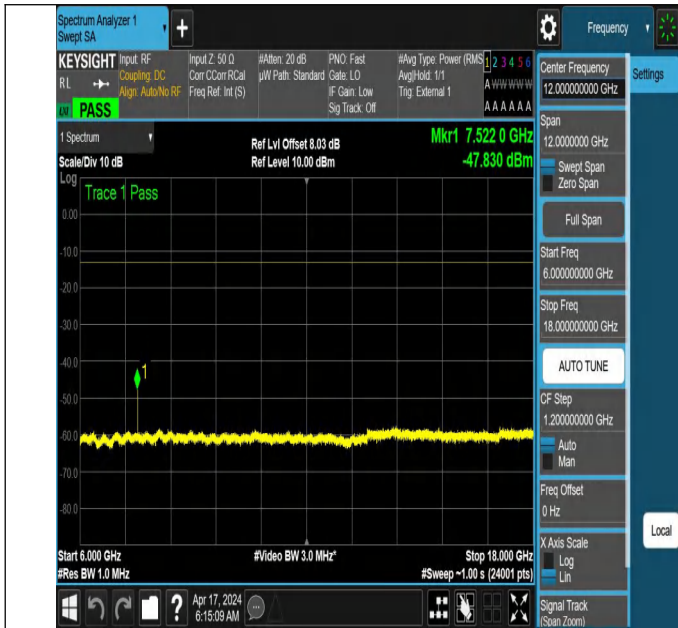
NTNV_N78-3700-3800_PC2_30_40_H_TID2_NS_01_6000_180
