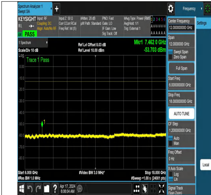
NTNV_N78-3700-3800_PC2_30_40_M_TID5_NS_01_6000_180
