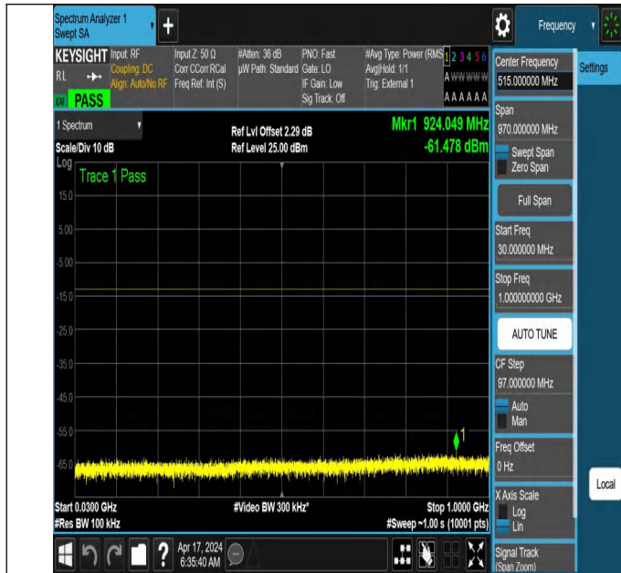
NTNV_N78-3700-3800_PC2_30_50_L_TID3_NS_01_30_1000_
