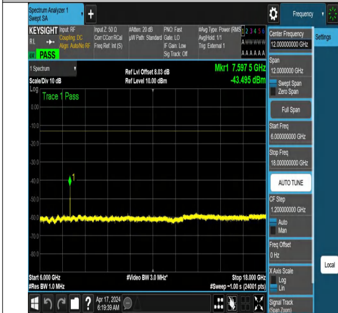
NTNV_N78-3700-3800_PC2_30_40_H_TID3_NS_01_6000_18000_#1
