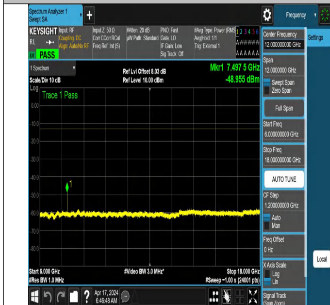
NTNV_N78-3700-3800_PC2_30_50_L_TID6_NS_01_6000_180
