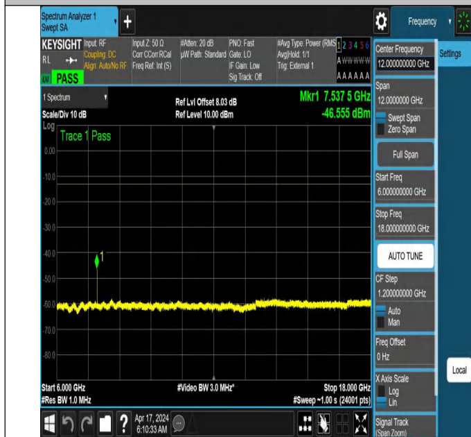
NTNV_N78-3700-3800_PC2_30_40_M_TID6_NS_01_6000_18000_#1
