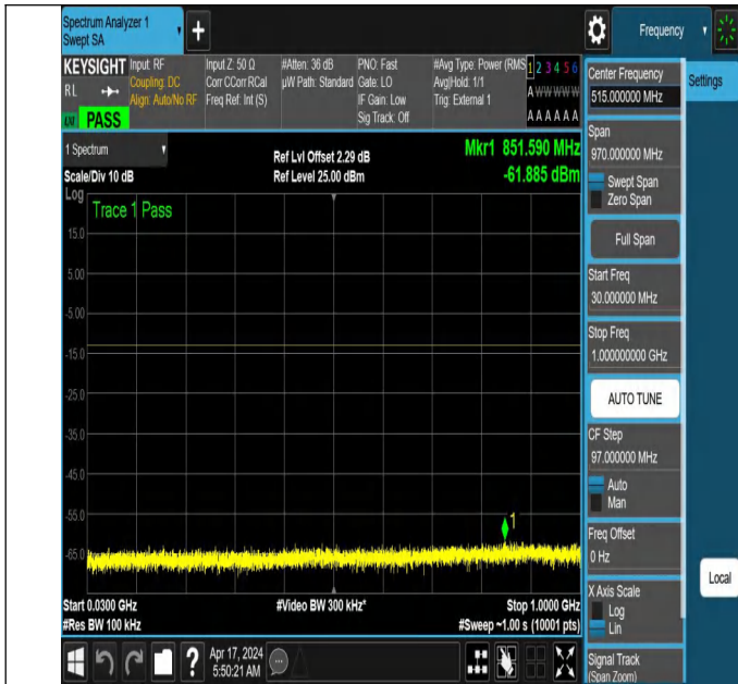
NTNV_N78-3700-3800_PC2_30_40_L_TID6_NS_01_30_1000_#1
