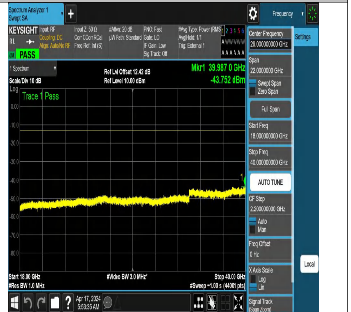
NTNV_N78-3700-3800_PC2_30_40_L_TID6_NS_01_18000_40000_#1
