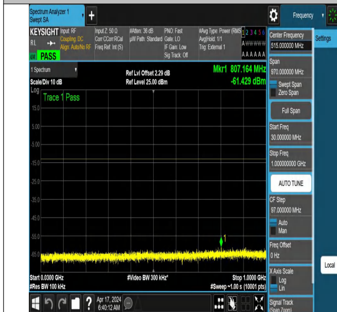
NTNV_N78-3700-3800_PC2_30_50_L_TID5_NS_01_30_1000_ #1
