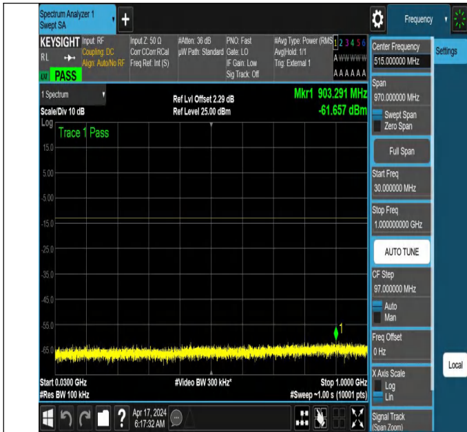
NTNV_N78-3700-3800_PC2_30_40_H_TID3_NS_01_30_1000_#1
