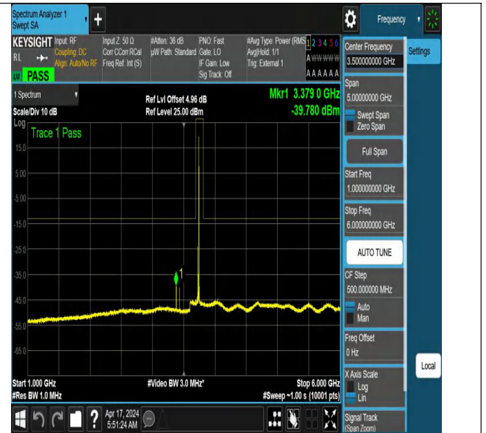
NTNV_N78-3700-3800_PC2_30_40_L_TID6_NS_01_1000_6000_#1
