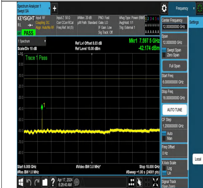
NTNV_N78-3700-3800_PC2_30_40_H_TID6_NS_01_6000_18000_#1
