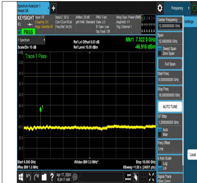
NTNV_N78-3700-3800_PC2_30_40_H_TID5_NS_01_6000_18000_#1
