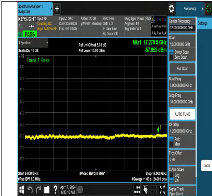
NTNV_N78-3700-3800_PC2_30_50_L_TID2_NS_01_6000_180
