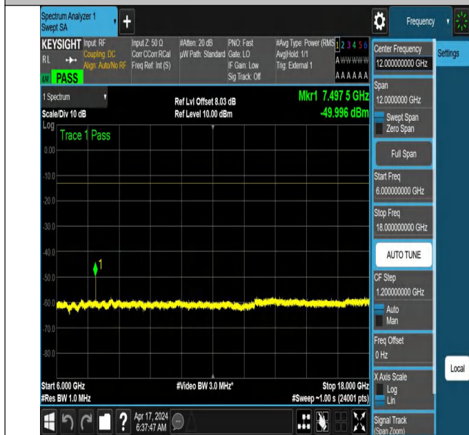
NTNV_N78-3700-3800_PC2_30_50_L_TID3_NS_01_6000_180
