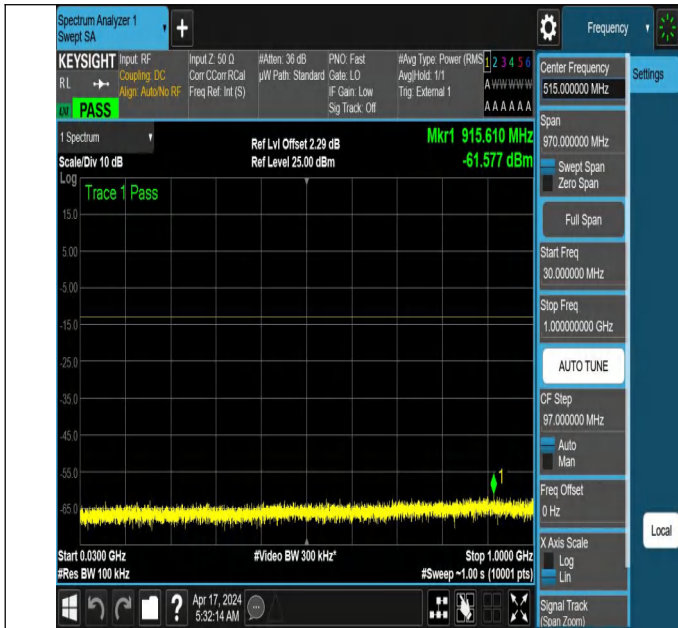
NTNV_N78-3700-3800_PC2_30_30_H_TID6_NS_01_30_1000_
