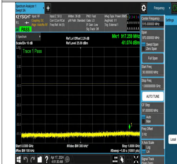
NTNV_N78-3700-3800_PC2_30_30_L_TID5_NS_01_30_1000_ #1
