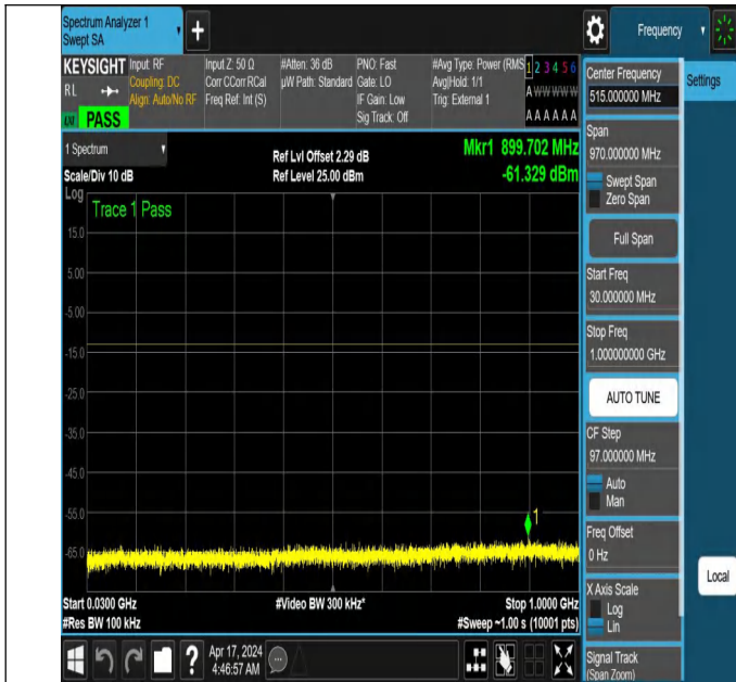
NTNV_N78-3700-3800_PC2_30_30_L_TID3_NS_01_30_1000_
