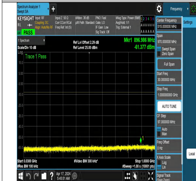
NTNV_N78-3700-3800_PC2_30_40_L_TID5_NS_01_30_1000_ #1
