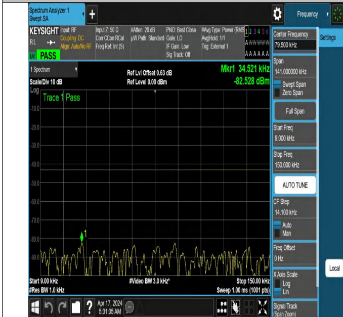
NTNV_N78-3700-3800_PC2_30_30_H_TID6_NS_01_0.009_0.15_#1
