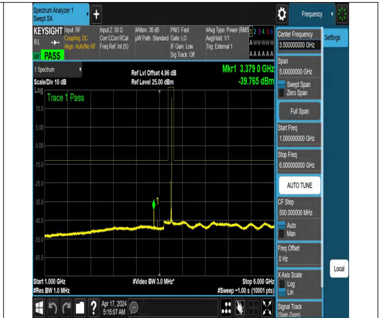
NTNV_N78-3700-3800_PC2_30_30_M_TID6_NS_01_1000_6000_#1
