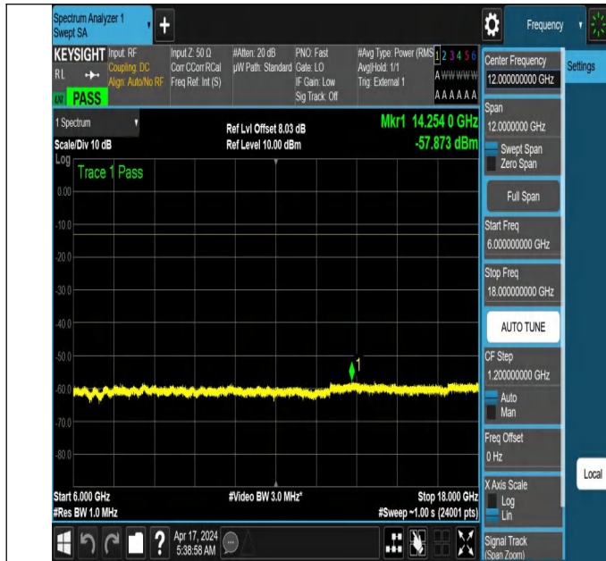
NTNV_N78-3700-3800_PC2_30_40_L_TID2_NS_01_6000_180
