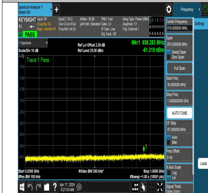
NTNV_N78-3700-3800_PC2_30_30_H_TID5_NS_01_30_1000_ #1
