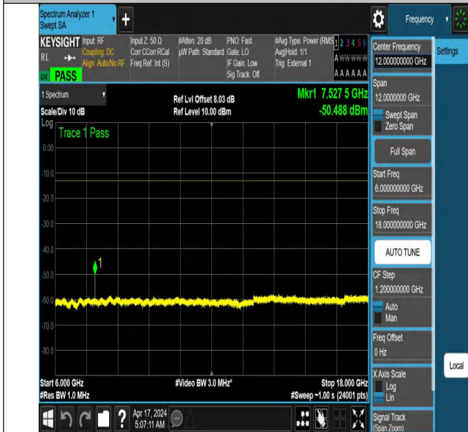
NTNV_N78-3700-3800_PC2_30_30_M_TID3_NS_01_6000_18000_#1
