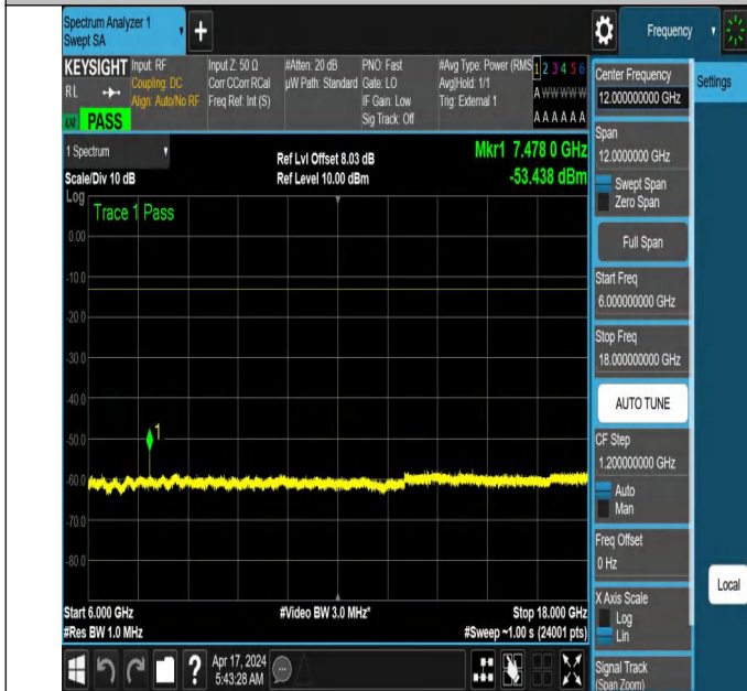
NTNV_N78-3700-3800_PC2_30_40_L_TID3_NS_01_6000_18000_#1
