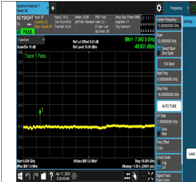
NTNV_N78-3700-3800_PC2_30_30_H_TID2_NS_01_6000_18000_#1
