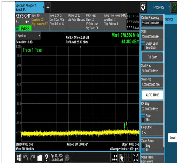
NTNV_N78-3700-3800_PC2_30_30_L_TID6_NS_01_30_1000_#1
