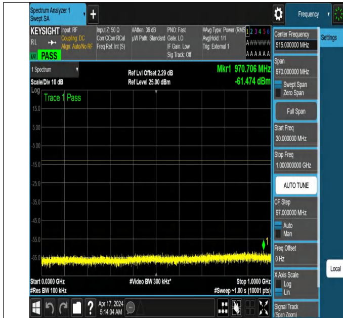
NTNV_N78-3700-3800_PC2_30_30_M_TID6_NS_01_30_1000_#1
