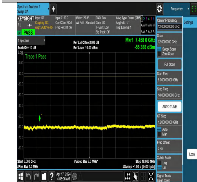
NTNV_N78-3700-3800_PC2_30_30_L_TID6_NS_01_6000_18000_#1
