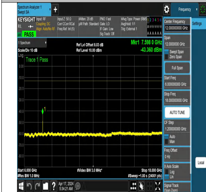
NTNV_N78-3700-3800_PC2_30_30_H_TID6_NS_01_6000_180
