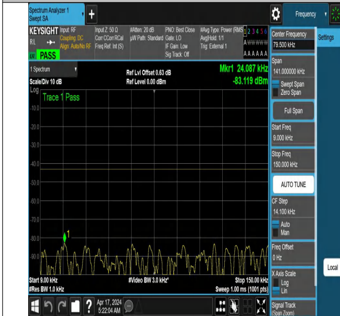
NTNV_N78-3700-3800_PC2_30_30_H_TID3_NS_01_0.009_0.15_#1
