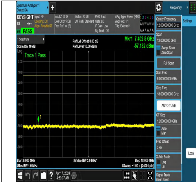
NTNV_N78-3700-3800_PC2_30_30_L_TID5_NS_01_6000_180
