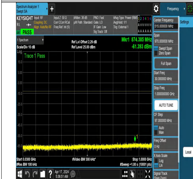
NTNV_N78-3700-3800_PC2_30_40_L_TID2_NS_01_30_1000_#1
