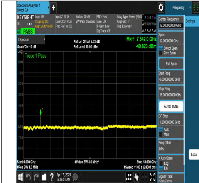
NTNV_N78-3700-3800_PC2_30_30_H_TID5_NS_01_6000_18000_#1
