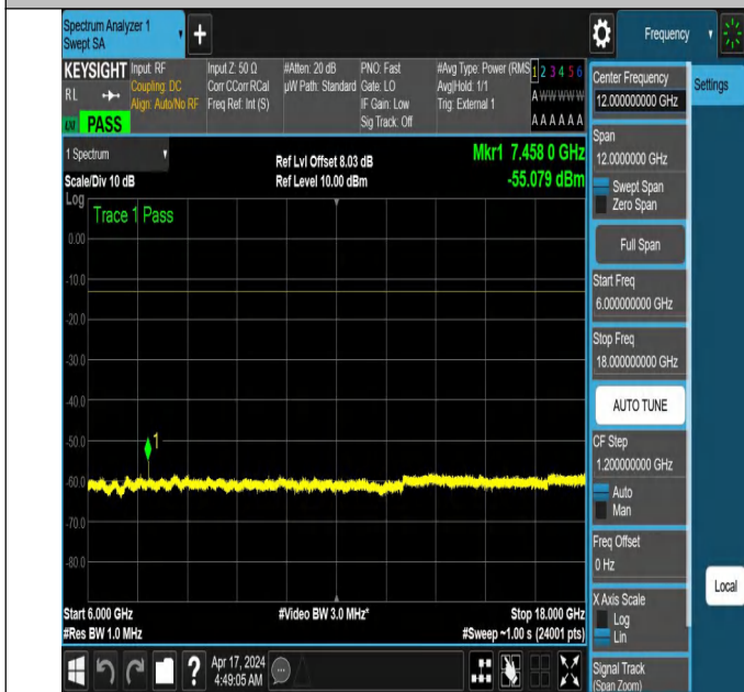
NTNV_N78-3700-3800_PC2_30_30_L_TID3_NS_01_6000_180
