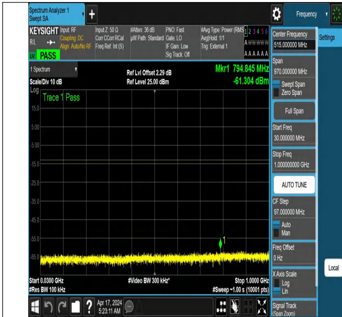
NTNV_N78-3700-3800_PC2_30_30_H_TID3_NS_01_30_1000_
