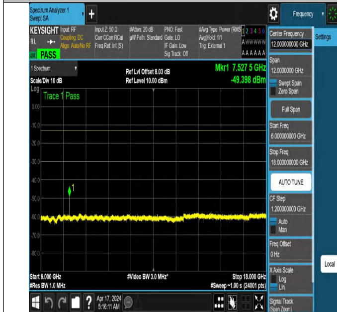
NTNV_N78-3700-3800_PC2_30_30_M_TID6_NS_01_6000_18000_#1
