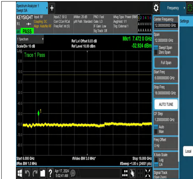
NTNV_N78-3700-3800_PC2_30_30_M_TID2_NS_01_6000_180
