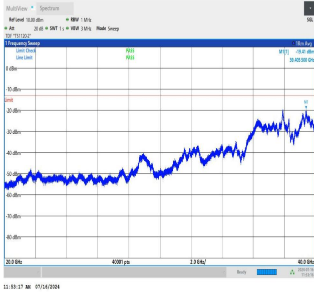
NTNV_N78-3450-3550_PC2_30_90_H_TID2_NS_01_20000_400_00_#1
