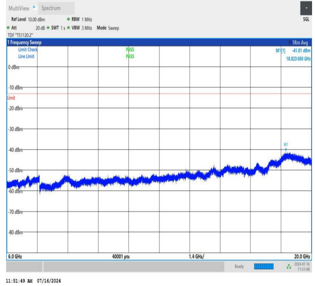
NTNV_N78-3450-3550_PC2_30_90_M_TID2_NS_01_6000_2000
