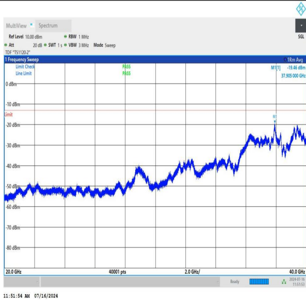
NTNV_N78-3450-3550_PC2_30_90_M_TID2_NS_01_20000_400
