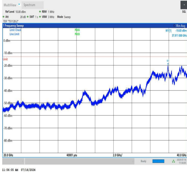
NTNV_N78-3450-3550_PC2_30_100_M_TID2_NS_01_20000_40000_#1
