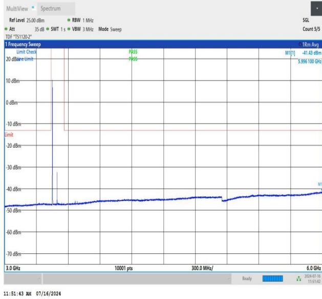
NTNV_N78-3450-3550_PC2_30_90_M_TID2_NS_01_3000_6000
