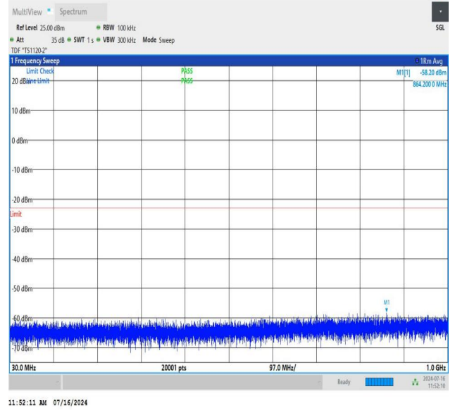
NTNV_N78-3450-3550_PC2_30_90_M_TID3_NS_01_30_1000_#
