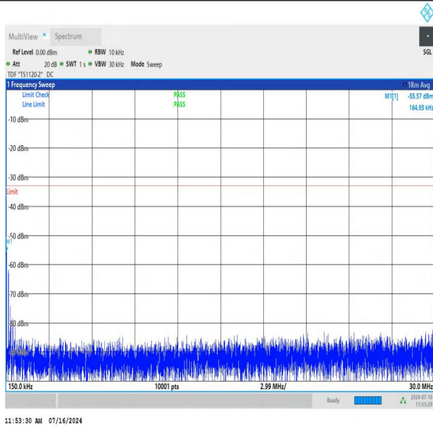
NTNV_N78-3450-3550_PC2_30_90_H_TID2_NS_01_20000_400_00_#1
