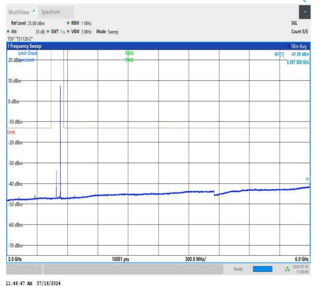
NTNV_N78-3450-3550_PC2_30_80_L_TID3_NS_01_3000_6000_#1
