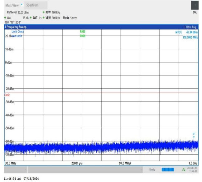
NTNV_N78-3450-3550_PC2_30_80_L_TID3_NS_01_30_1000_#1
