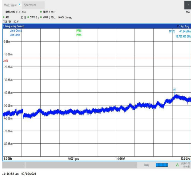
NTNV_N78-3450-3550_PC2_30_80_L_TID3_NS_01_6000_20000
