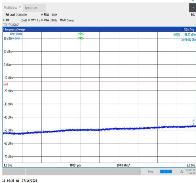
NTNV_N78-3450-3550_PC2_30_80_L_TID3_NS_01_1000_3000_#1
