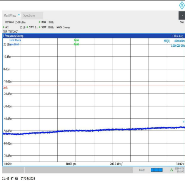
NTNV_N78-3450-3550_PC2_30_70_M_TID3_NS_01_1000_3000_#1
