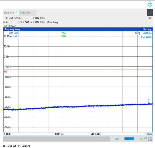
NTNV_N78-3450-3550_PC2_30_80_L_TID2_NS_01_1000_3000_#1
