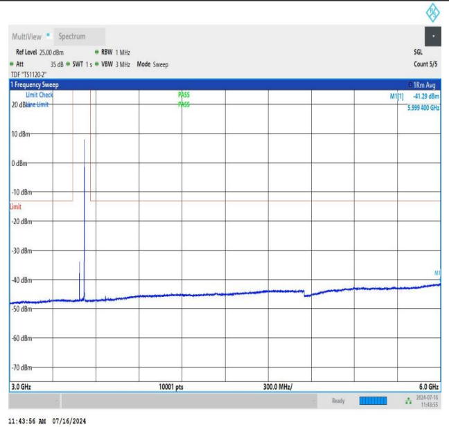
NTNV_N78-3450-3550_PC2_30_70_M_TID3_NS_01_3000_6000_#1
