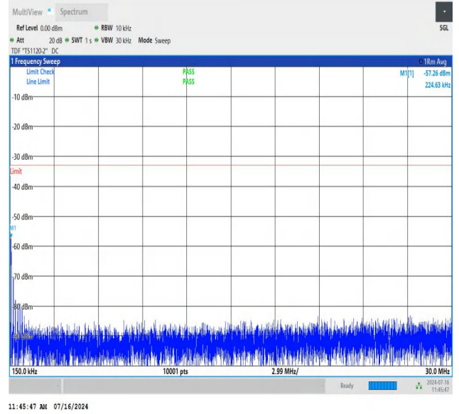
NTNV_N78-3450-3550_PC2_30_80_L_TID2_NS_01_0.15_30_#1
