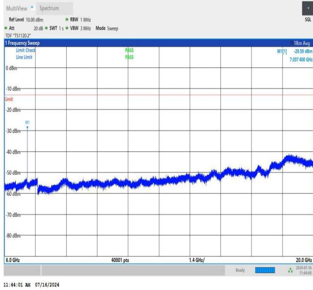
NTNV_N78-3450-3550_PC2_30_70_M_TID3_NS_01_6000_2000_0_#1
