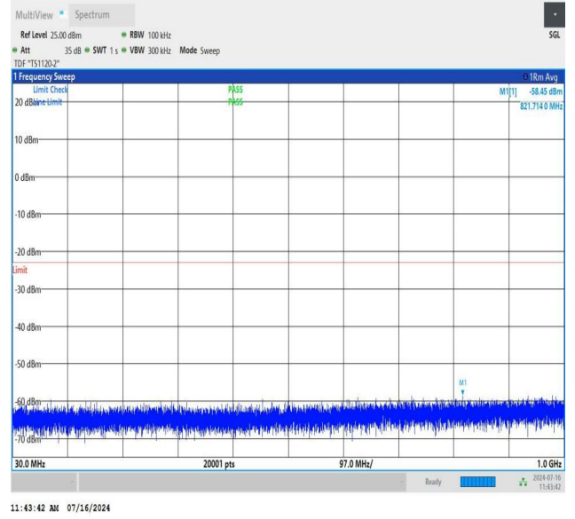
NTNV_N78-3450-3550_PC2_30_70_M_TID3_NS_01_30_1000_#
