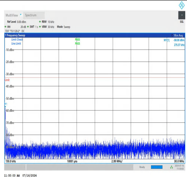
NTNV_N78-3450-3550_PC2_30_90_L_TID2_NS_01_0.15_30_#1
