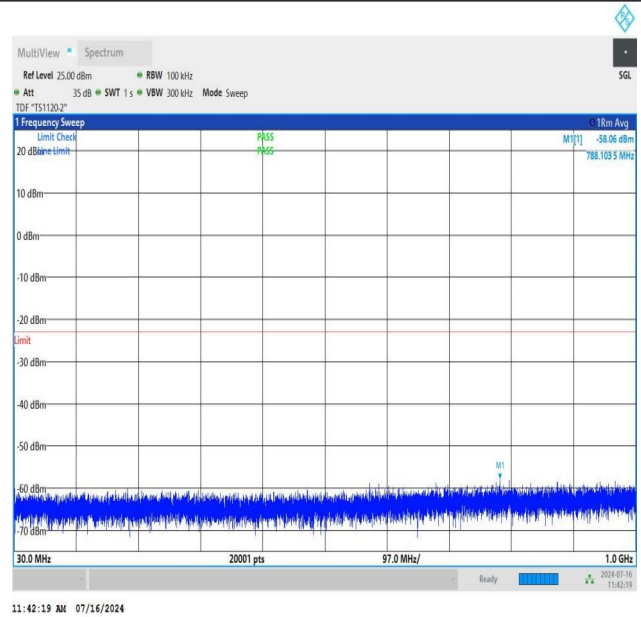
NTNV_N78-3450-3550_PC2_30_70_L_TID3_NS_01_30_1000_#1
