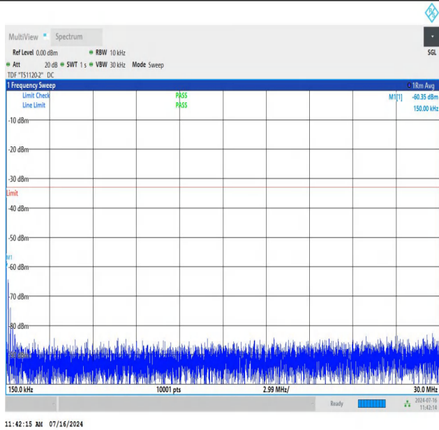
NTNV_N78-3450-3550_PC2_30_70_L_TID3_NS_01_0.15_30_#1
