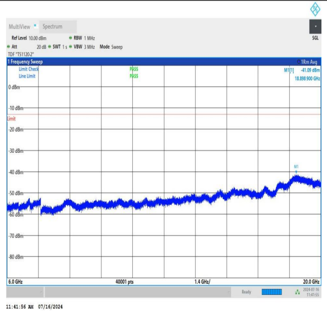
NTNV_N78-3450-3550_PC2_30_70_L_TID2_NS_01_6000_20000_#1
