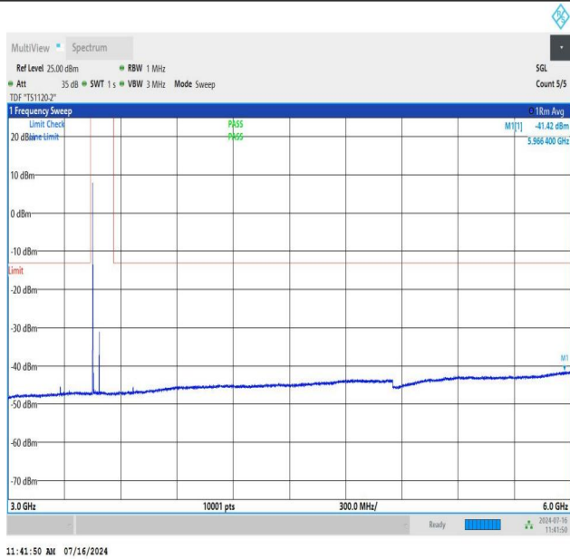
NTNV_N78-3450-3550_PC2_30_70_L_TID2_NS_01_3000_6000_#1
