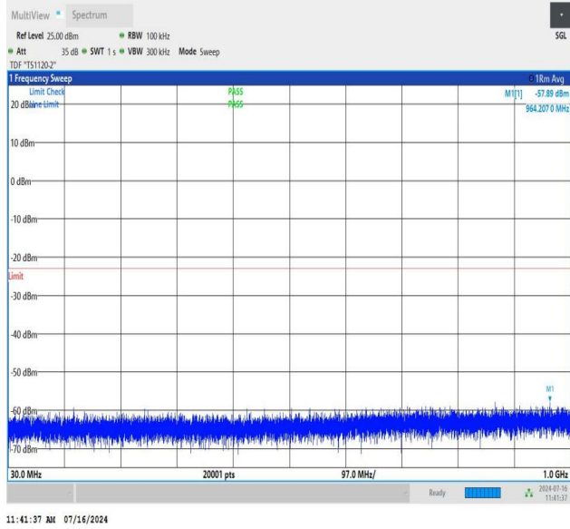
NTNV_N78-3450-3550_PC2_30_70_L_TID2_NS_01_30_1000_#1
