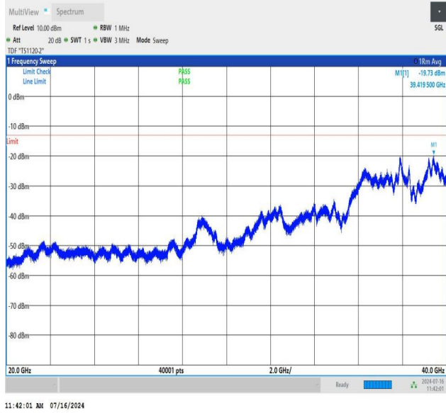
NTNV_N78-3450-3550_PC2_30_70_L_TID2_NS_01_20000_4000_0_#1
