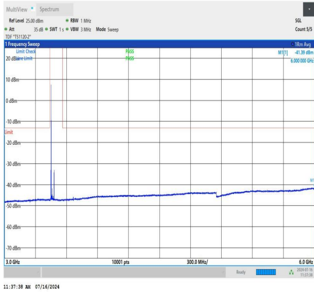
NTNV_N78-3450-3550_PC2_30_60_L_TID2_NS_01_3000_6000_#1
