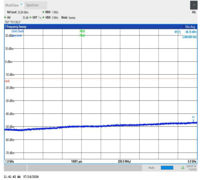
NTNV_N78-3450-3550_PC2_30_70_L_TID2_NS_01_1000_3000_#1
