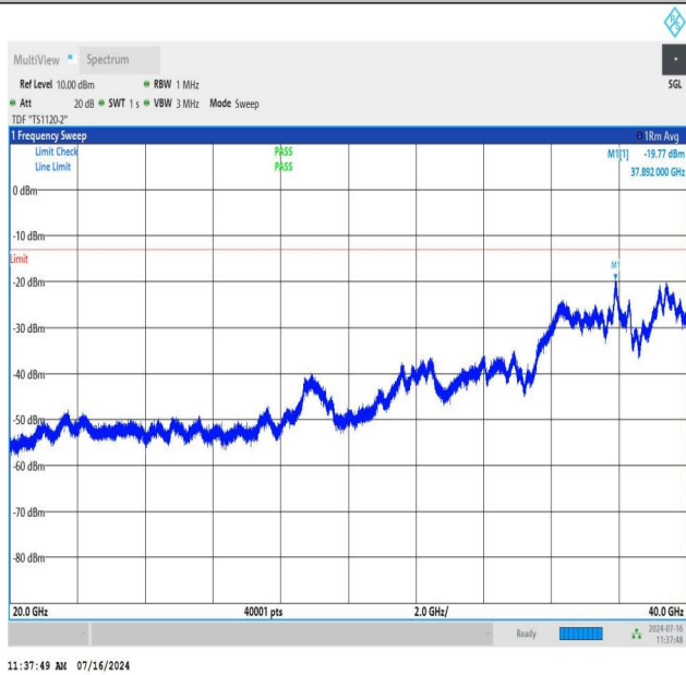
NTNV_N78-3450-3550_PC2_30_60_L_TID2_NS_01_20000_4000_0_#1
