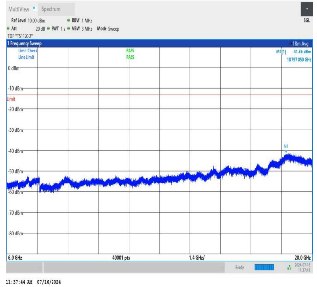
NTNV_N78-3450-3550_PC2_30_60_L_TID2_NS_01_6000_20000_#1
