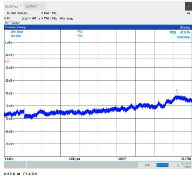
NTNV_N78-3450-3550_PC2_30_80_M_TID2_NS_01_6000_2000
