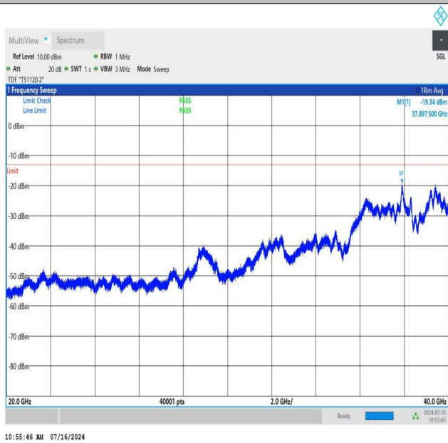
NTNV_N78-3450-3550_PC2_30_80_M_TID2_NS_01_20000_400
