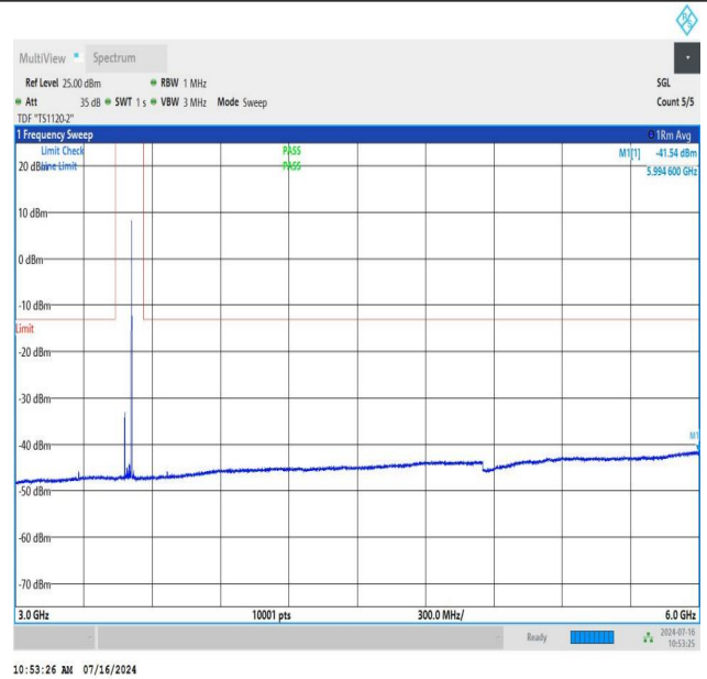
NTNV_N78-3450-3550_PC2_30_60_H_TID3_NS_01_3000_6000_#1
