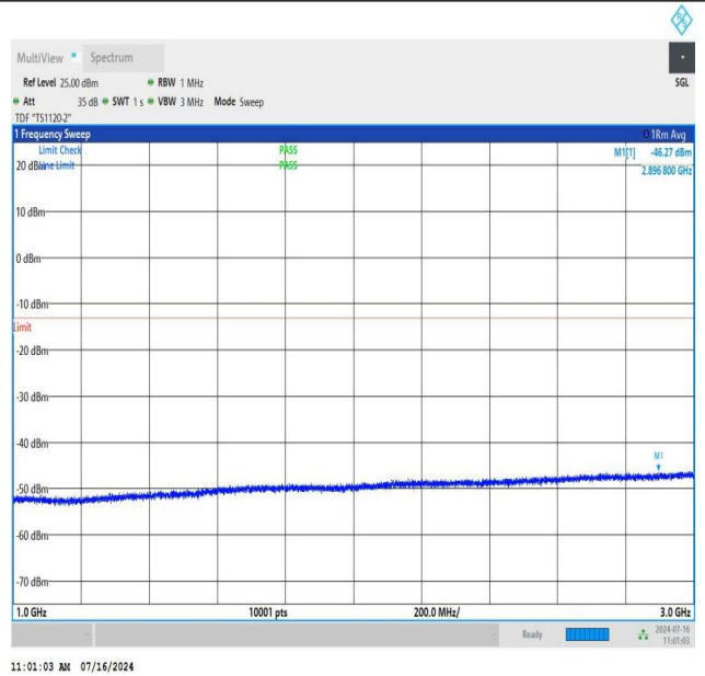
NTNV_N78-3450-3550_PC2_30_90_H_TID2_NS_01_1000_3000_#1
