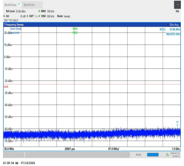
NTNV_N78-3450-3550_PC2_30_90_L_TID3_NS_01_30_1000_#1
