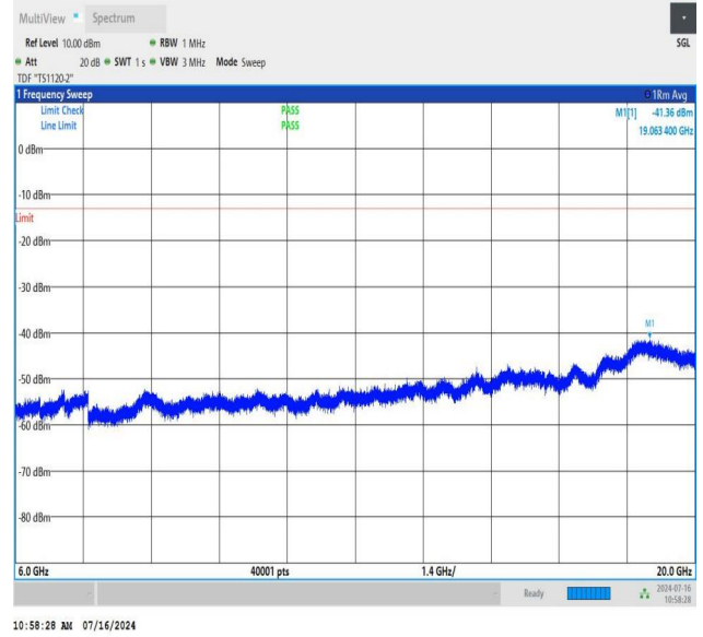
NTNV_N78-3450-3550_PC2_30_90_L_TID2_NS_01_6000_20000_
