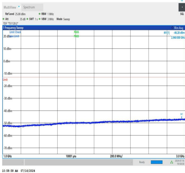
NTNV_N78-3450-3550_PC2_30_90_L_TID3_NS_01_1000_3000_#1
