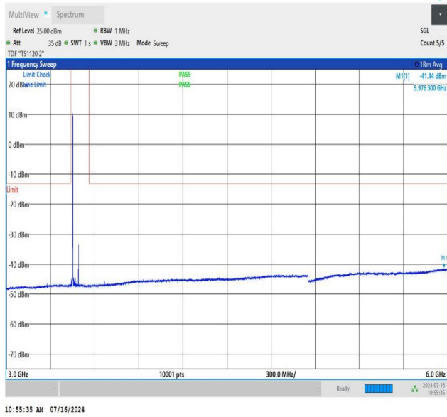
NTNV_N78-3450-3550_PC2_30_80_M_TID2_NS_01_3000_6000
