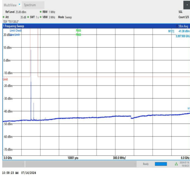
NTNV_N78-3450-3550_PC2_30_90_L_TID2_NS_01_3000_6000_
