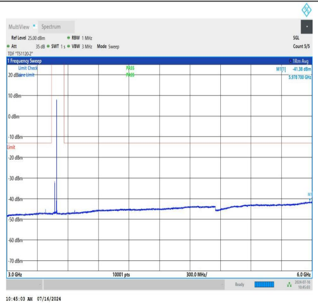
NTNV_N78-3450-3550_PC2_30_40_H_TID3_NS_01_3000_6000_#1
