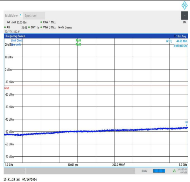
NTNV_N78-3450-3550_PC2_30_40_L_TID2_NS_01_1000_3000_#1
