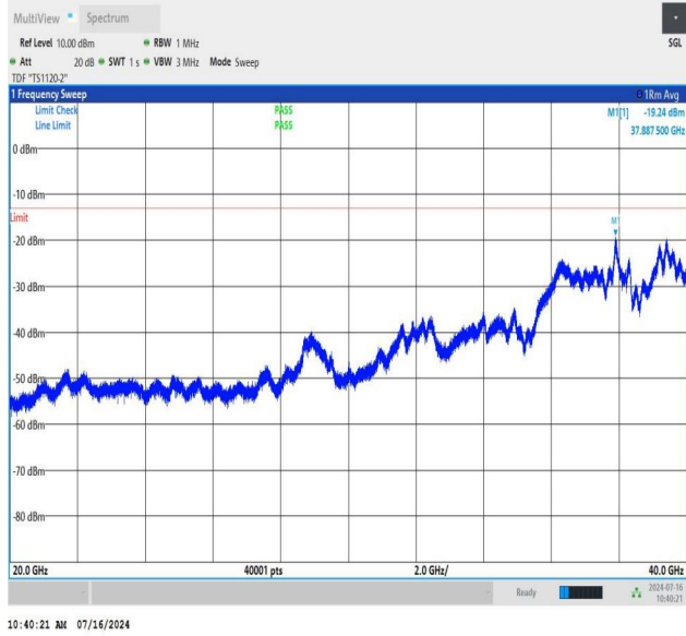
NTNV_N78-3450-3550_PC2_30_30_H_TID2_NS_01_20000_400 00_#1
