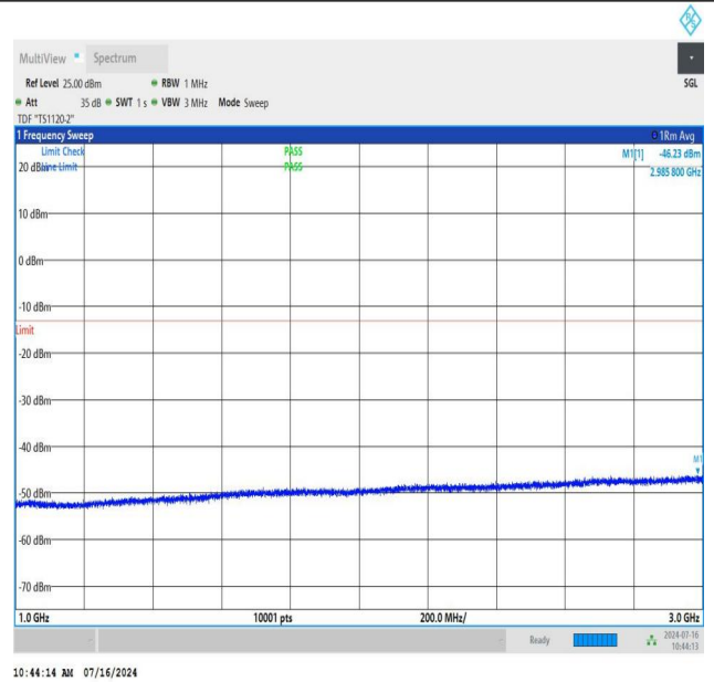
NTNV_N78-3450-3550_PC2_30_40_H_TID2_NS_01_1000_3000_#1
