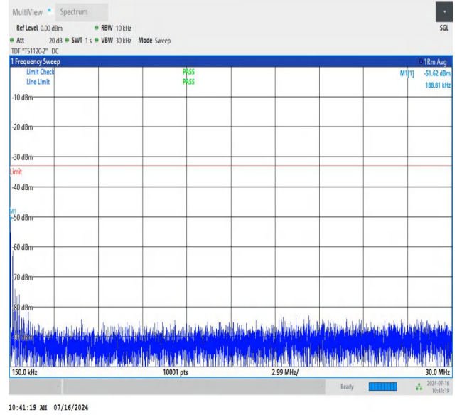
NTNV_N78-3450-3550_PC2_30_40_L_TID2_NS_01_0.15_30_#1
