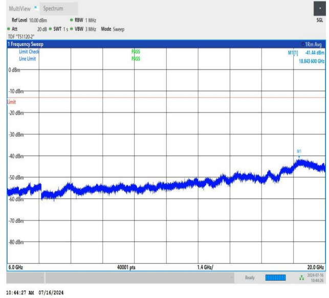
NTNV_N78-3450-3550_PC2_30_40_H_TID2_NS_01_6000_2000_0_#1
