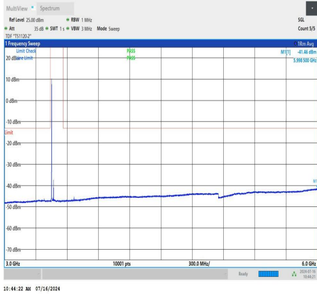
NTNV_N78-3450-3550_PC2_30_40_H_TID2_NS_01_3000_6000_#1
