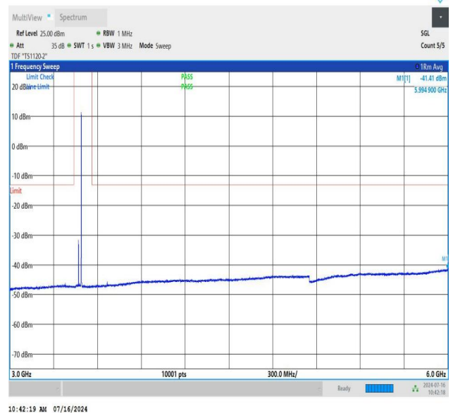
NTNV_N78-3450-3550_PC2_30_40_L_TID3_NS_01_3000_6000_#1
