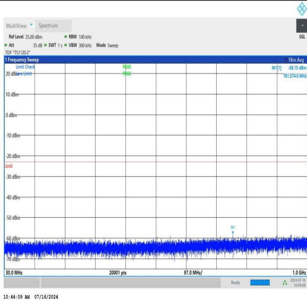
NTNV_N78-3450-3550_PC2_30_40_H_TID2_NS_01_30_1000_#1
