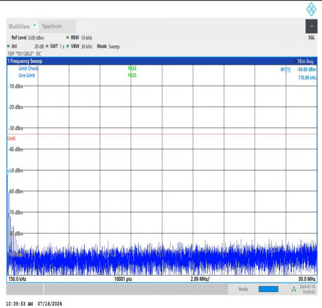
NTNV_N78-3450-3550_PC2_30_30_H_TID2_NS_01_0.15_30_#1
