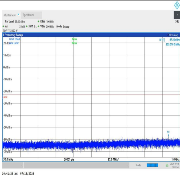
NTNV_N78-3450-3550_PC2_30_40_L_TID2_NS_01_30_1000_#1
