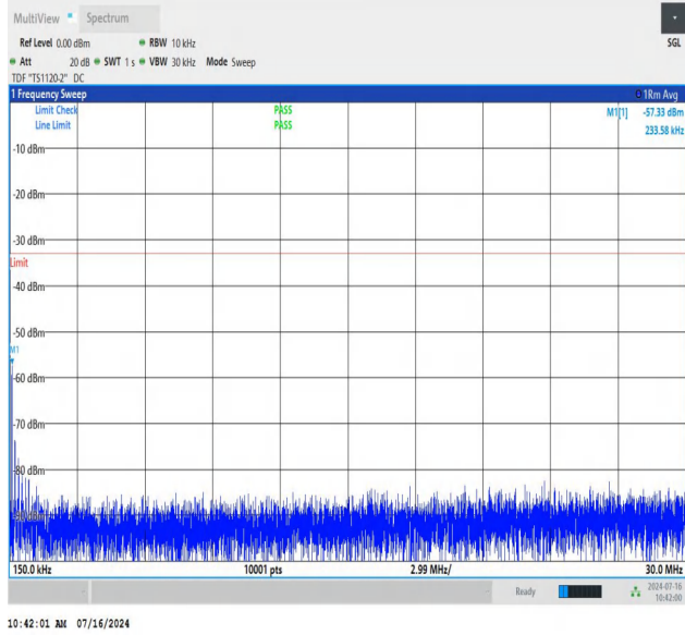
NTNV_N78-3450-3550_PC2_30_40_L_TID3_NS_01_0.15_30_#1
