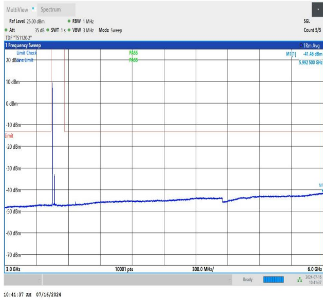
NTNV_N78-3450-3550_PC2_30_40_L_TID2_NS_01_3000_6000_
