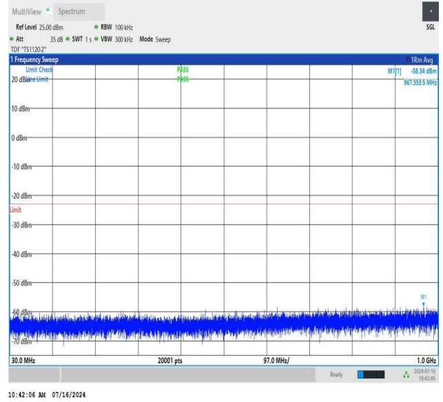
NTNV_N78-3450-3550_PC2_30_40_L_TID3_NS_01_30_1000_#1
