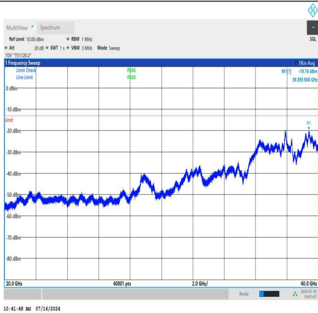
NTNV_N78-3450-3550_PC2_30_40_L_TID2_NS_01_20000_4000_
