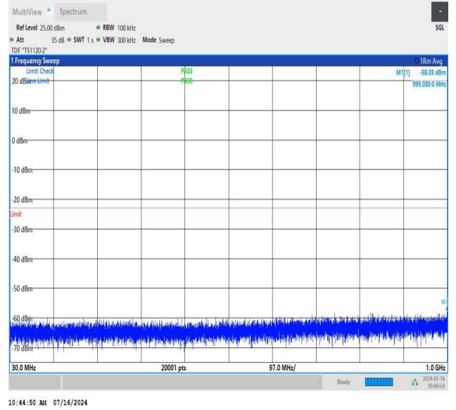
NTNV_N78-3450-3550_PC2_30_40_H_TID3_NS_01_30_1000_# 1
