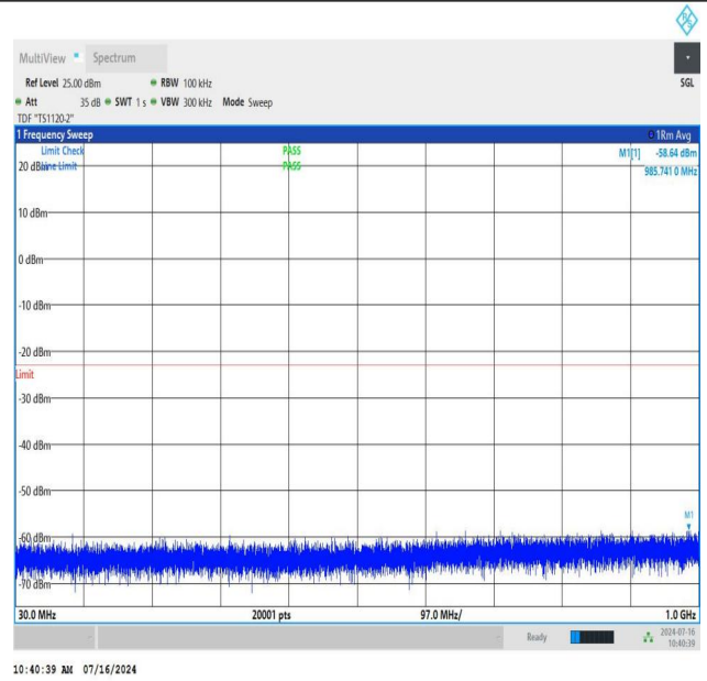
NTNV_N78-3450-3550_PC2_30_30_H_TID3_NS_01_30_1000_# 1
