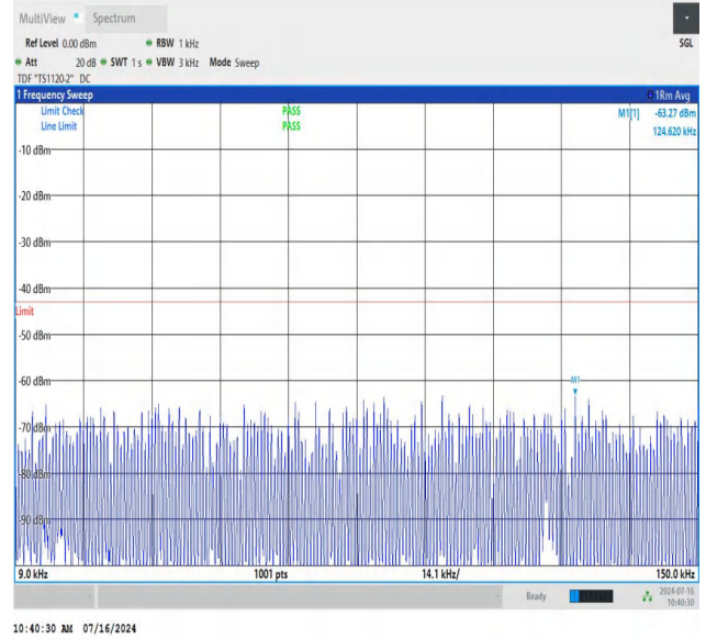
NTNV_N78-3450-3550_PC2_30_30_H_TID3_NS_01_0.009_0.15 _#1
