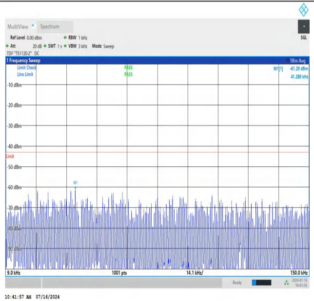
NTNV_N78-3450-3550_PC2_30_40_L_TID3_NS_01_0.009_0.15_
