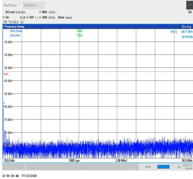
NTNV_N78-3450-3550_PC2_30_40_H_TID3_NS_01_0.15_30_#1
