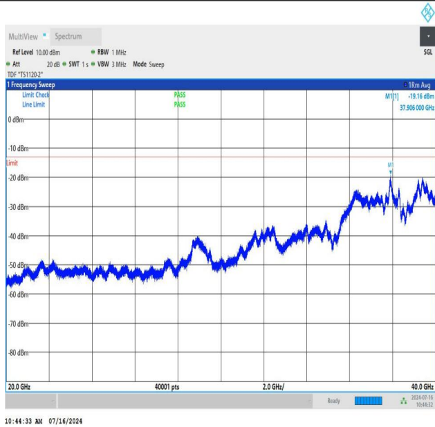
NTNV_N78-3450-3550_PC2_30_40_H_TID2_NS_01_20000_400_00_#1
