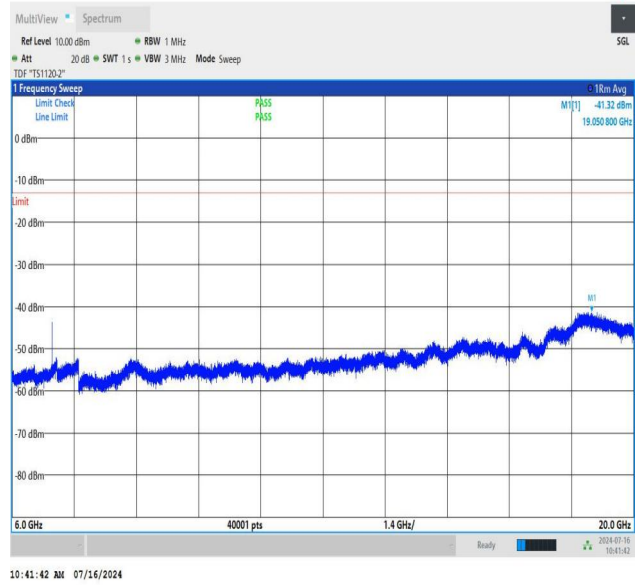
NTNV_N78-3450-3550_PC2_30_40_L_TID2_NS_01_6000_20000_
