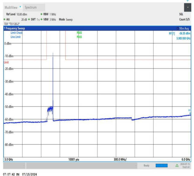
NTNV_N77-3700-3980_PC2_30_90_L_TID3_NS_01_3000_6000_#1
