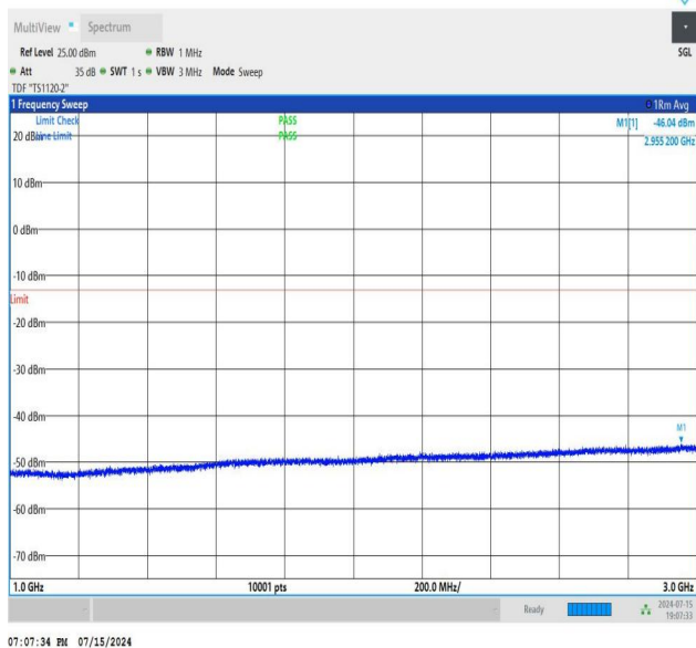
NTNV_N77-3700-3980_PC2_30_90_L_TID3_NS_01_1000_3000_#1
