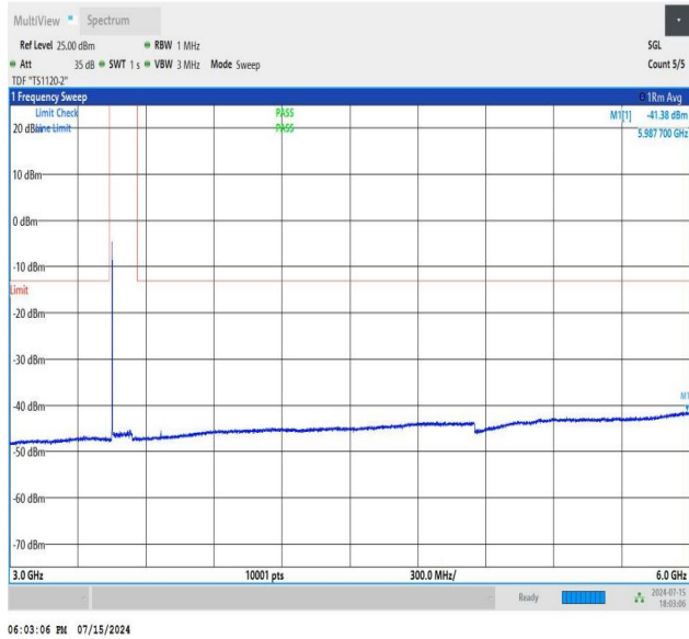
NTNV_N77-3450-3550_PC2_30_90_L_TID2_NS_01_3000_6000_#1
