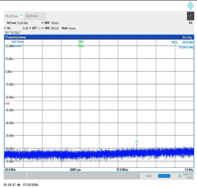
NTNV_N77-3450-3550_PC2_30_80_L_TID3_NS_01_30_1000_#1
