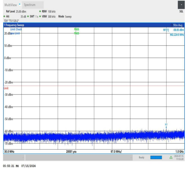
NTNV_N77-3450-3550_PC2_30_60_L_TID3_NS_01_30_1000_#1
