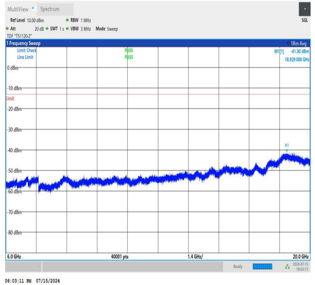
NTNV_N77-3450-3550_PC2_30_90_L_TID2_NS_01_6000_20000_#1
