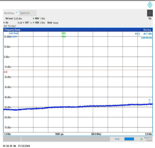
NTNV_N77-3450-3550_PC2_30_60_L_TID2_NS_01_1000_3000_#1
