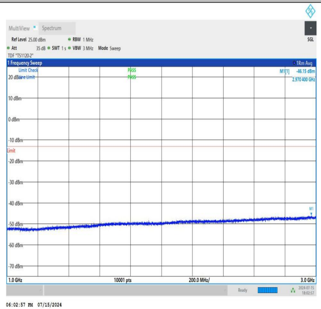
NTNV_N77-3450-3550_PC2_30_90_L_TID2_NS_01_1000_3000_#1
