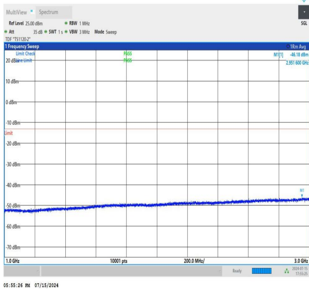
NTNV_N77-3450-3550_PC2_30_60_L_TID3_NS_01_1000_3000_#1
