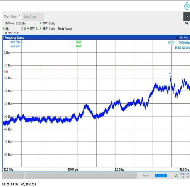
NTNV_N77-3450-3550_PC2_30_90_L_TID2_NS_01_20000_4000_0_#1
