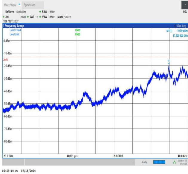
NTNV_N77-3450-3550_PC2_30_80_L_TID2_NS_01_20000_4000_0_#1
