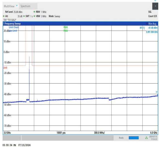
NTNV_N77-3450-3550_PC2_30_60_L_TID3_NS_01_3000_6000_#1
