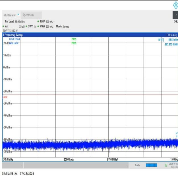
NTNV_N77-3450-3550_PC2_30_50_M_TID2_NS_01_30_1000_#1
