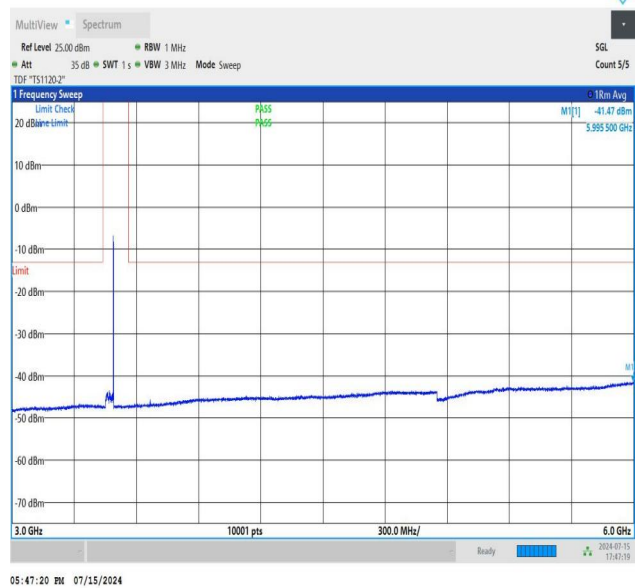
NTNV_N77-3450-3550_PC2_30_40_L_TID3_NS_01_3000_6000_#1
