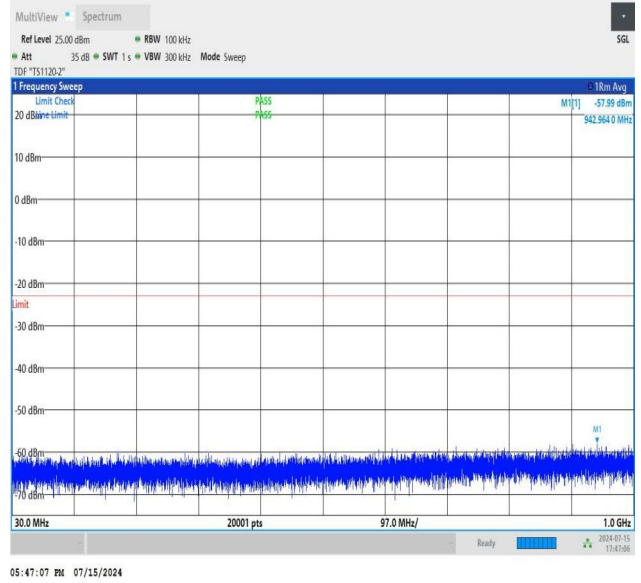
NTNV_N77-3450-3550_PC2_30_40_L_TID3_NS_01_30_1000_#1
