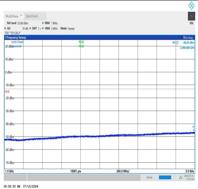
NTNV_N77-3450-3550_PC2_30_50_M_TID2_NS_01_1000_3000_#1
