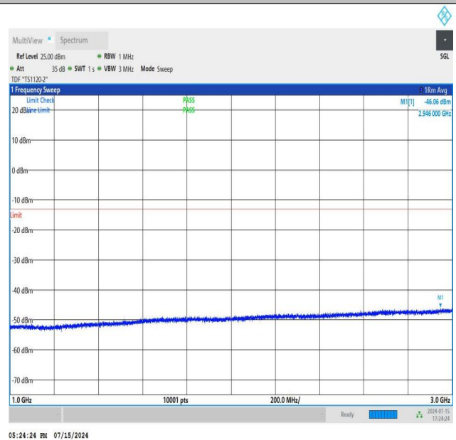
NTNV_N77-3450-3550_PC2_30_60_L_TID2_NS_01_1000_3000_ #1
