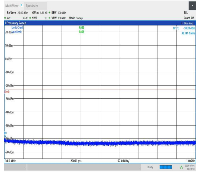
NTNV_DC_26A_n78A-3450-3550_PC3_30_5+80_M+L_TID2_NS _01_30_1000_#1
