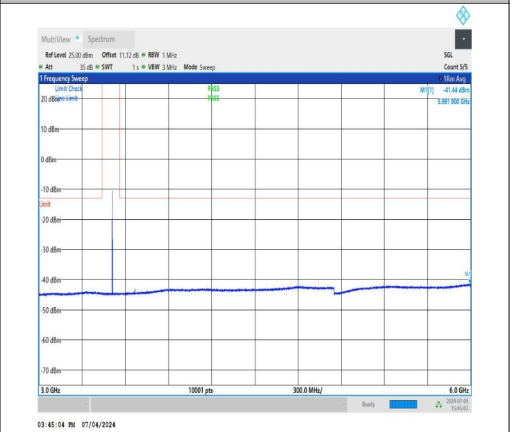
NTNV_DC_26A_n78A-3450-3550_PC3_30_5+60_M+L_TID2_NS_01_3000_6000_#1
