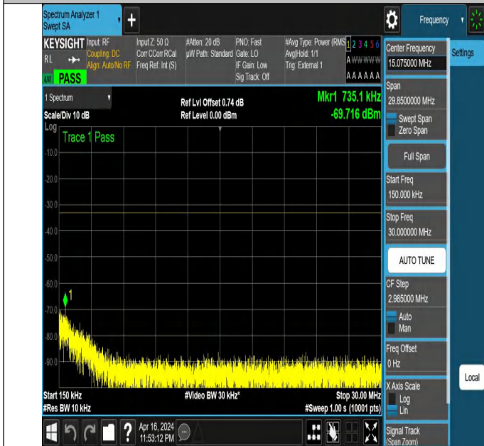
NTNV_N78-3450-3550_PC2_30_100_L_TID6_NS_01_0.15_30_#1
