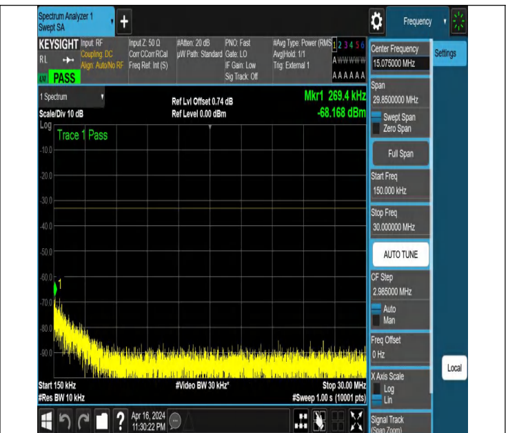
NTNV_N78-3450-3550_PC2_30_100_L_TID2_NS_01_0.15_30_#1
