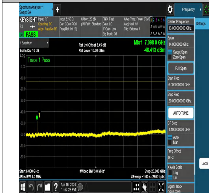
NTNV_N78-3450-3550_PC2_30_100_L_TID6_NS_01_6000_200
