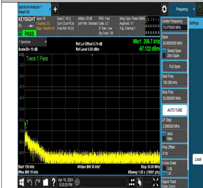
NTNV_N78-3450-3550_PC2_30_80_M_TID6_NS_01_0.15_30_#
