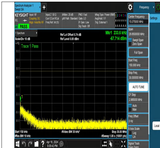
NTNV_N78-3450-3550_PC2_30_80_H_TID3_NS_01_0.15_30_#
