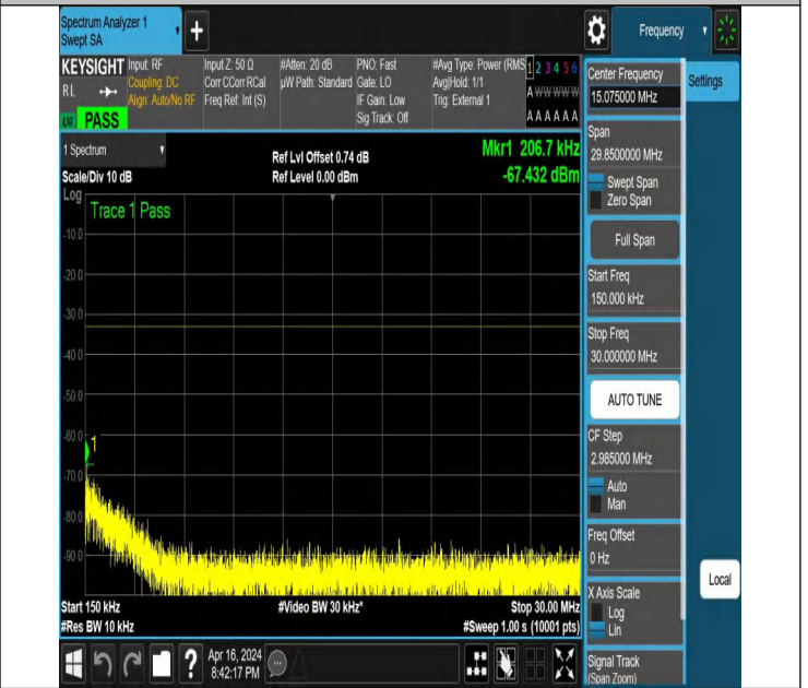
NTNV_N78-3450-3550_PC2_30_80_L_TID5_NS_01_0.15_30_#
