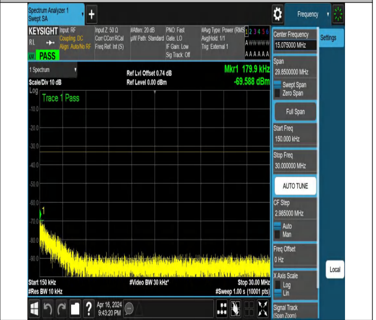
NTNV_N78-3450-3550_PC2_30_80_H_TID5_NS_01_0.15_30_#
