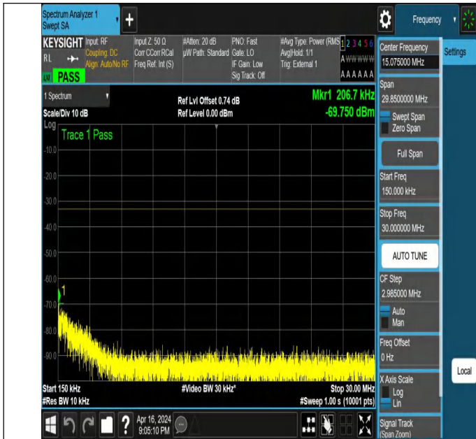
NTNV_N78-3450-3550_PC2_30_80_M_TID3_NS_01_0.15_30_#
