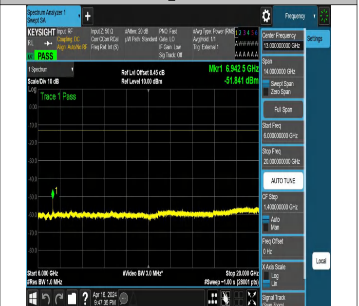
NTNV N78-3450-3550 PC2 30 80 H TID5 NS 01 6000 2000
