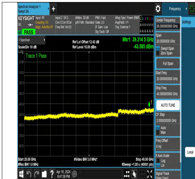
NTNV_N78-3450-3550_PC2_30_80_L_TID5_NS_01_20000_400 00 #1
