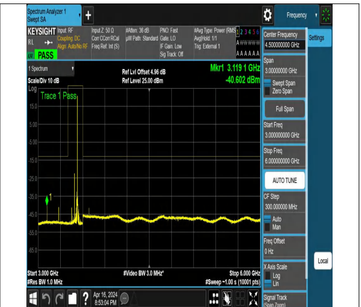
NTNV_N78-3450-3550_PC2_30_80_L_TID6_NS_01_3000_6000
