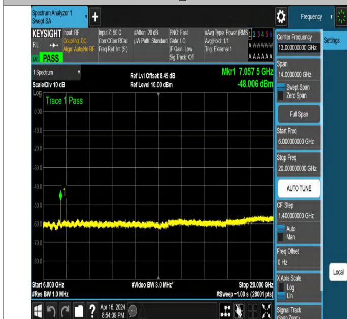
NTNV_N78-3450-3550_PC2_30_80_L_TID6_NS_01_6000_2000
