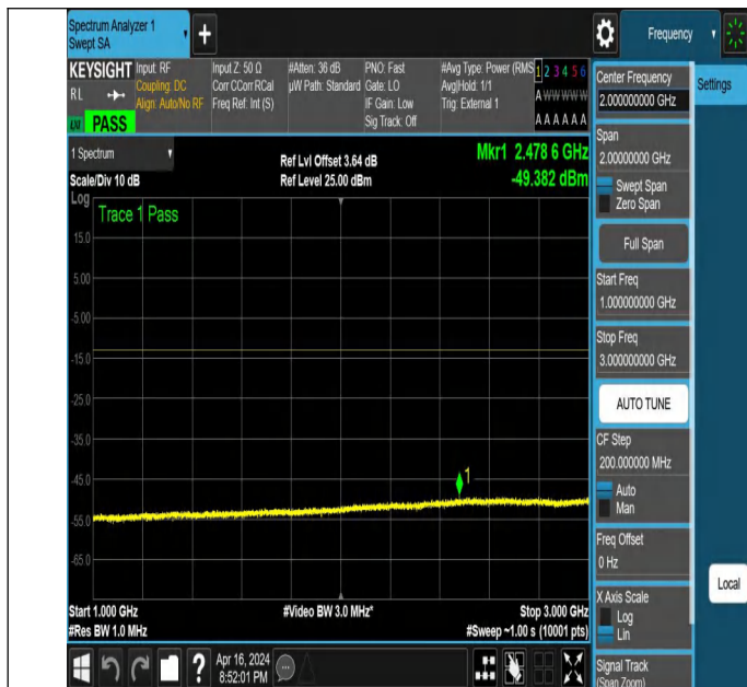
NTNV_N78-3450-3550_PC2_30_80_L_TID6 NS_01_1000_3000
