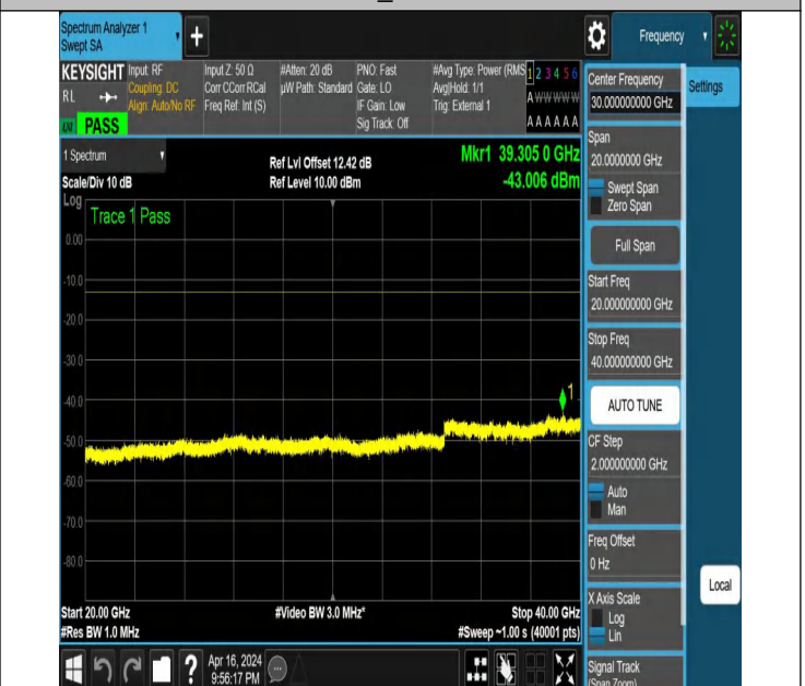
NTNV_N78-3450-3550_PC2_30_80_H_TID6_NS_01_20000_400
