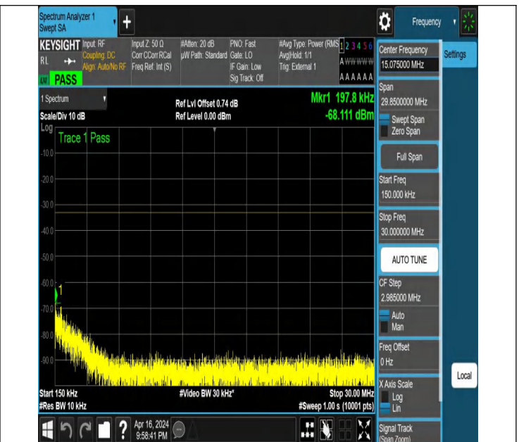
NTNV_N78-3450-3550_PC2_30_90_L_TID2_NS_01_0.15_30_#
