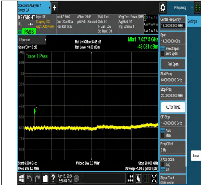
NTNV_N78-3450-3550_PC2_30_80_L_TID3_NS_01_6000_2000
