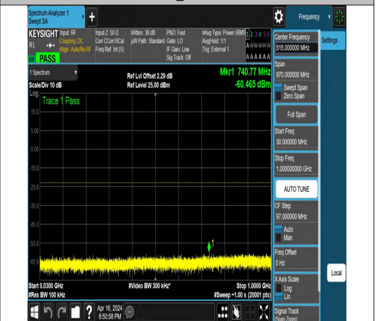
NTNV_N78-3450-3550_PC2_30_80_L_TID6_NS_01_30_1000_#
