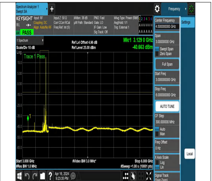
NTNV_N78-3450-3550_PC2_30_80_M_TID6_NS_01_3000_600
