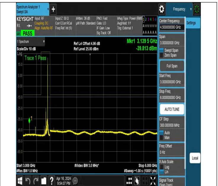
NTNV_N78-3450-3550_PC2_30_80_H_TID6_NS_01_3000_6000
