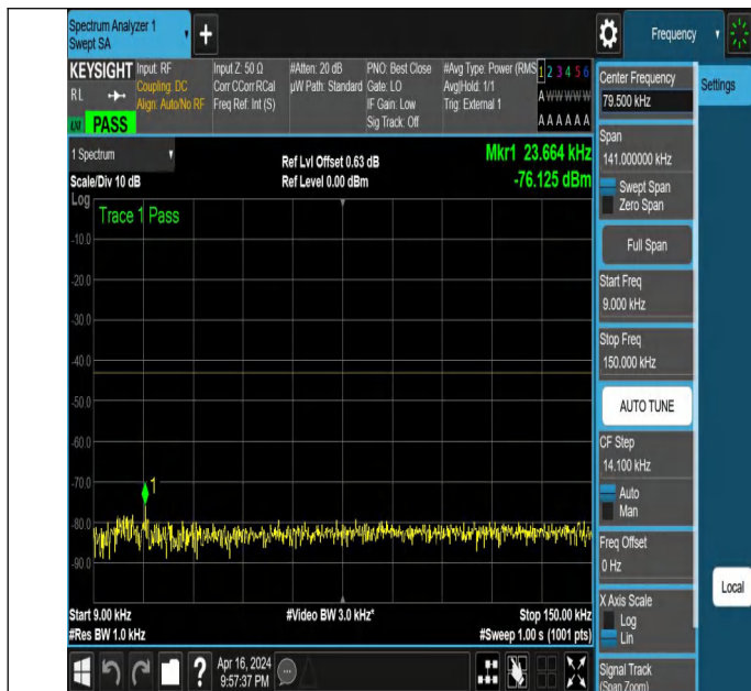
NTNV_N78-3450-3550_PC2_30_90_L_TID2_NS_01_0.009_0.15 #1
