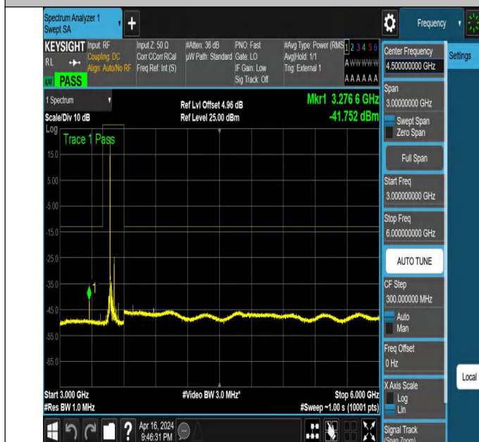
NTNV N78-3450-3550 PC2 30 80 H TID5 NS 01 3000 6000
