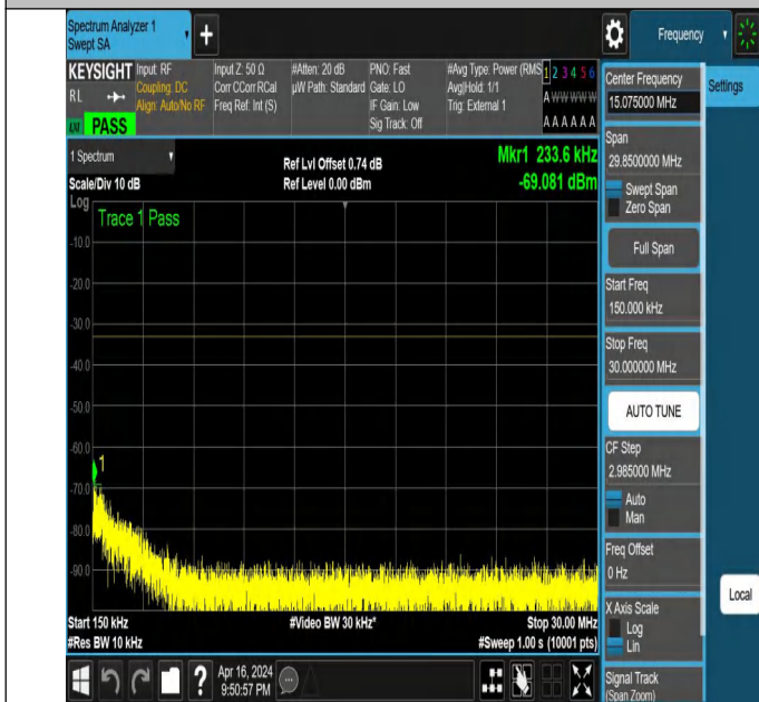
NTNV_N78-3450-3550_PC2_30_80_H_TID6_NS_01_0.15_30_#
