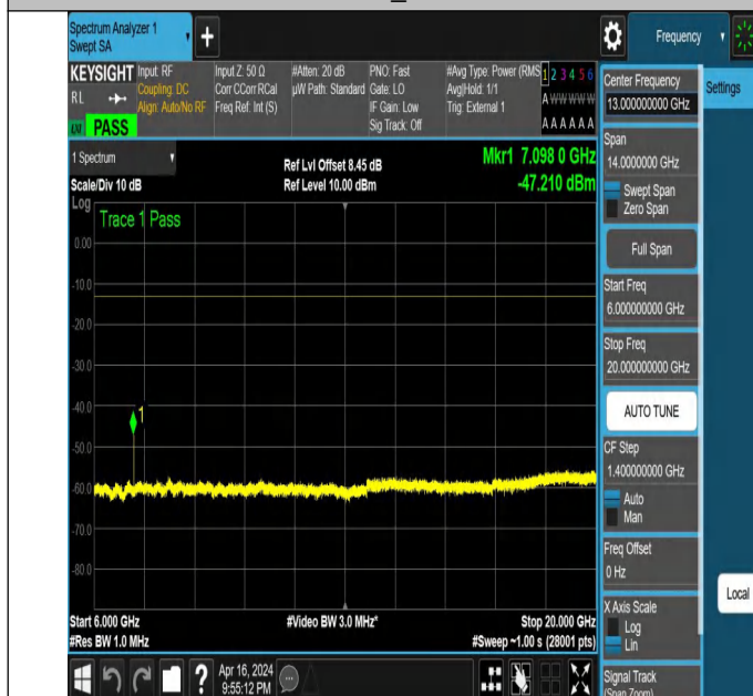
NTNV_N78-3450-3550_PC2_30_80_H_TID6_NS_01_6000_2000
