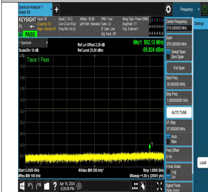
NTNV_N78-3450-3550_PC2_30_80_H_TID2_NS_01_30_1000_#
