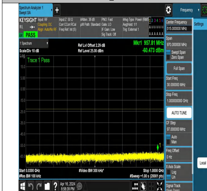
NTNV_N78-3450-3550_PC2_30_80_M_TID2_NS_01_30_1000_#1
