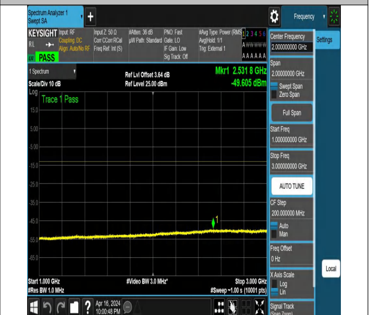
NTNV_N78-3450-3550_PC2_30_90_L_TID2_NS_01_1000_3000
