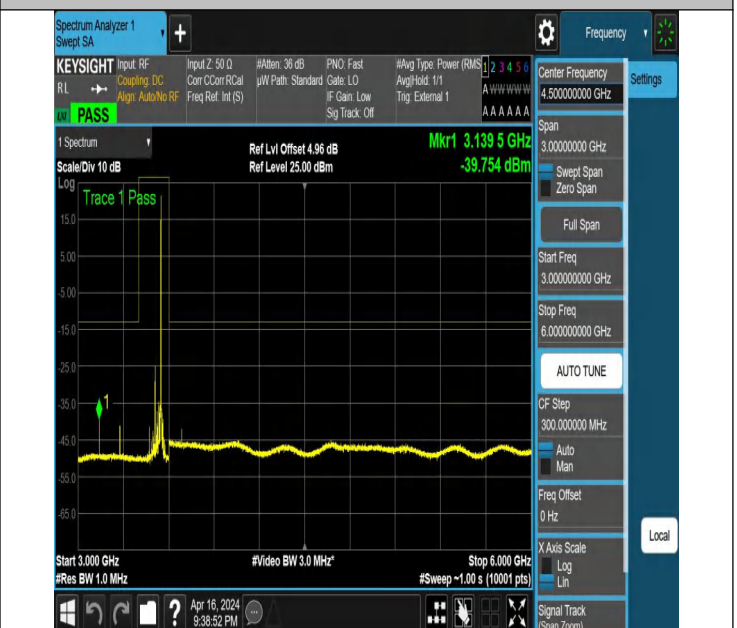
NTNV_N78-3450-3550_PC2_30_80_H_TID3_NS_01_3000_6000
