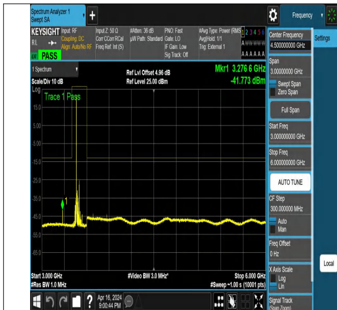
NTNV_N78-3450-3550_PC2_30_80_M_TID2_NS_01_3000_600
