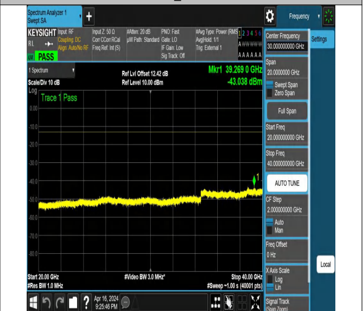
NTNV_N78-3450-3550_PC2_30_80_M_TID6_NS_01_20000_40 000 #1
