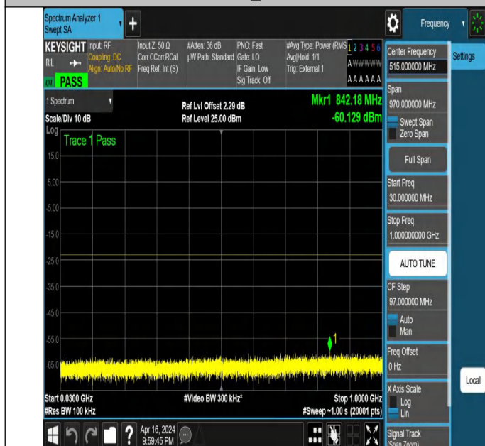
NTNV_N78-3450-3550_PC2_30_90_L_TID2_NS_01_30_1000_#
