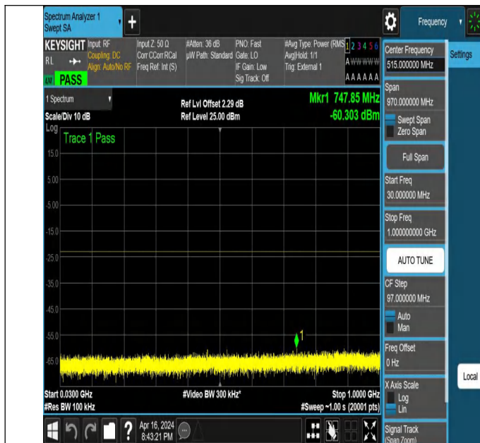
NTNV_N78-3450-3550_PC2_30_80_L_TID5 NS_01_30_1000_#
