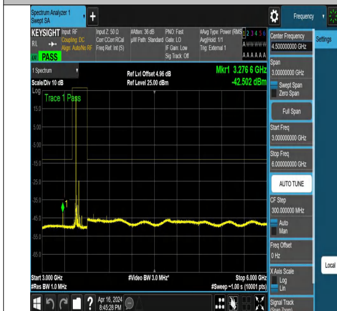
NTNV N78-3450-3550 PC2 30 80 L TID5 NS 01 3000 6000
