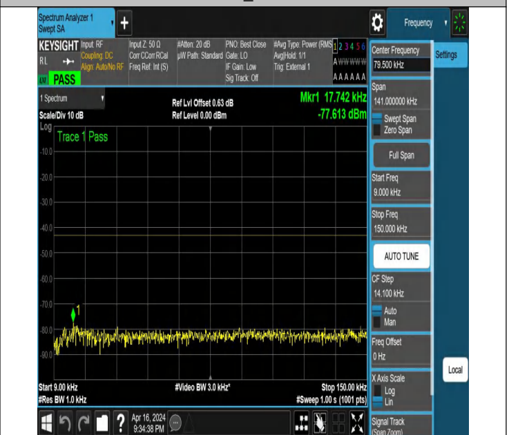
NTNV N78-3450-3550 PC2 30 80 H TID3 NS 01 0.009 0.15
