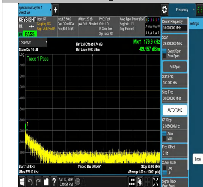
NTNV_N78-3450-3550_PC2_30_80_L_TID6_NS_01_0.15_30_# 1
