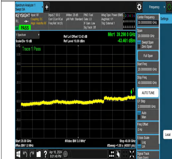
NTNV_N78-3450-3550_PC2_30_70_H_TID2_NS_01_20000_400
