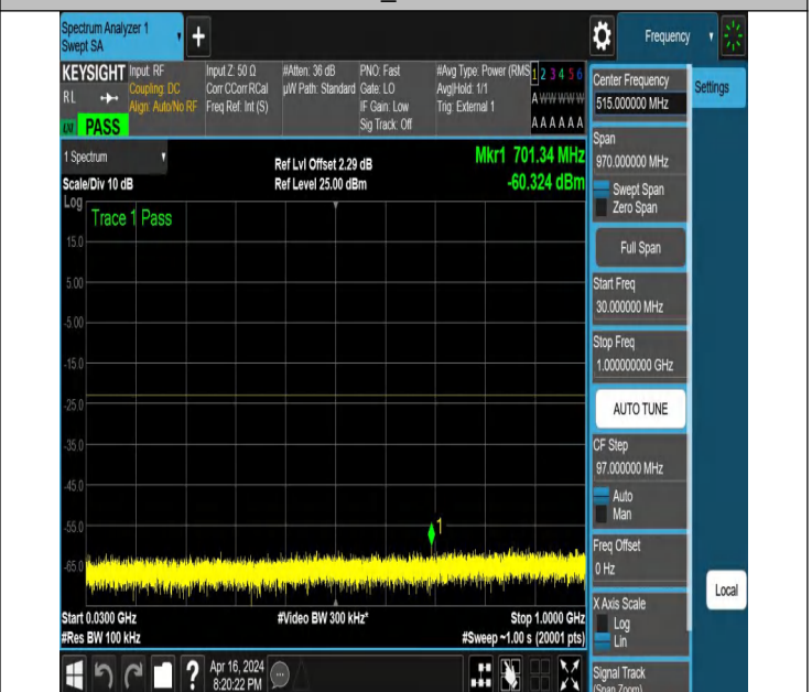
NTNV_N78-3450-3550_PC2_30_70_H_TID6_NS_01_30_1000_# 1
