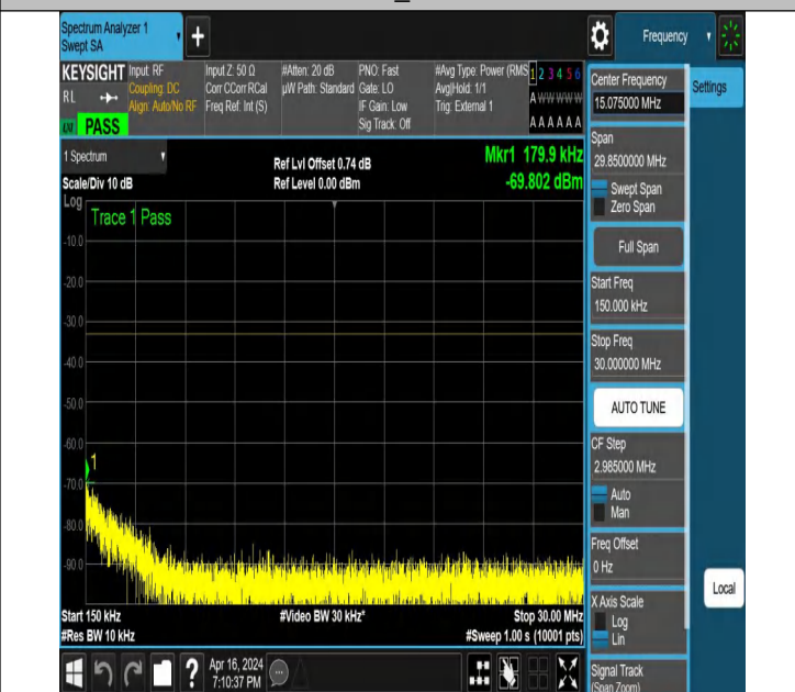
NTNV_N78-3450-3550_PC2_30_70_L_TID5_NS_01_0.15_30_#
