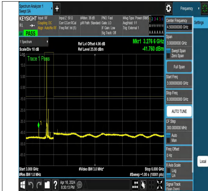
NTNV_N78-3450-3550_PC2_30_80_L_TID2_NS_01_3000_6000
