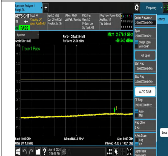
NTNV_N78-3450-3550_PC2_30_70_M_TID3_NS_01_1000_300
