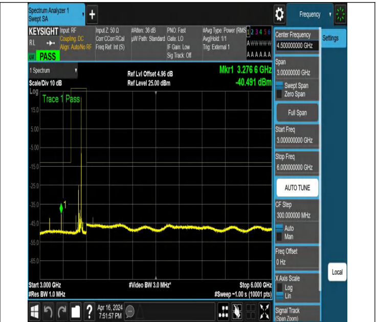
NTNV_N78-3450-3550_PC2_30_70_M_TID6_NS_01_3000_600
