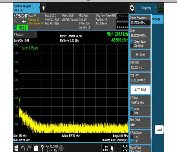
NTNV_N78-3450-3550_PC2_30_70_H_TID5_NS_01_0.15_30_# 1
