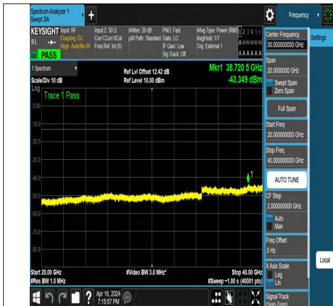
NTNV_N78-3450-3550_PC2_30_70_L_TID5_NS_01_20000_400 00 #1
