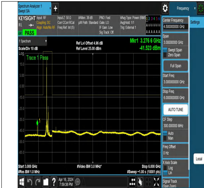
NTNV_N78-3450-3550_PC2_30_70_H_TID2_NS_01_3000_6000
