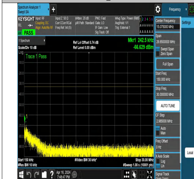
NTNV_N78-3450-3550_PC2_30_70_M_TID6_NS_01_0.15_30_#
