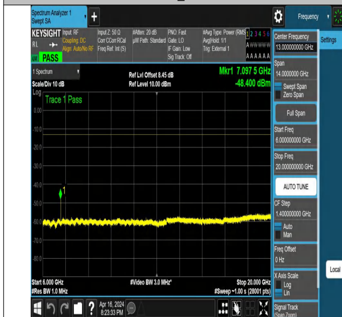
NTNV_N78-3450-3550_PC2_30_70_H_TID6_NS_01_6000_2000
