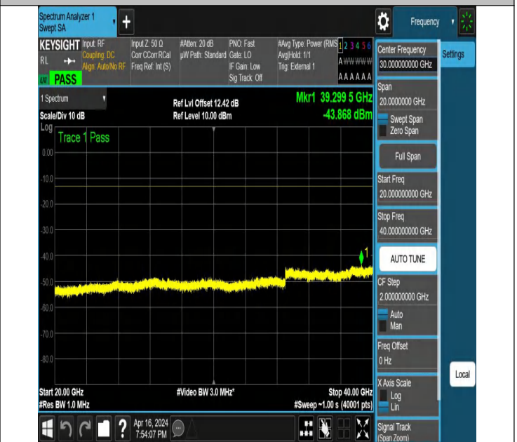
NTNV_N78-3450-3550_PC2_30_70_M_TID6_NS_01_20000_40
