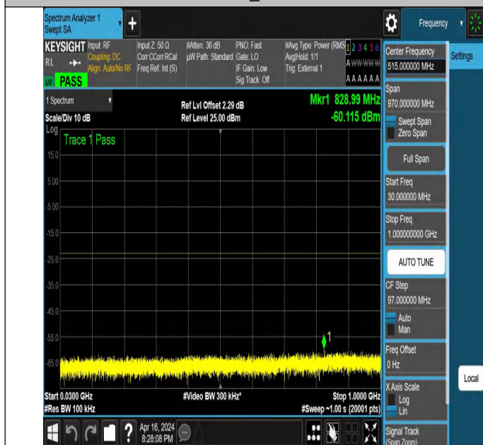
NTNV_N78-3450-3550_PC2_30_80_L_TID2_NS_01_30_1000_#
