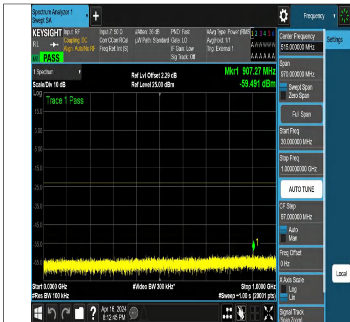
NTNV_N78-3450-3550_PC2_30_70_H_TID5 NS_01_30_1000_#
