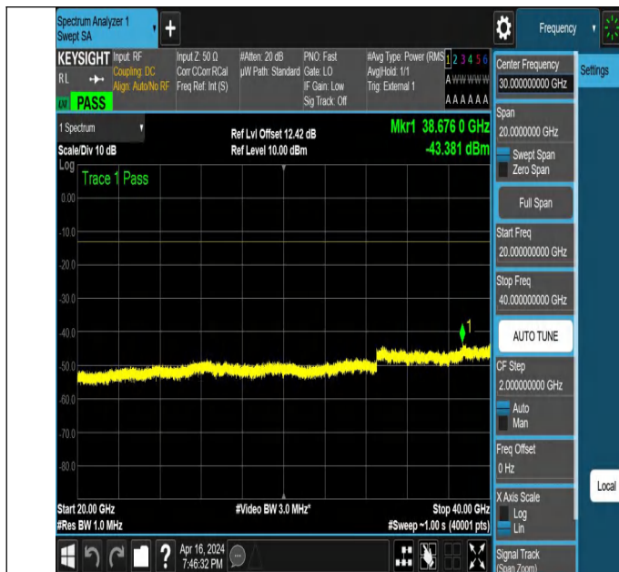
NTNV_N78-3450-3550_PC2_30_70_M_TID5_NS_01_20000_40 000 #1
