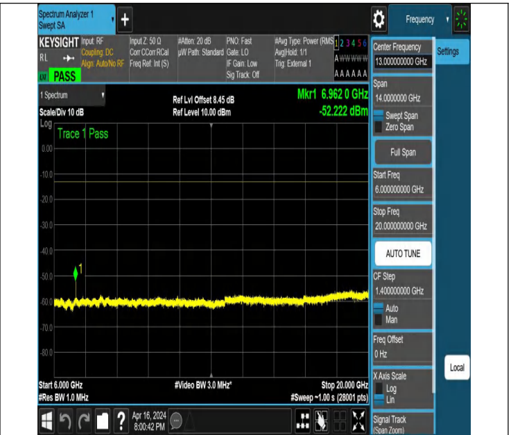
NTNV_N78-3450-3550_PC2_30_70_H_TID2_NS_01_6000_2000
