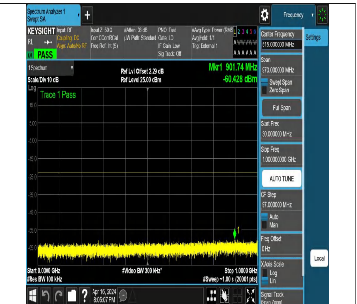
NTNV_N78-3450-3550_PC2_30_70_H_TID3_NS_01_30_1000_#
