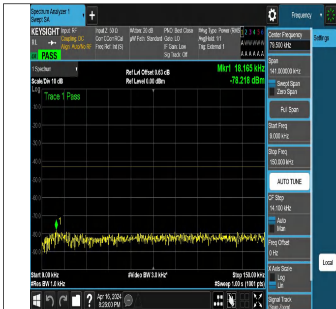
NTNV_N78-3450-3550_PC2_30_80_L_TID2_NS_01_0.009_0.15
