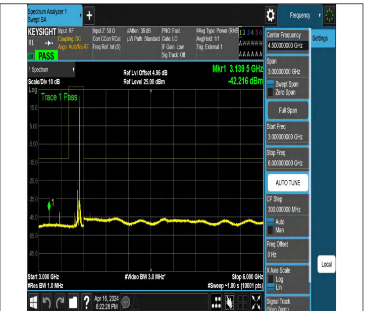
NTNV_N78-3450-3550_PC2_30_70_H_TID6_NS_01_3000_6000
