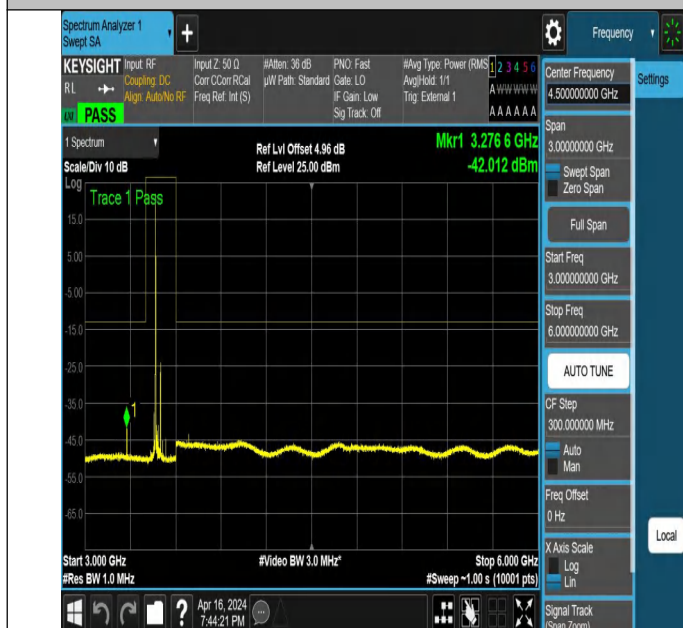
NTNV_N78-3450-3550_PC2_30_70_M_TID5_NS_01_3000_600
