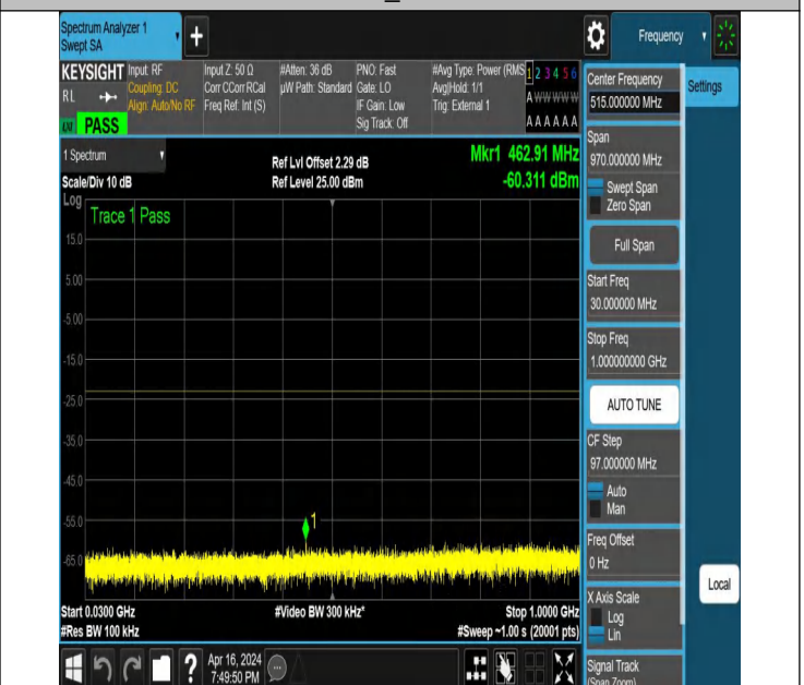
NTNV_N78-3450-3550_PC2_30_70_M_TID6_NS_01_30_1000_
