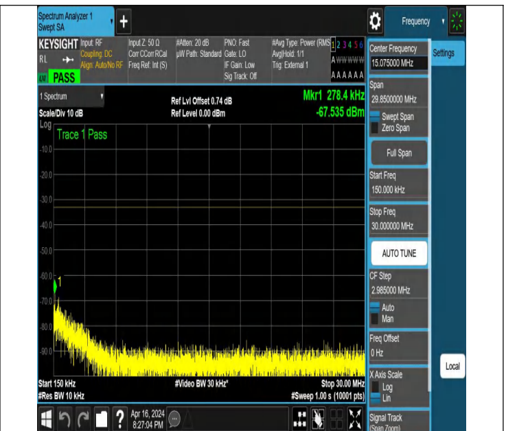
NTNV_N78-3450-3550_PC2_30_80_L_TID2_NS_01_0.15_30_#
