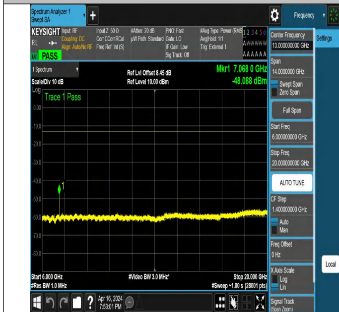
NTNV_N78-3450-3550_PC2_30_70_M_TID6_NS_01_6000_200
