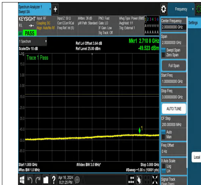
NTNV_N78-3450-3550_PC2_30_70_H_TID6 NS_01_1000_3000
