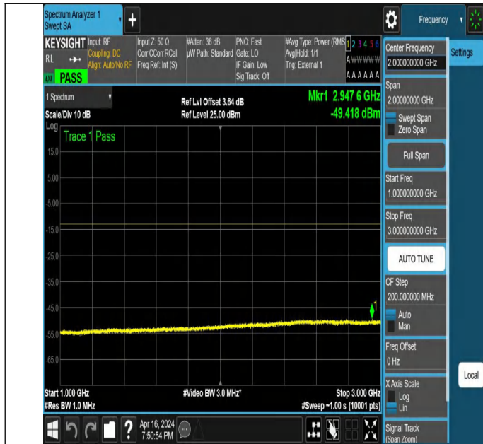
NTNV_N78-3450-3550_PC2_30_70_M_TID6_NS_01_1000_300
