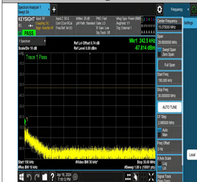
NTNV_N78-3450-3550_PC2_30_70_L_TID6_NS_01_0.15_30_#
