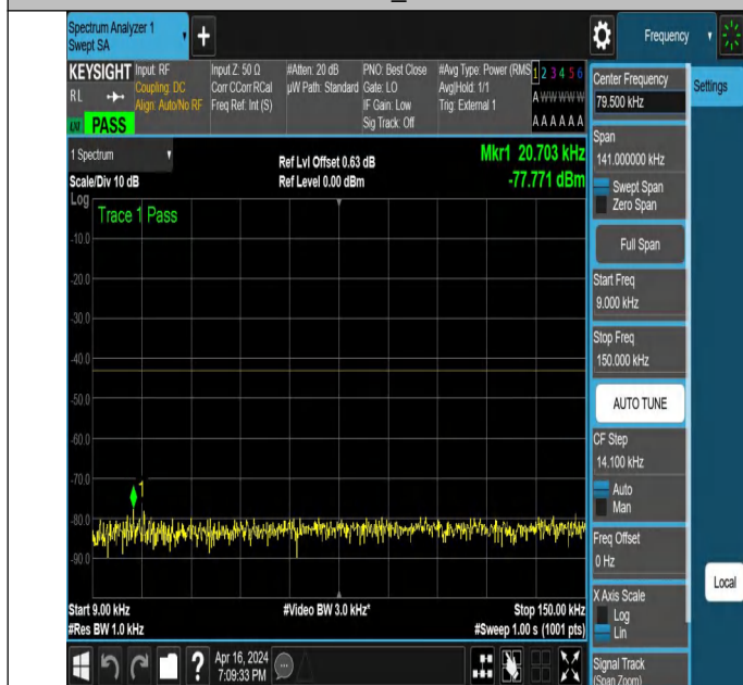
NTNV_N78-3450-3550_PC2_30_70_L_TID5_NS_01_0.009_0.15
