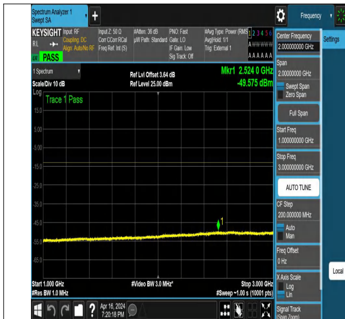
NTNV_N78-3450-3550_PC2_30_70_L_TID6 NS_01_1000_3000
