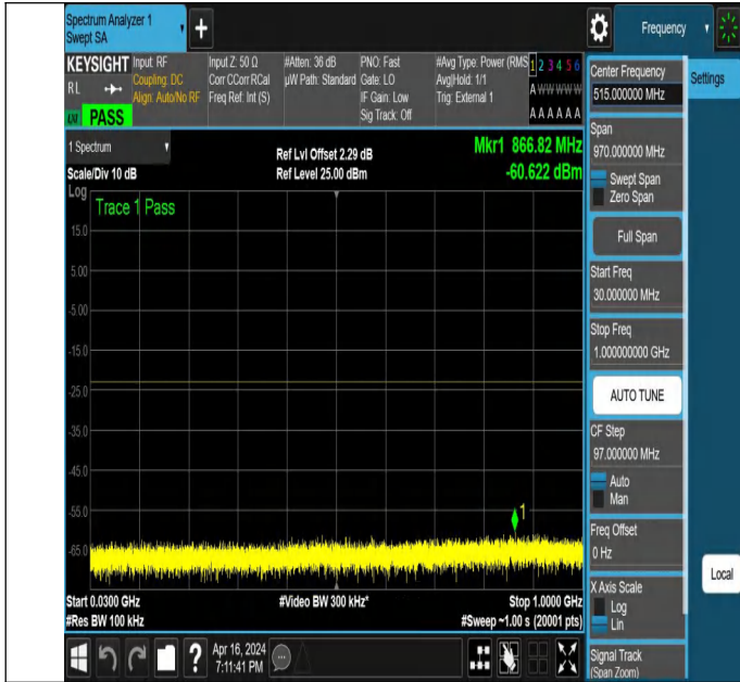
NTNV_N78-3450-3550_PC2_30_70_L_TID5_NS_01_30_1000_#
