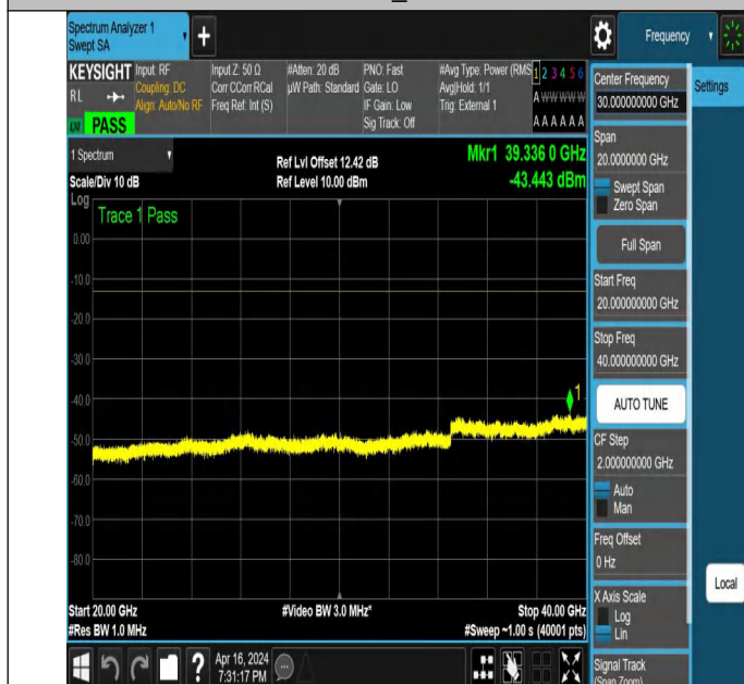
NTNV_N78-3450-3550_PC2_30_70_M_TID2_NS_01_20000_40 000 #1
