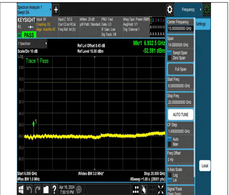
NTNV_N78-3450-3550_PC2_30_70_M_TID2_NS_01_6000_200 00 #1
