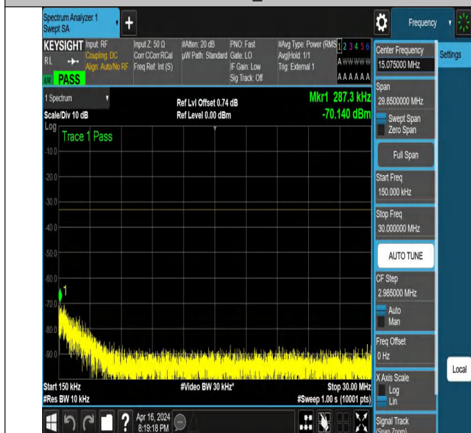
NTNV_N78-3450-3550_PC2_30_70_H_TID6_NS_01_0.15_30_# 1
