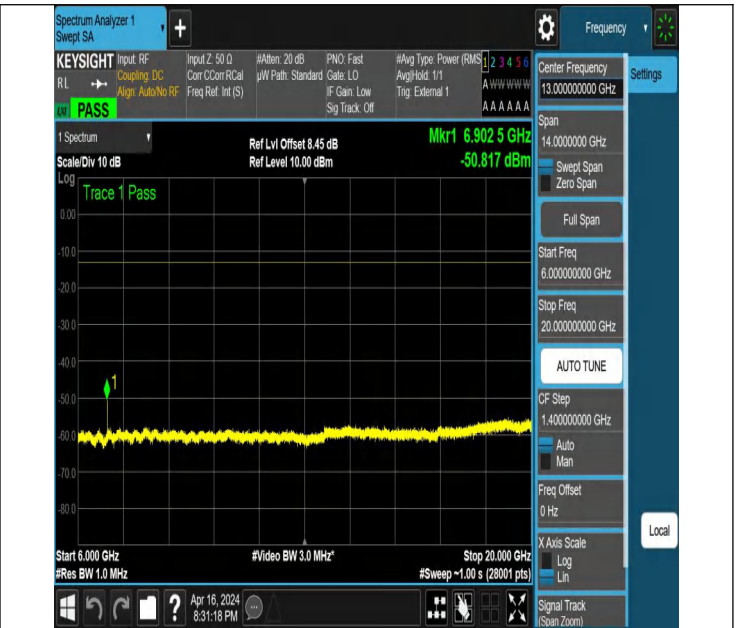
NTNV_N78-3450-3550_PC2_30_80_L_TID2_NS_01_6000_2000
