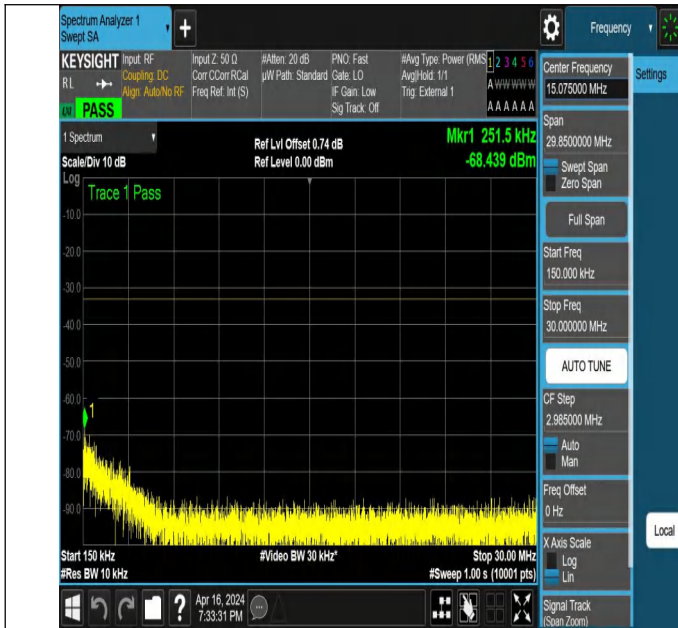
NTNV_N78-3450-3550_PC2_30_70_M_TID3_NS_01_0.15_30_#
