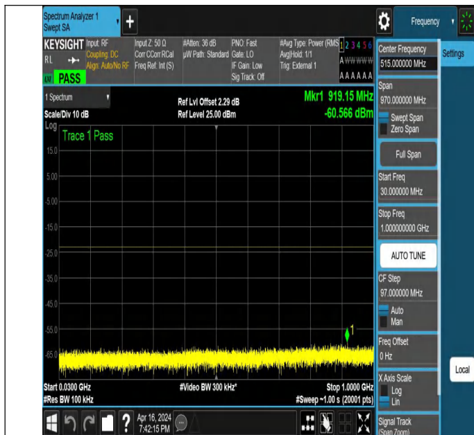
NTNV_N78-3450-3550_PC2_30_70_M_TID5_NS_01_30_1000_#1
