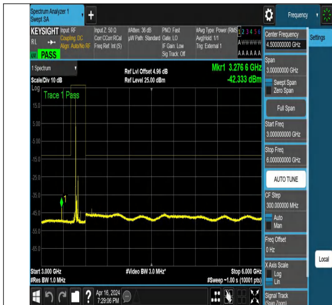
NTNV_N78-3450-3550_PC2_30_70_M_TID2_NS_01_3000_600
