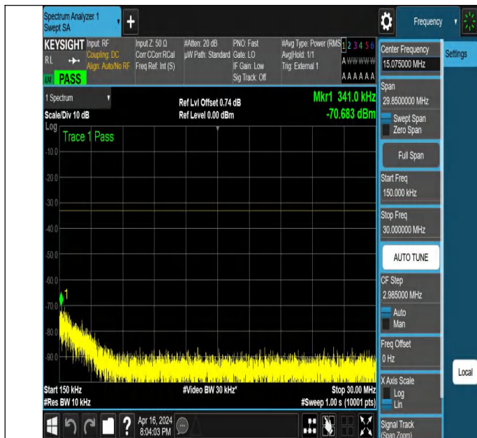
NTNV_N78-3450-3550_PC2_30_70_H_TID3_NS_01_0.15_30_#
