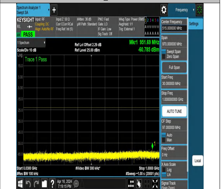
NTNV_N78-3450-3550_PC2_30_70_L_TID6_NS_01_30_1000_#
