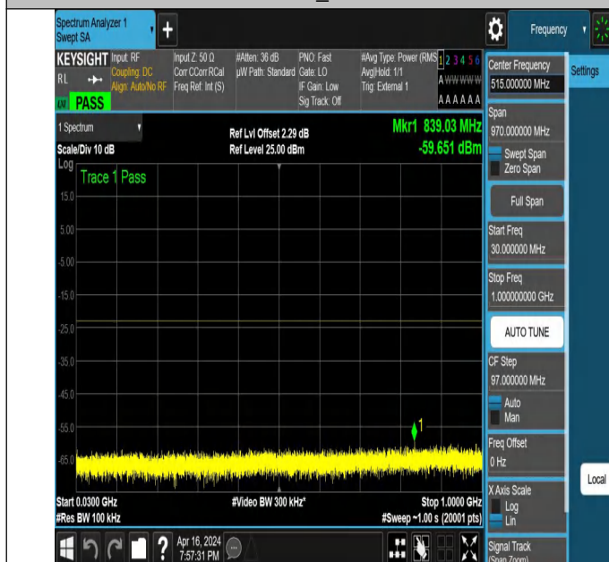
NTNV_N78-3450-3550_PC2_30_70_H_TID2_NS_01_30_1000_# 1
