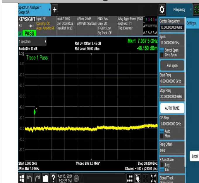
NTNV_N78-3450-3550_PC2_30_70_L_TID6_NS_01_6000_2000
