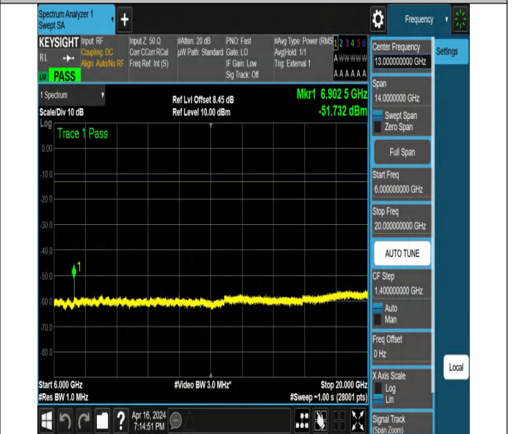
NTNV_N78-3450-3550_PC2_30_70_L_TID5_NS_01_6000_2000
