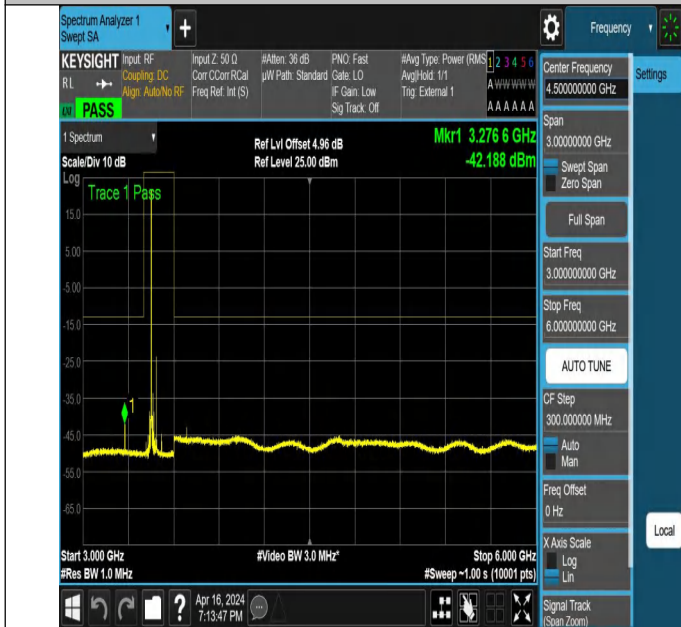
NTNV_N78-3450-3550_PC2_30_70_L_TID5_NS_01_3000_6000
