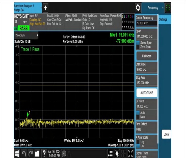
NTNV_N78-3450-3550_PC2_30_70_L_TID6_NS_01_0.009_0.15 #1
