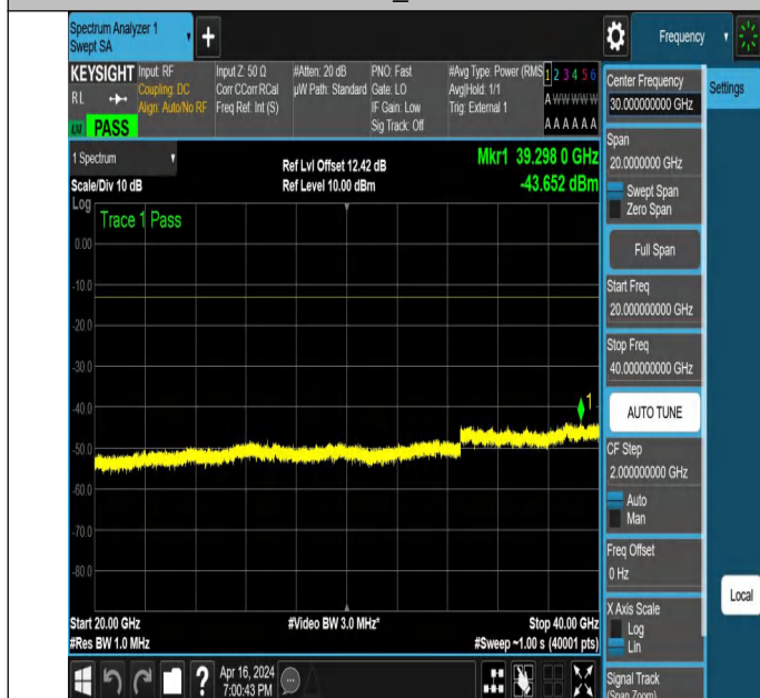
NTNV_N78-3450-3550_PC2_30_70_L_TID2_NS_01_20000_400
