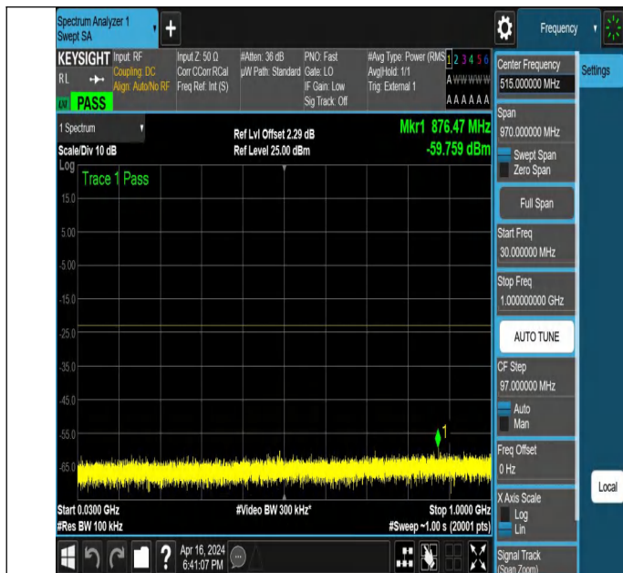
NTNV_N78-3450-3550_PC2_30_60_H_TID5 NS_01_30_1000_#
