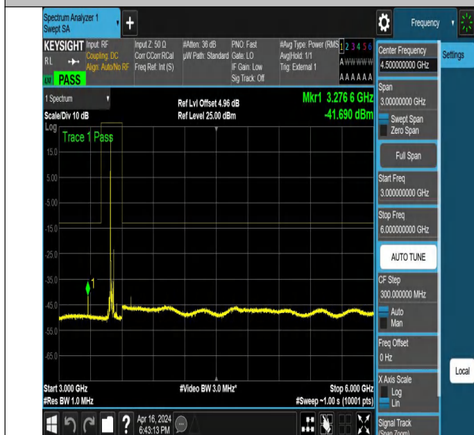
NTNV_N78-3450-3550_PC2_30_60_H_TID5_NS_01_3000_6000
