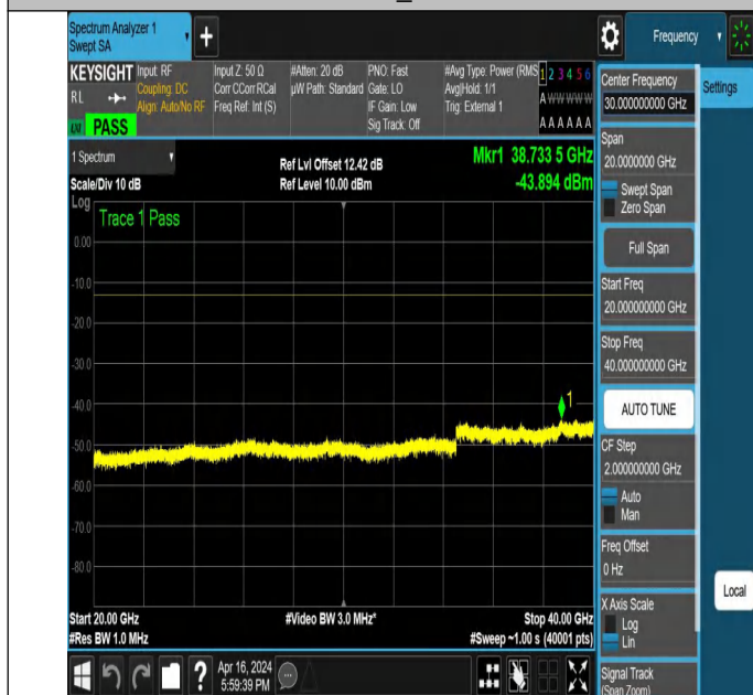
NTNV_N78-3450-3550_PC2_30_60_M_TID2_NS_01_20000_40000_#1
