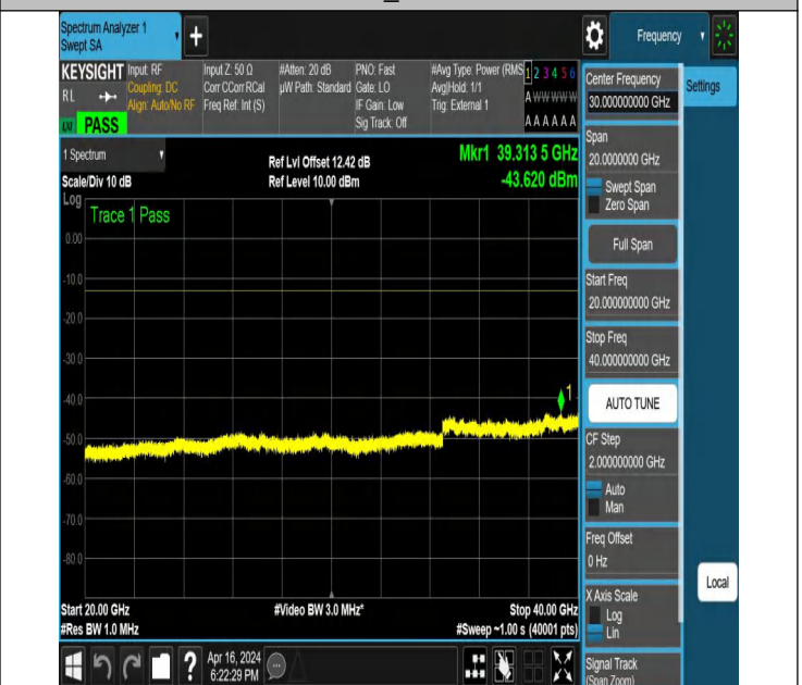
NTNV_N78-3450-3550_PC2_30_60_M_TID6_NS_01_20000_40 000 #1
