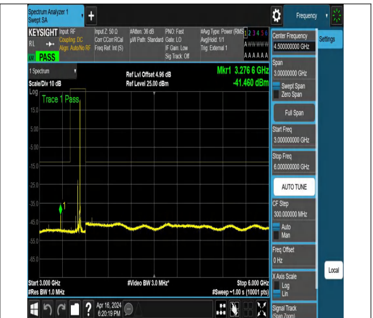
NTNV_N78-3450-3550_PC2_30_60_M_TID6_NS_01_3000_600
