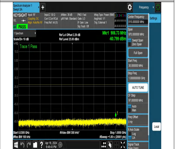
NTNV_N78-3450-3550_PC2_30_60_H_TID6_NS_01_30_1000_#
