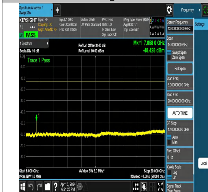
NTNV_N78-3450-3550_PC2_30_60_M_TID6_NS_01_6000_200 00 #1
