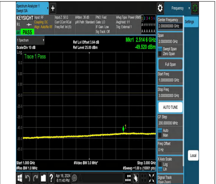
NTNV_N78-3450-3550_PC2_30_60_M_TID5_NS_01_1000_300
