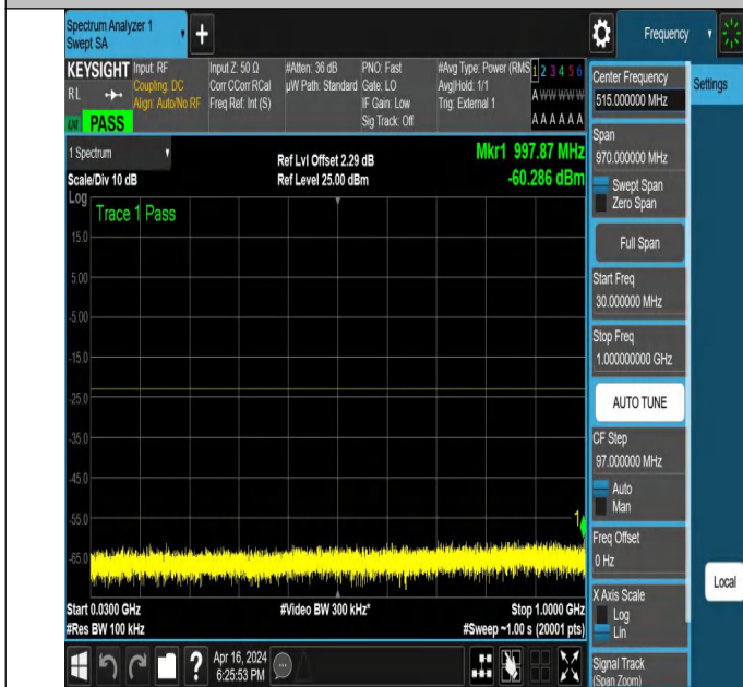
NTNV_N78-3450-3550_PC2_30_60_H_TID2_NS_01_30_1000_#
