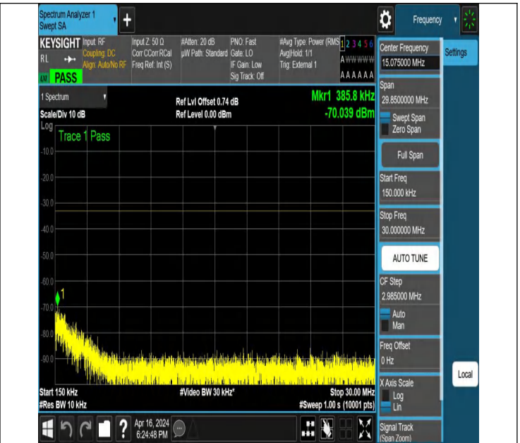
NTNV_N78-3450-3550_PC2_30_60_H_TID2_NS_01_0.15_30_#
