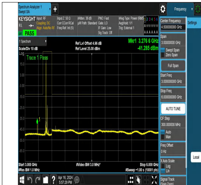
NTNV_N78-3450-3550_PC2_30_60_M_TID2_NS_01_3000_600
