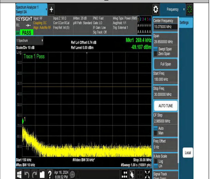
NTNV_N78-3450-3550_PC2_30_60_M_TID5_NS_01_0.15_30_#
