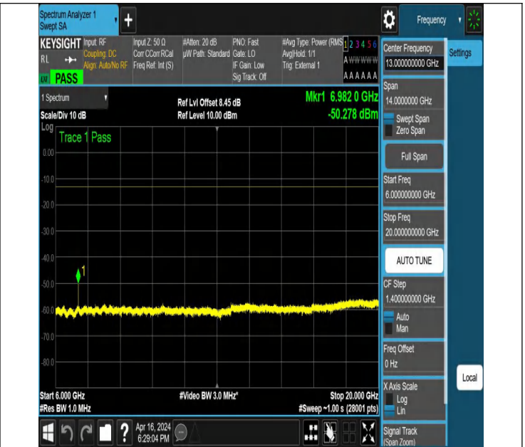
NTNV_N78-3450-3550_PC2_30_60_H_TID2_NS_01_6000_2000
