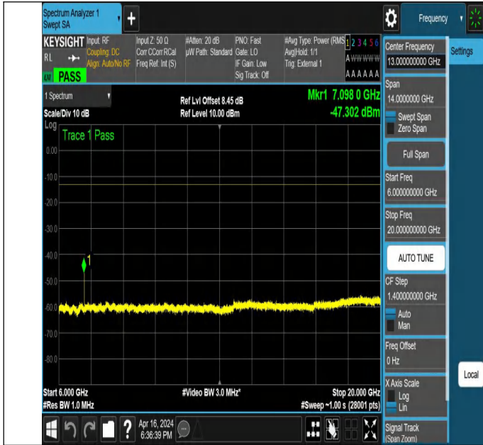
NTNV_N78-3450-3550_PC2_30_60_H_TID3_NS_01_6000_2000
