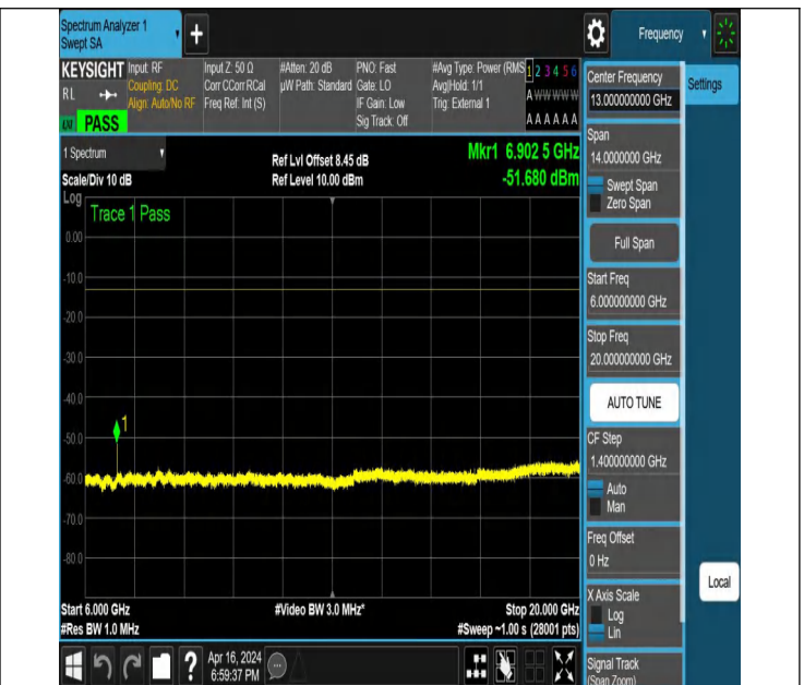
NTNV_N78-3450-3550_PC2_30_70_L_TID2_NS_01_6000_2000
