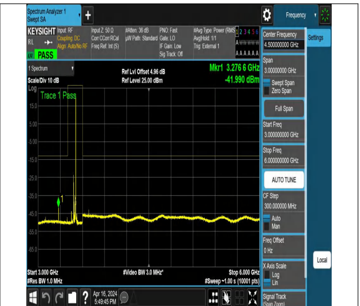
NTNV_N78-3450-3550_PC2_30_60_L_TID6_NS_01_3000_6000
