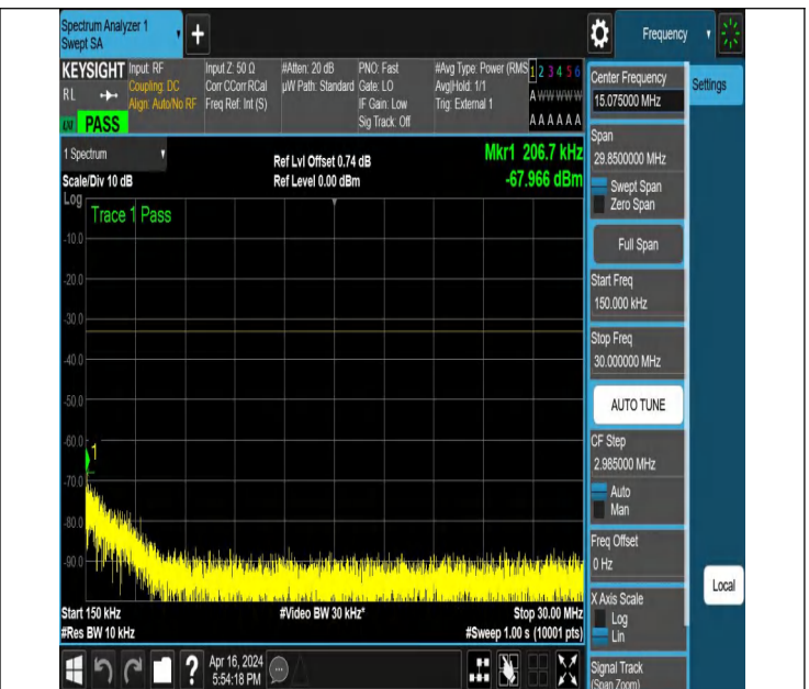
NTNV_N78-3450-3550_PC2_30_60_M_TID2_NS_01_0.15_30_#
