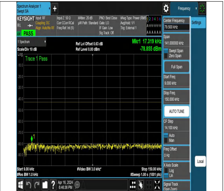
NTNV_N78-3450-3550_PC2_30_60_H_TID6_NS_01_0.009_0.15
