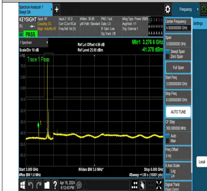
NTNV_N78-3450-3550_PC2_30_60_M_TID5_NS_01_3000_600
