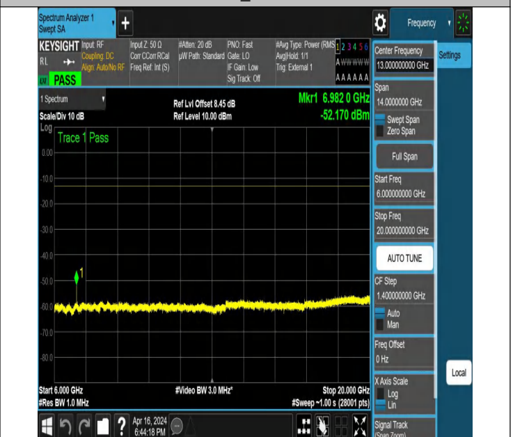
NTNV_N78-3450-3550_PC2_30_60_H_TID5_NS_01_6000_2000
