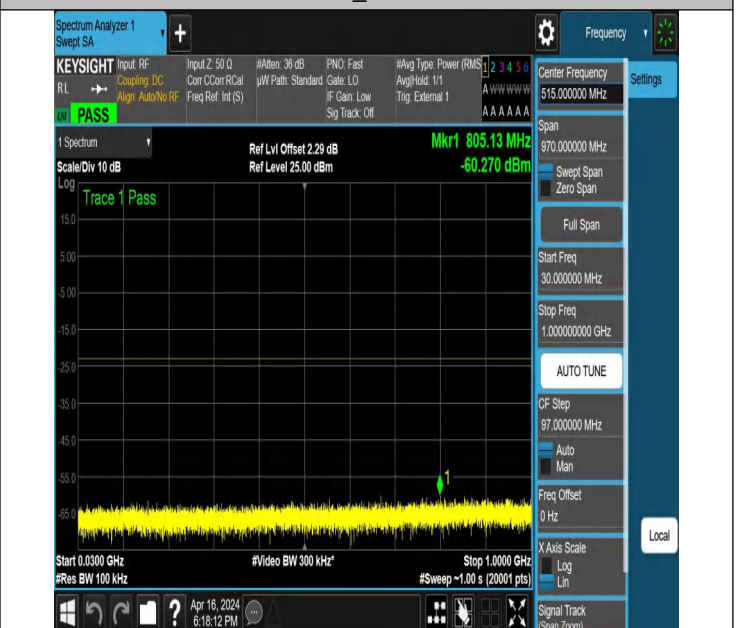
NTNV_N78-3450-3550_PC2_30_60_M_TID6_NS_01_30_1000_ #1
