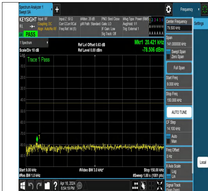
NTNV_N78-3450-3550_PC2_30_70_L_TID2_NS_01_0.009_0.15
