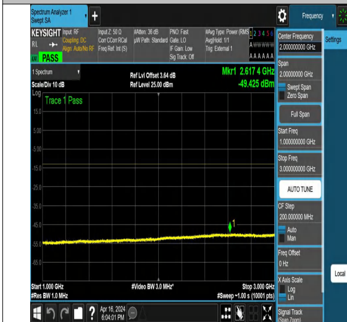
NTNV_N78-3450-3550_PC2_30_60_M_TID3_NS_01_1000_300
