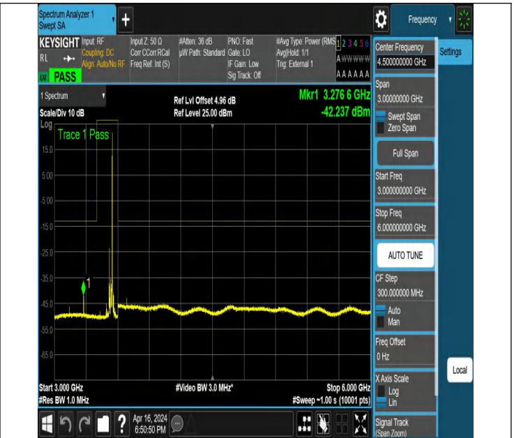
NTNV_N78-3450-3550_PC2_30_60_H_TID6_NS_01_3000_6000
