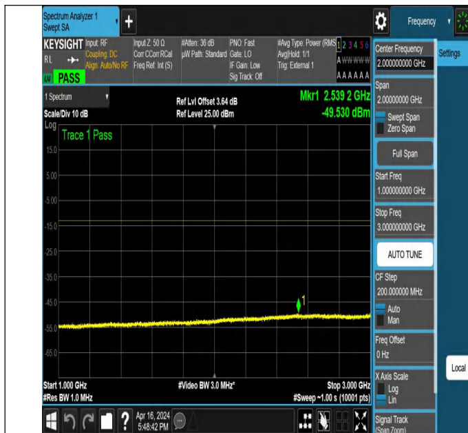
NTNV_N78-3450-3550_PC2_30_60_L_TID6 NS_01_1000_3000
