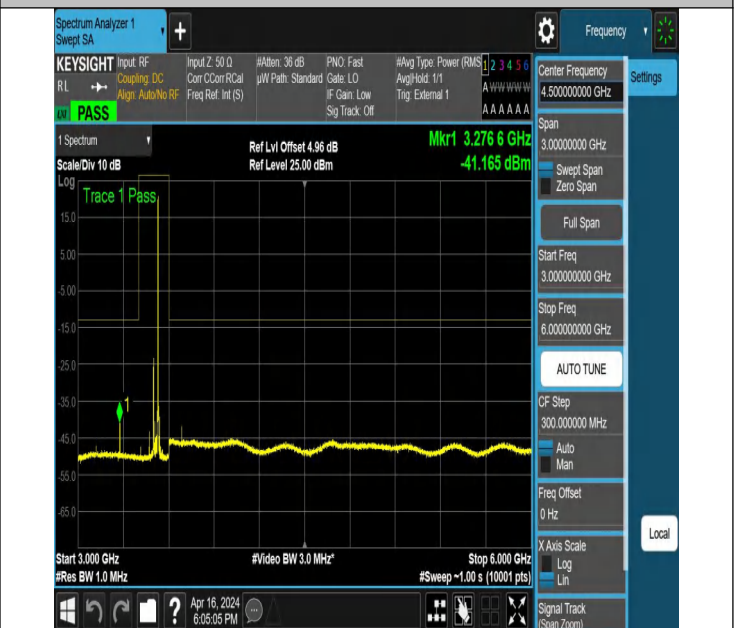
NTNV_N78-3450-3550_PC2_30_60_M_TID3_NS_01_3000_600
