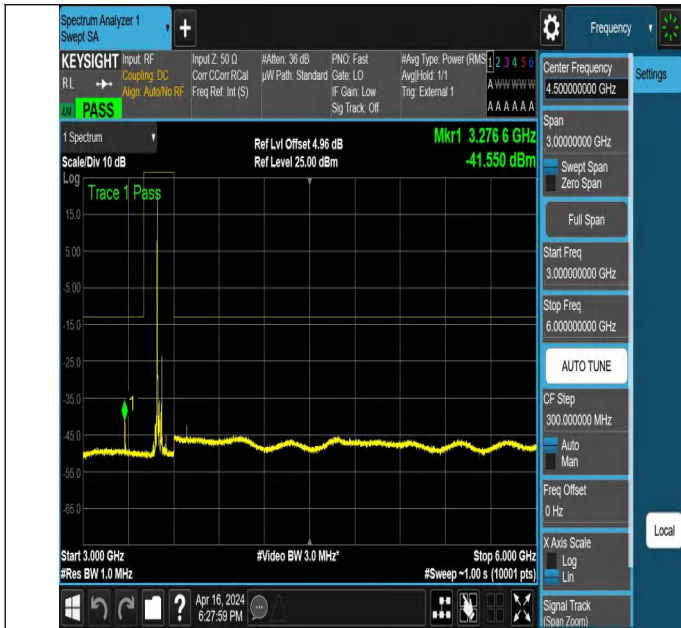
NTNV_N78-3450-3550_PC2_30_60_H_TID2_NS_01_3000_6000
