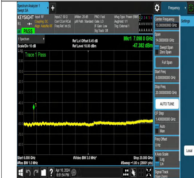
NTNV_N78-3450-3550_PC2_30_60_H_TID6_NS_01_6000_2000
