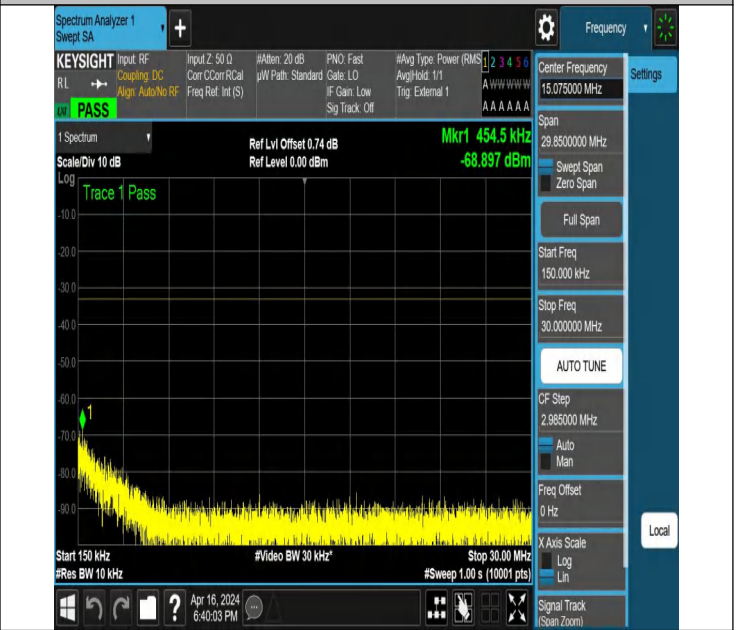
NTNV_N78-3450-3550_PC2_30_60_H_TID5_NS_01_0.15_30_#
