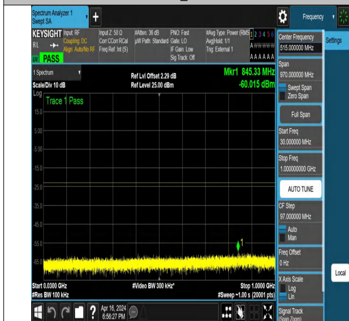
NTNV_N78-3450-3550_PC2_30_70_L_TID2_NS_01_30_1000_# 1
