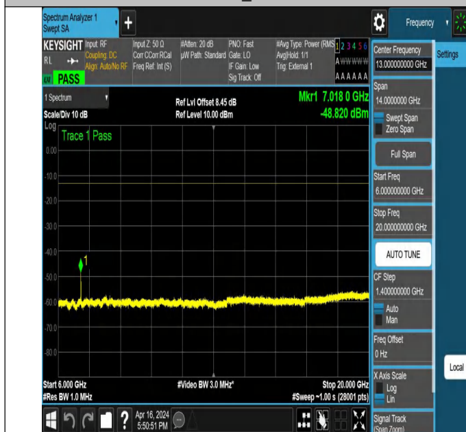
NTNV_N78-3450-3550_PC2_30_60_L_TID6_NS_01_6000_2000
