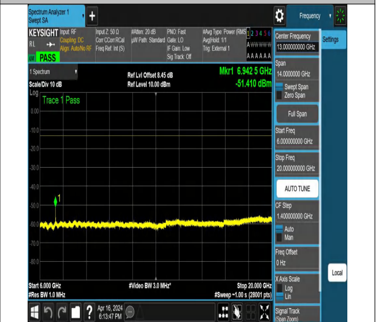
NTNV_N78-3450-3550_PC2_30_60_M_TID5_NS_01_6000_200
