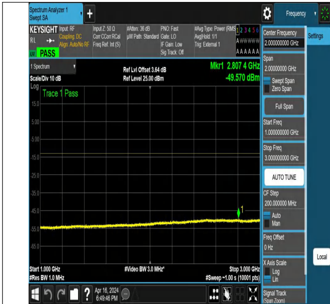
NTNV_N78-3450-3550_PC2_30_60_H_TID6_NS_01_1000_3000
