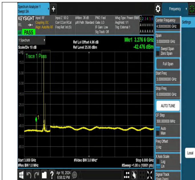
NTNV_N78-3450-3550_PC2_30_70_L_TID2_NS_01_3000_6000
