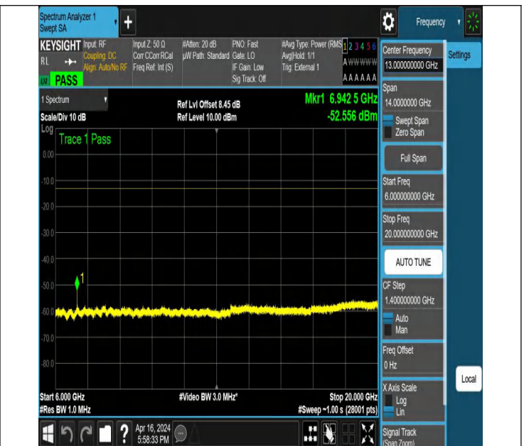
NTNV_N78-3450-3550_PC2_30_60_M_TID2_NS_01_6000_200 00 #1
