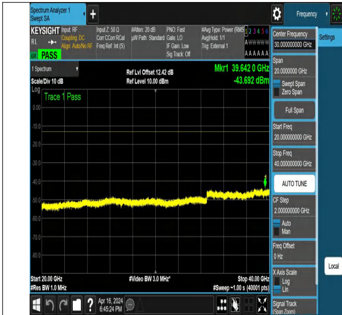
NTNV_N78-3450-3550_PC2_30_60_H_TID5_NS_01_20000_400
