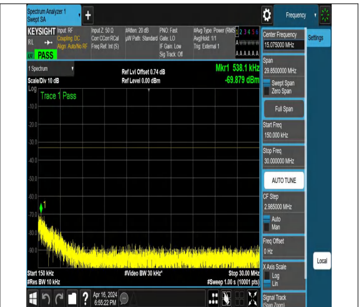
NTNV_N78-3450-3550_PC2_30_70_L_TID2_NS_01_0.15_30_#
