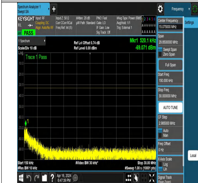
NTNV_N78-3450-3550_PC2_30_60_H_TID6_NS_01_0.15_30_#
