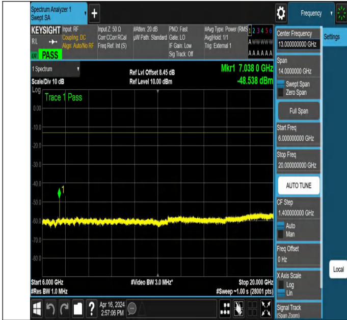
NTNV_N78-3450-3550_PC2_30_40_M_TID3_NS_01_6000_200_00_#1
