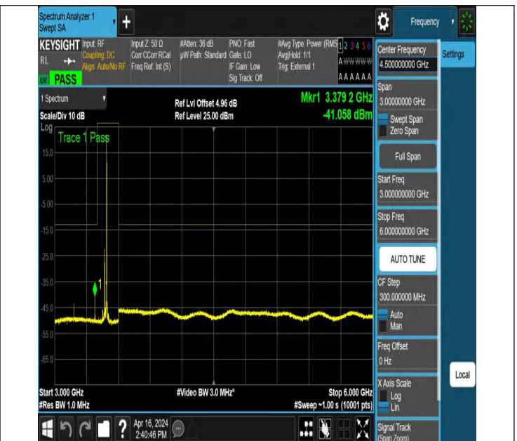
NTNV_N78-3450-3550_PC2_30_40_L_TID6_NS_01_3000_6000
