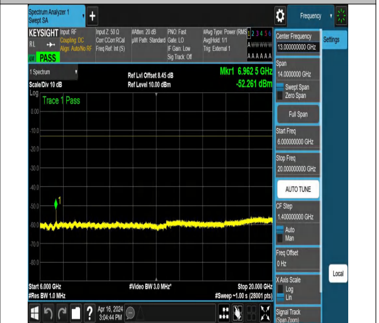
NTNV_N78-3450-3550_PC2_30_40_M_TID5_NS_01_6000_200
