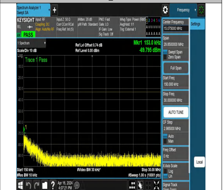
NTNV_N78-3450-3550_PC2_30_50_L_TID5_NS_01_0.15_30_#
