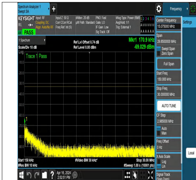
NTNV_N78-3450-3550_PC2_30_40_M_TID3_NS_01_0.15_30_#
