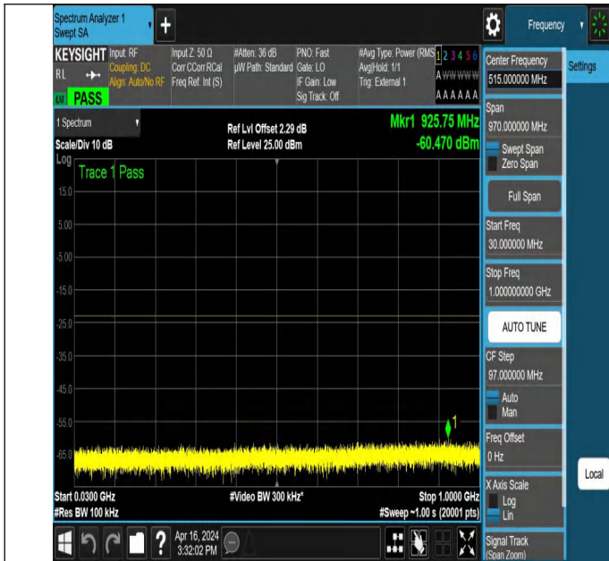
NTNV_N78-3450-3550_PC2_30_40_H_TID5_NS_01_30_1000_#
