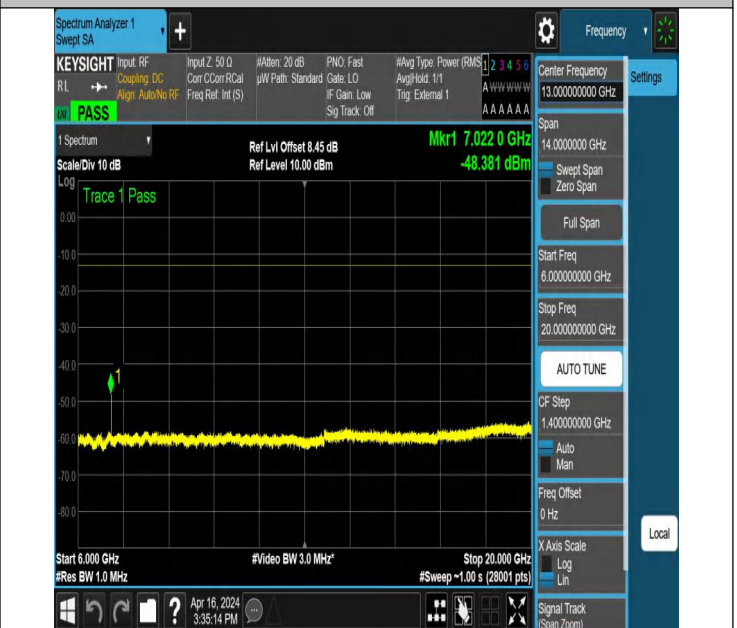
NTNV_N78-3450-3550_PC2_30_40_H_TID5_NS_01_6000_2000_0_#1
