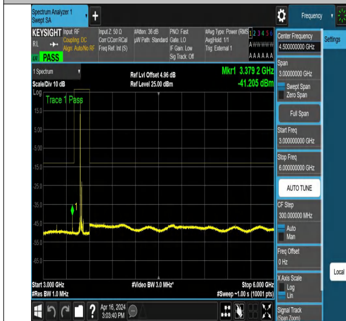
NTNV_N78-3450-3550_PC2_30_40_M_TID5_NS_01_3000_600
