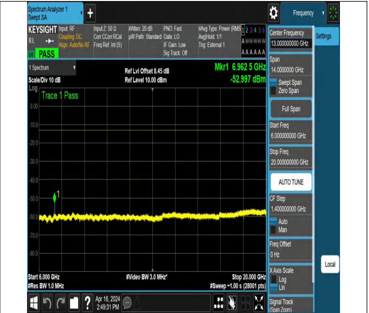
NTNV_N78-3450-3550_PC2_30_40_M_TID2_NS_01_6000_200
