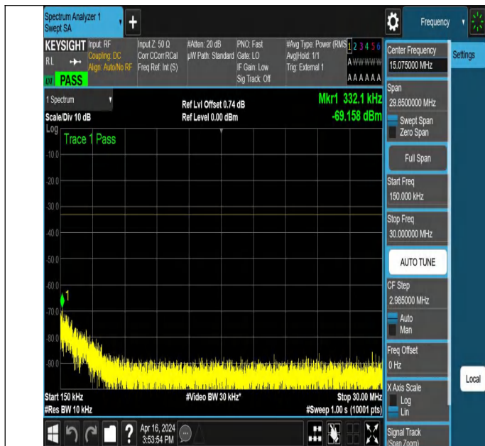
NTNV_N78-3450-3550_PC2_30_50_L_TID3_NS_01_0.15_30_#
