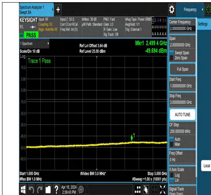
NTNV_N78-3450-3550_PC2_30_40_L_TID6 NS_01_1000_3000
