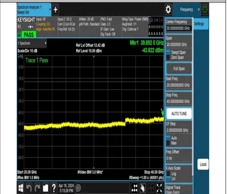
NTNV_N78-3450-3550_PC2_30_40_M_TID6_NS_01_20000_40
