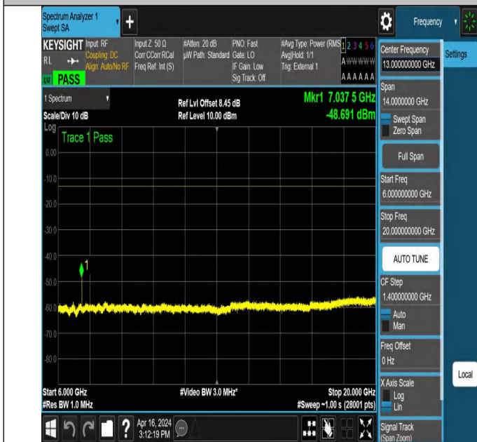
NTNV_N78-3450-3550_PC2_30_40_M_TID6_NS_01_6000_200
