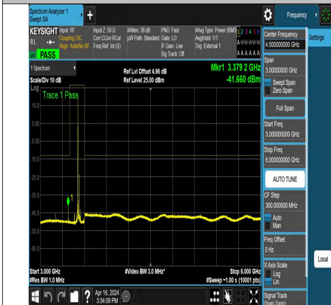
NTNV_N78-3450-3550_PC2_30_40_H_TID5_NS_01_3000_6000_#1
