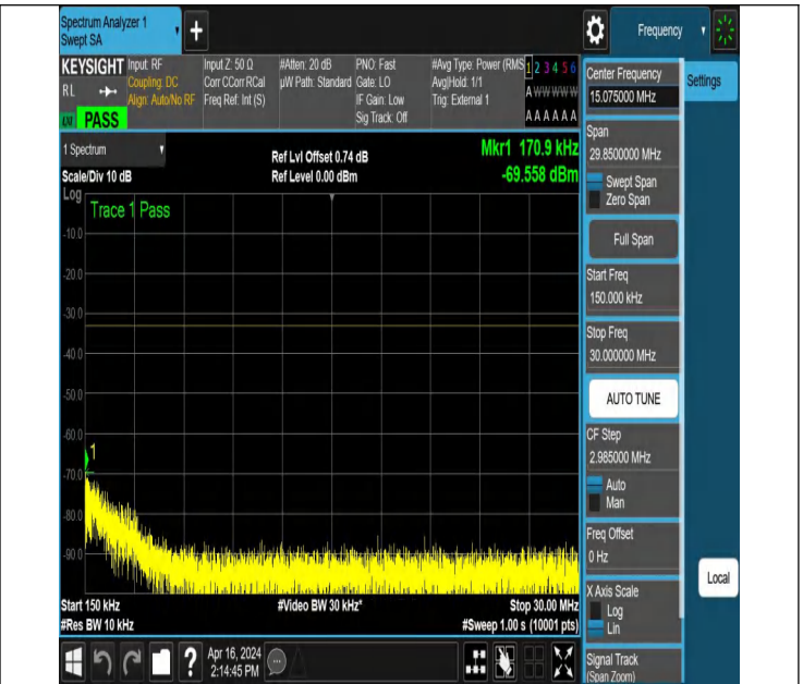
NTNV_N78-3450-3550_PC2_30_40_L_TID2_NS_01_0.15_30_#
