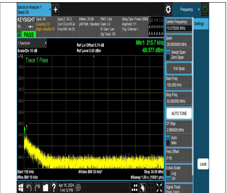
NTNV_N78-3450-3550_PC2_30_30_H_TID2_NS_01_0.15_30_#
