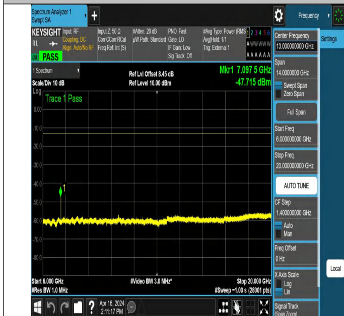
NTNV_N78-3450-3550_PC2_30_30_H_TID6_NS_01_6000_2000
