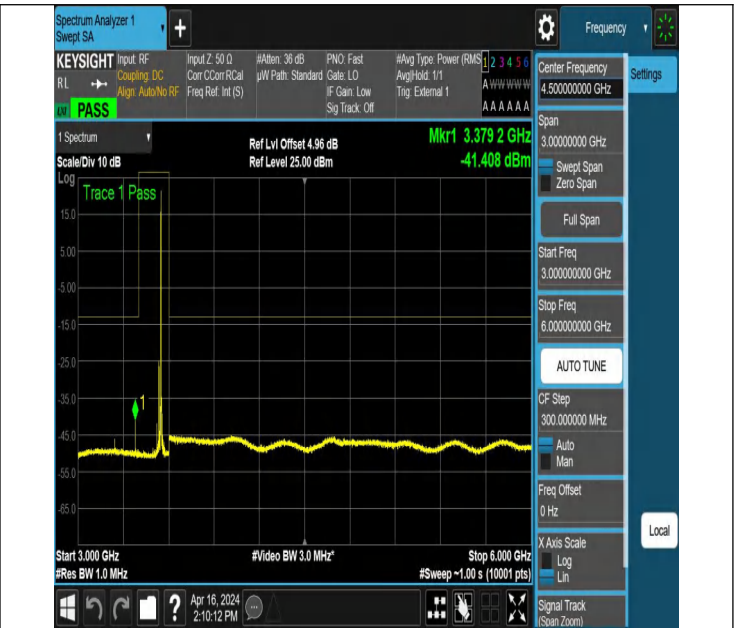
NTNV_N78-3450-3550_PC2_30_30_H_TID6_NS_01_3000_6000
