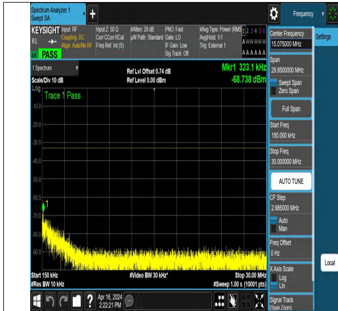
NTNV_N78-3450-3550_PC2_30_40_L_TID3_NS_01_0.15_30_#
