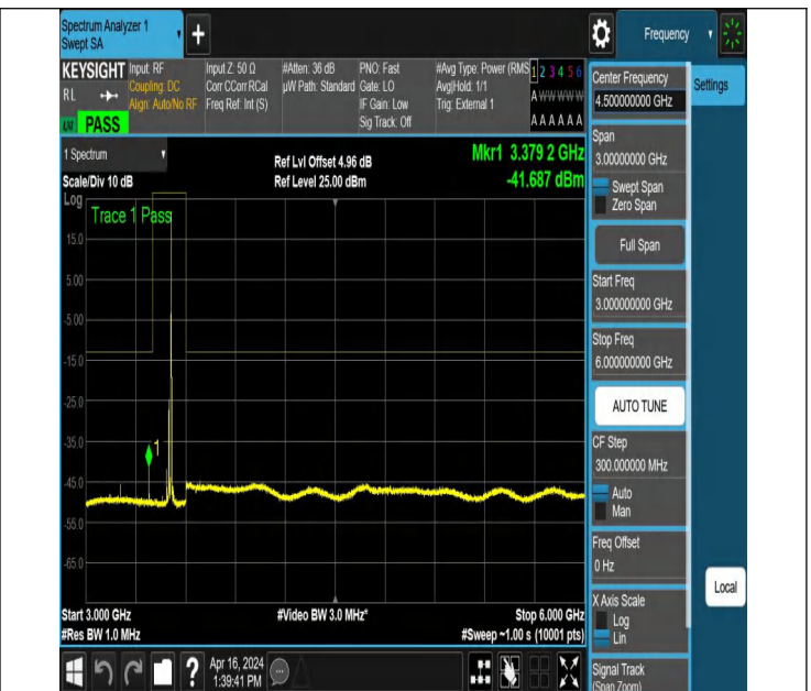
NTNV_N78-3450-3550_PC2_30_30_M_TID6_NS_01_3000_600 0 #1
