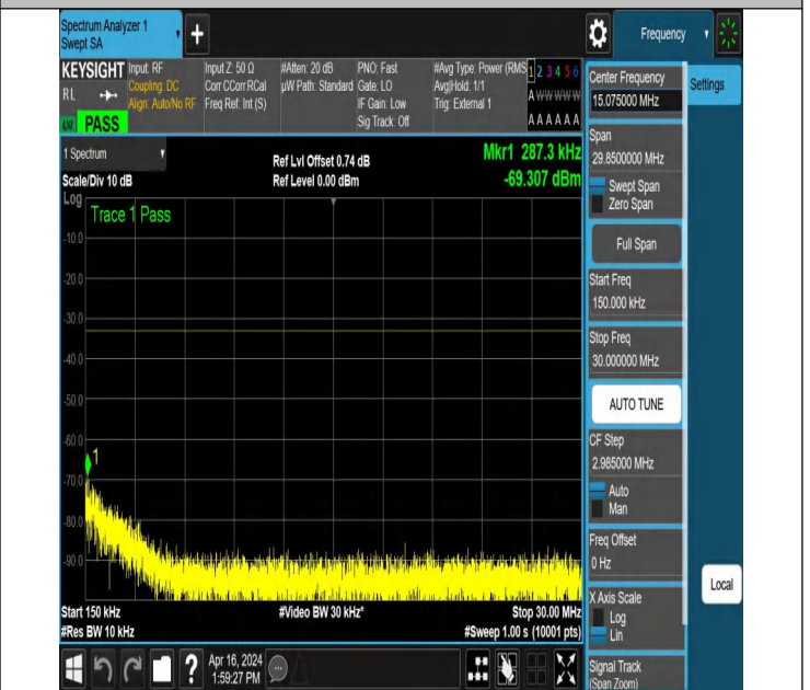
NTNV_N78-3450-3550_PC2_30_30_H_TID5_NS_01_0.15_30_#
