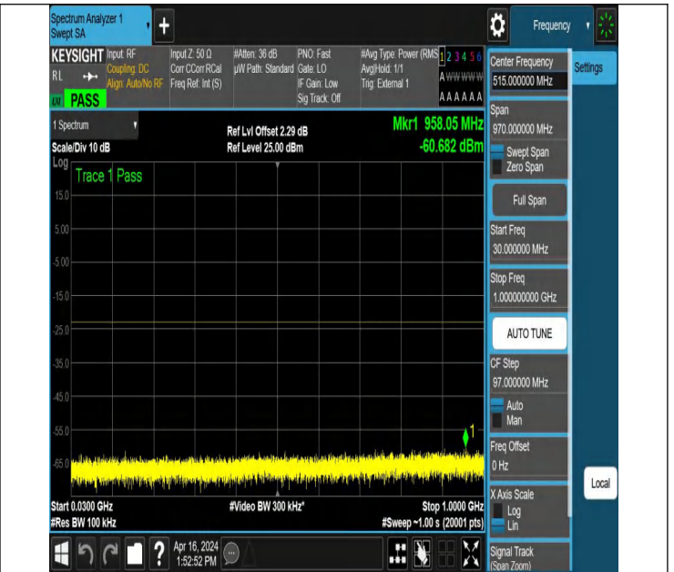
NTNV_N78-3450-3550_PC2_30_30_H_TID3_NS_01_30_1000_#
