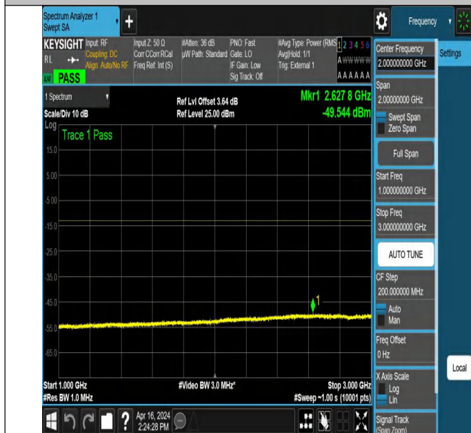
NTNV_N78-3450-3550_PC2_30_40_L_TID3_NS_01_1000_3000
