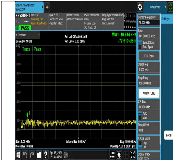
NTNV_N78-3450-3550_PC2_30_40_L_TID2_NS_01_0.009_0.15
