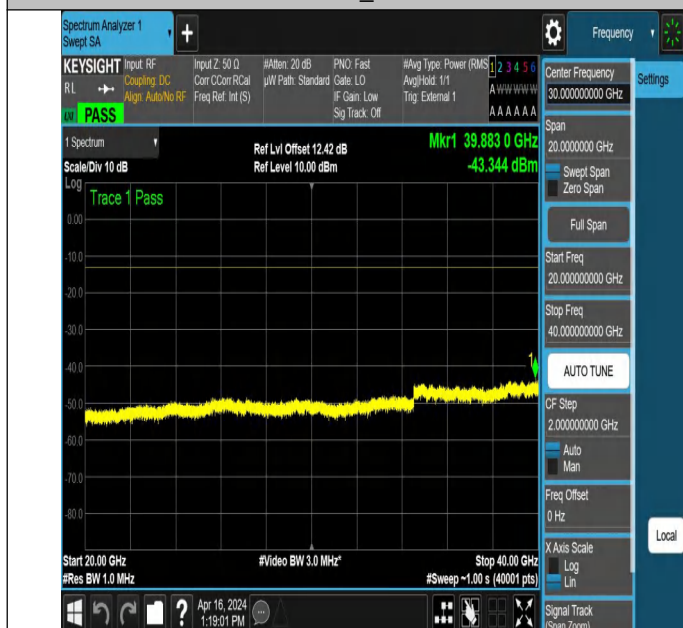
NTNV_N78-3450-3550_PC2_30_30_M_TID2_NS_01_20000_40 000 #1
