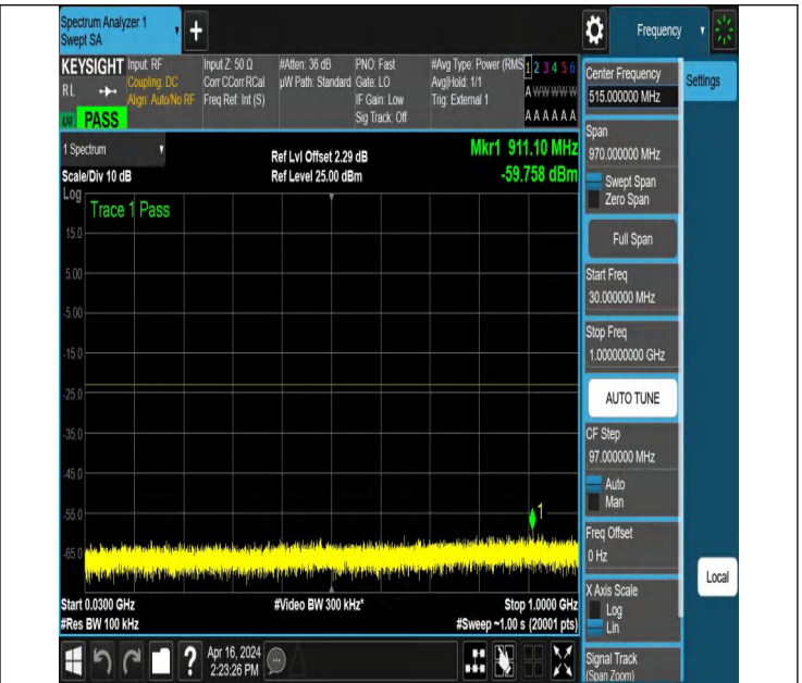
NTNV_N78-3450-3550_PC2_30_40_L_TID3_NS_01_30_1000_#
