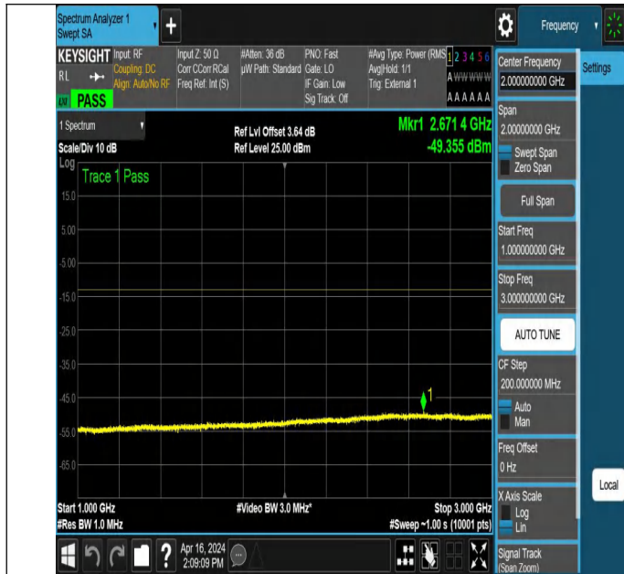
NTNV_N78-3450-3550_PC2_30_30_H_TID6_NS_01_1000_3000
