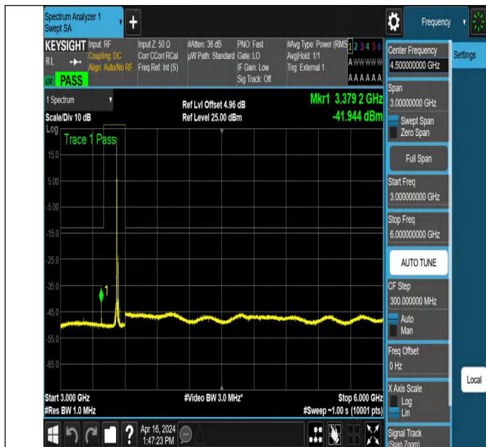
NTNV_N78-3450-3550_PC2_30_30_H_TID2_NS_01_3000_6000
