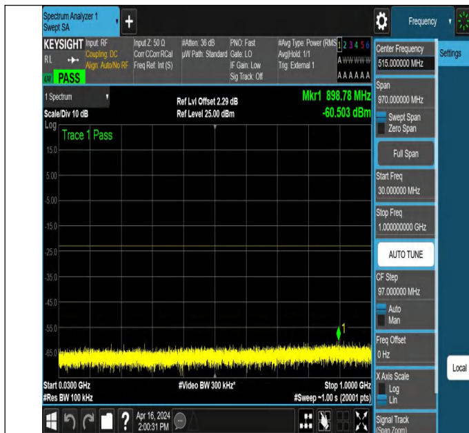
NTNV_N78-3450-3550_PC2_30_30_H_TID5 NS_01_30_1000_#
