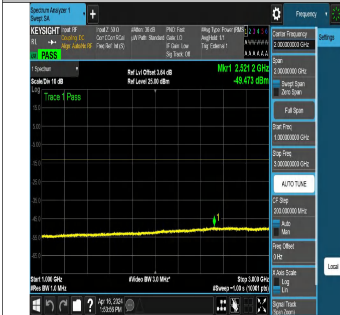
NTNV_N78-3450-3550_PC2_30_30_H_TID3_NS_01_1000_3000
