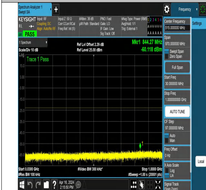
NTNV_N78-3450-3550_PC2_30_40_L_TID2_NS_01_30_1000_#
