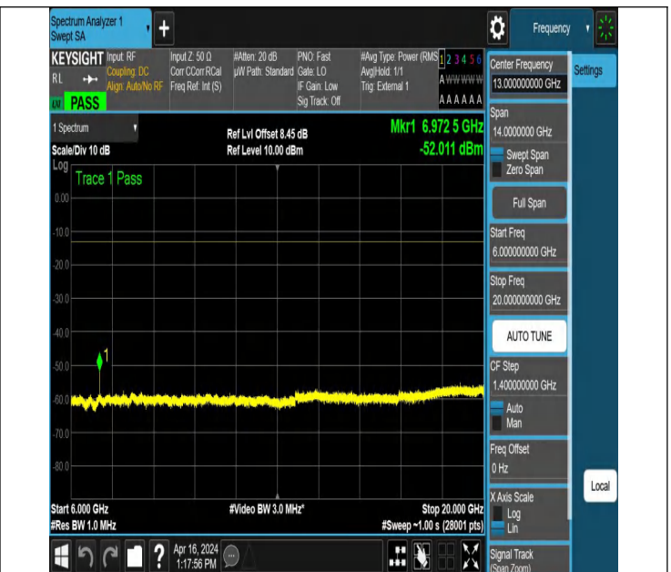
NTNV_N78-3450-3550_PC2_30_30_M_TID2_NS_01_6000_200 00 #1
