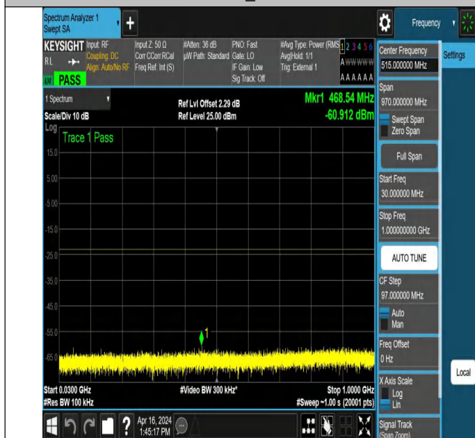
NTNV_N78-3450-3550_PC2_30_30_H_TID2_NS_01_30_1000_#
