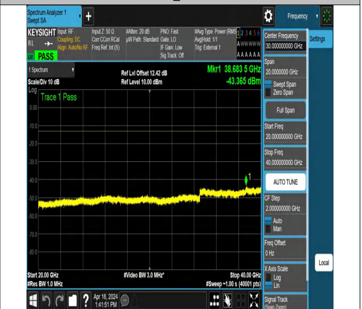
NTNV_N78-3450-3550_PC2_30_30_M_TID6_NS_01_20000_40 000 #1
