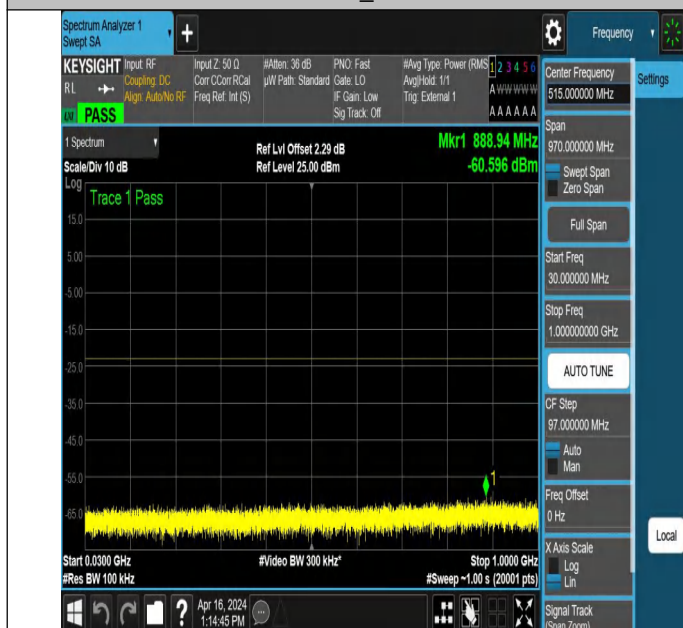
NTNV_N78-3450-3550_PC2_30_30_M_TID2_NS_01_30_1000_#1
