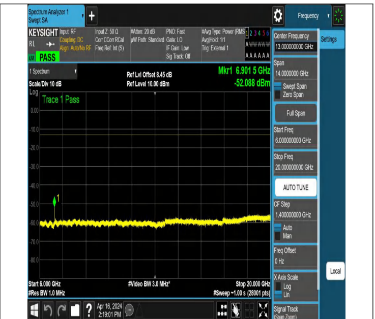
NTNV_N78-3450-3550_PC2_30_40_L_TID2_NS_01_6000_2000
