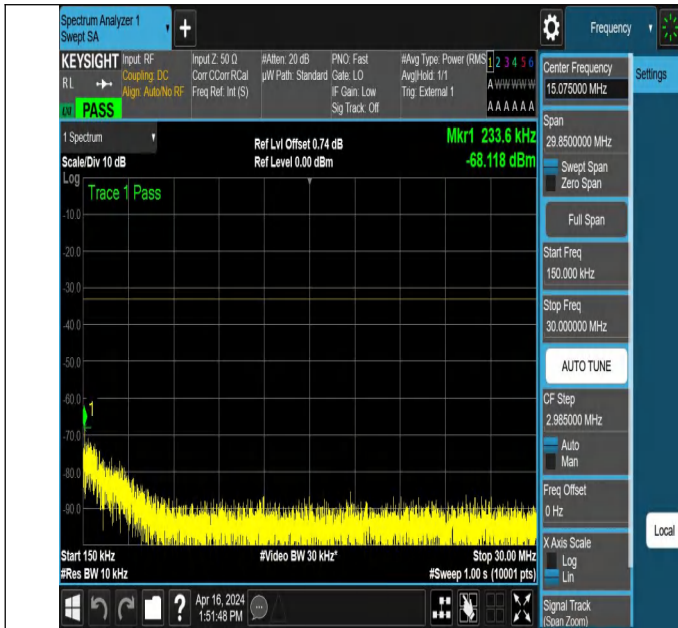
NTNV_N78-3450-3550_PC2_30_30_H_TID3_NS_01_0.15_30_#
