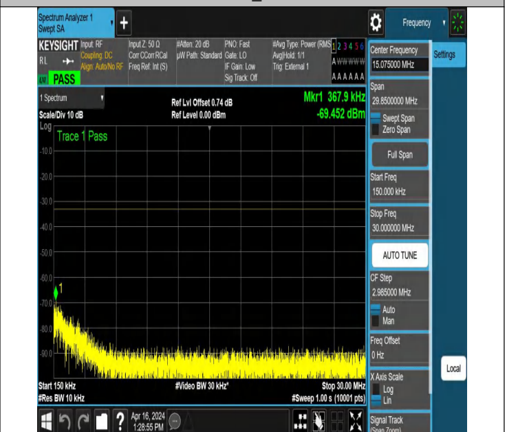
NTNV_N78-3450-3550_PC2_30_30_M_TID5_NS_01_0.15_30_# 1
