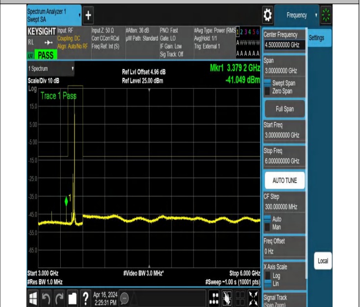
NTNV_N78-3450-3550_PC2_30_40_L_TID3_NS_01_3000_6000
