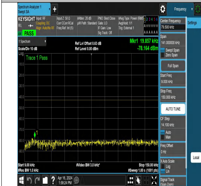
NTNV_N78-3450-3550_PC2_30_30_H_TID5_NS_01_0.009_0.15
