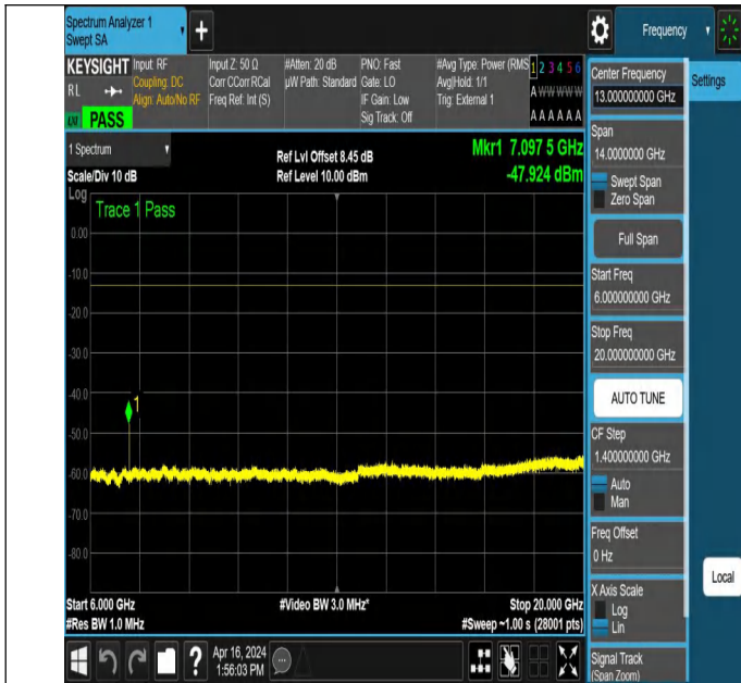
NTNV_N78-3450-3550_PC2_30_30_H_TID3_NS_01_6000_2000
