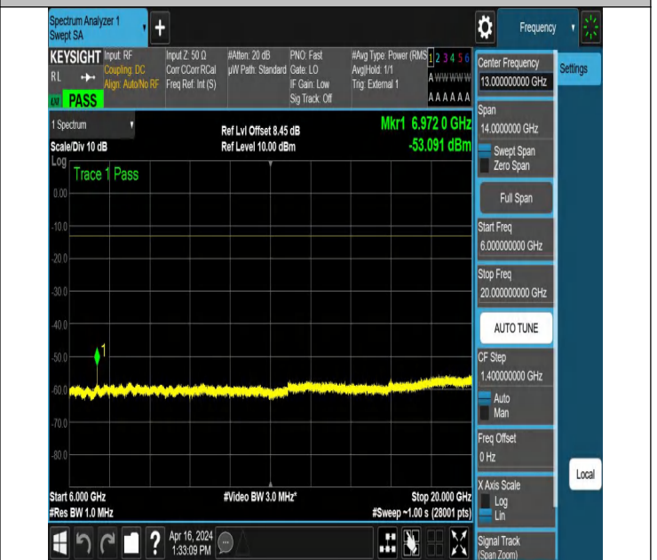
NTNV_N78-3450-3550_PC2_30_30_M_TID5_NS_01_6000_200
