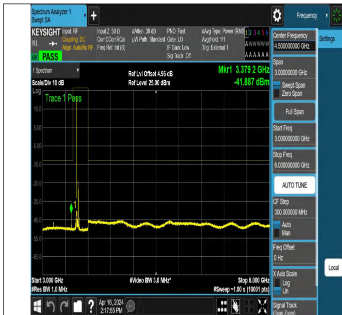
NTNV_N78-3450-3550_PC2_30_40_L_TID2_NS_01_3000_6000
