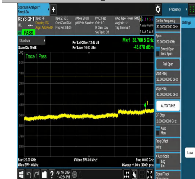
NTNV_N78-3450-3550_PC2_30_30_H_TID2_NS_01_20000_400
