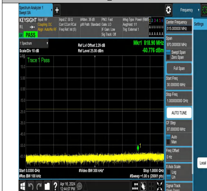
NTNV_N78-3450-3550_PC2_30_30_L_TID2_NS_01_30_1000_#
