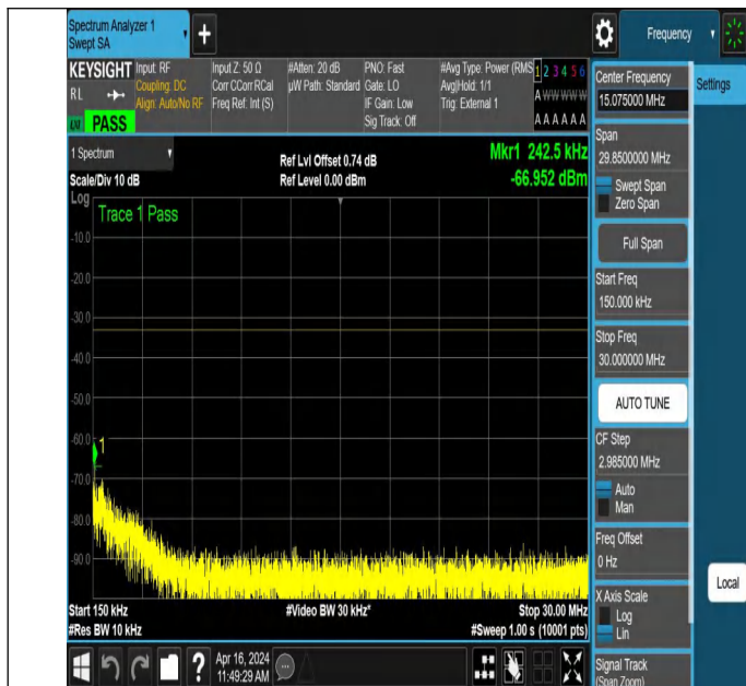
NTNV_N78-3450-3550_PC2_30_20_M_TID3_NS_01_0.15_30_#
