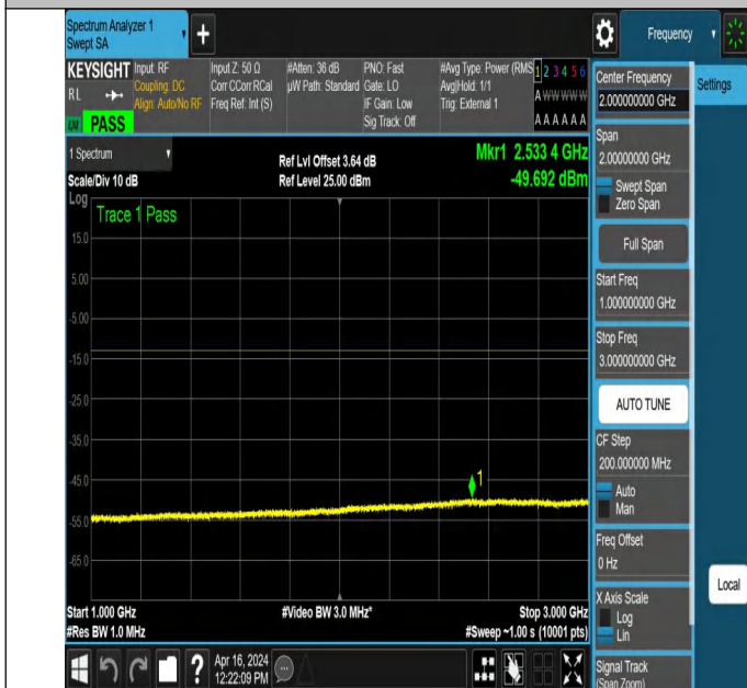
NTNV_N78-3450-3550_PC2_30_20_H_TID3_NS_01_1000_3000
