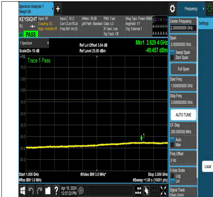
NTNV_N78-3450-3550_PC2_30_20_H_TID6_NS_01_1000_3000
