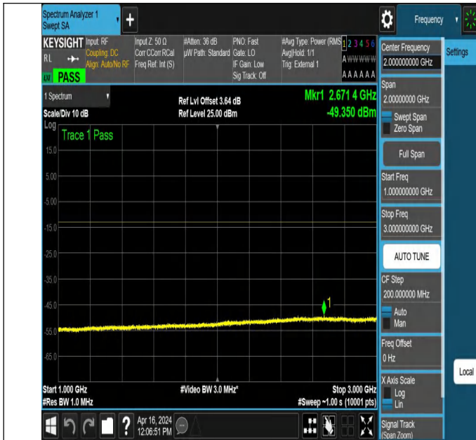
NTNV_N78-3450-3550_PC2_30_20_M_TID6_NS_01_1000_300
