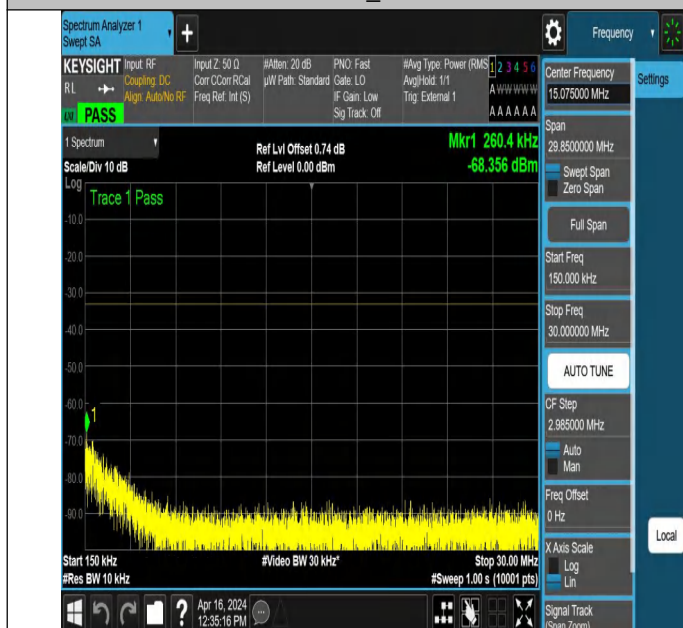
NTNV_N78-3450-3550_PC2_30_20_H_TID6_NS_01_0.15_30_# 1
