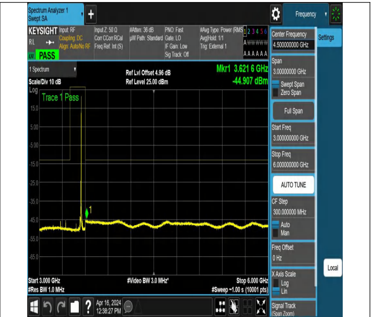
NTNV_N78-3450-3550_PC2_30_20_H_TID6_NS_01_3000_6000
