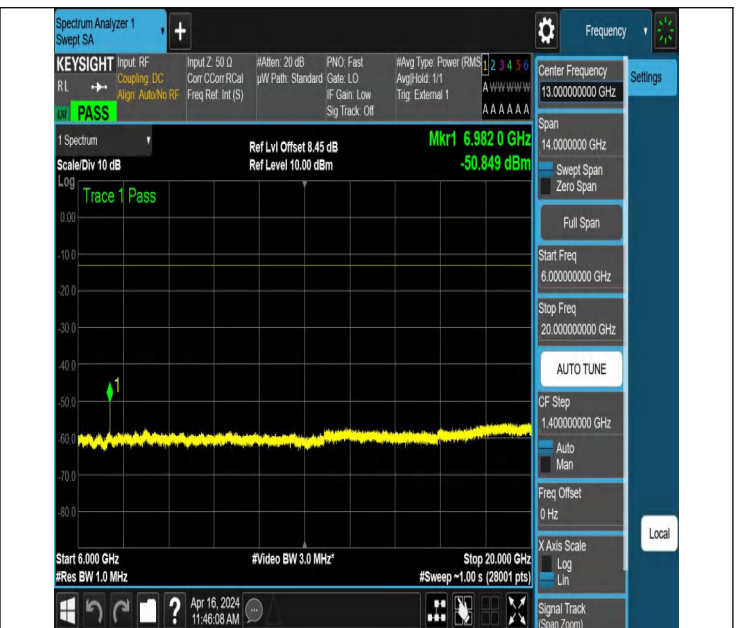
NTNV_N78-3450-3550_PC2_30_20_M_TID2_NS_01_6000_200 00 #1
