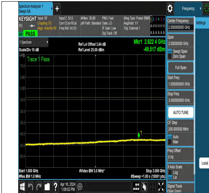
NTNV_N78-3450-3550_PC2_30_30_L_TID6_NS_01_1000_3000
