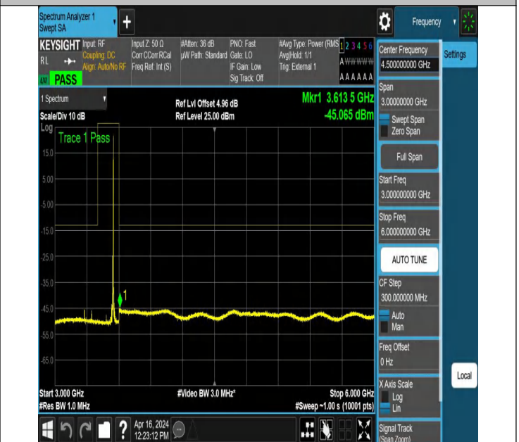
NTNV_N78-3450-3550_PC2_30_20_H_TID3_NS_01_3000_6000
