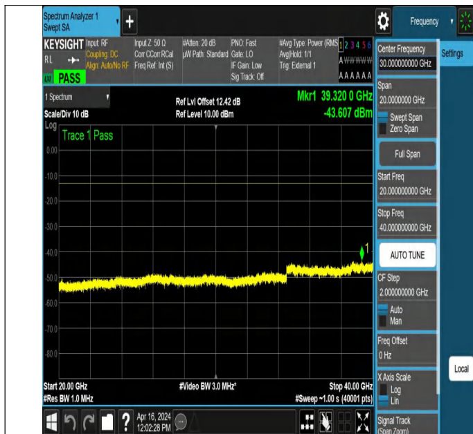
NTNV_N78-3450-3550_PC2_30_20_M_TID5_NS_01_20000_40 000 #1
