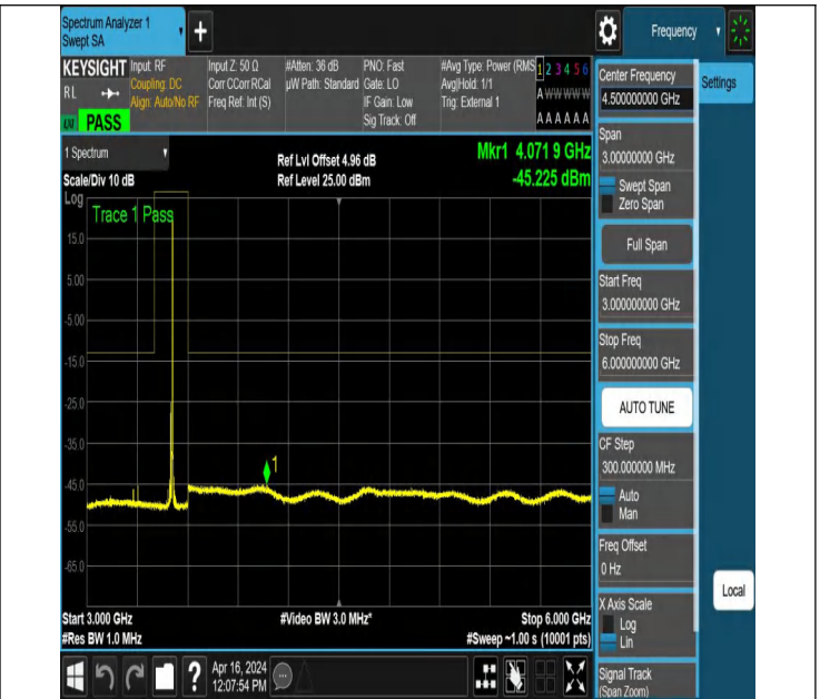
NTNV_N78-3450-3550_PC2_30_20_M_TID6_NS_01_3000_600
