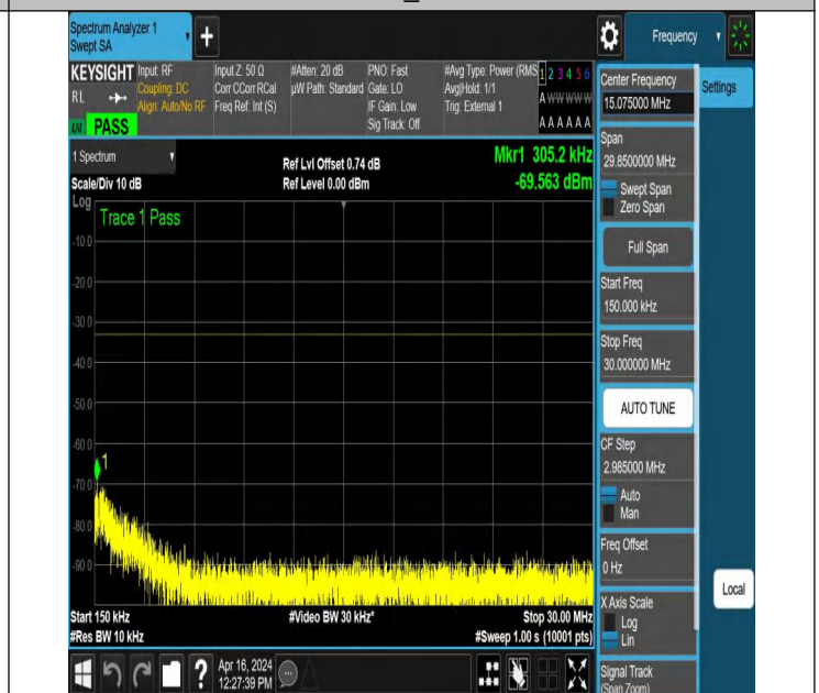
NTNV_N78-3450-3550_PC2_30_20_H_TID5_NS_01_0.15_30_#
