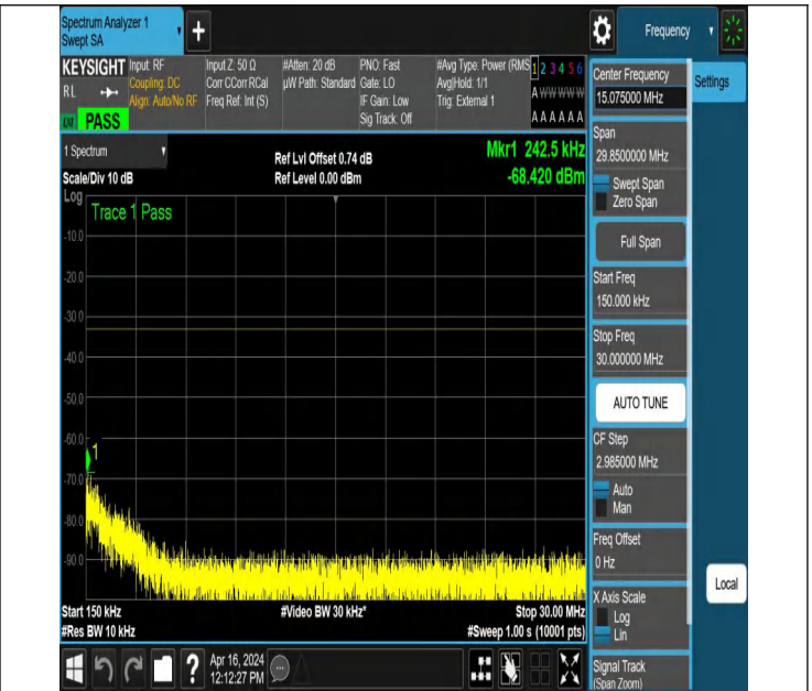
NTNV_N78-3450-3550_PC2_30_20_H_TID2_NS_01_0.15_30_#
