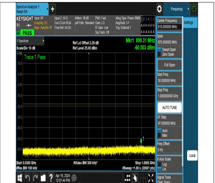
NTNV_N78-3450-3550_PC2_30_30_L_TID3_NS_01_30_1000_#
