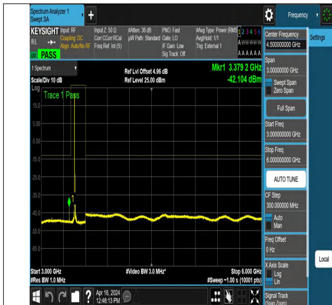
NTNV_N78-3450-3550_PC2_30_30_L_TID2_NS_01_3000_6000
