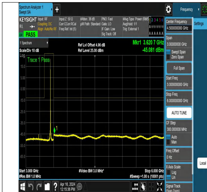
NTNV_N78-3450-3550_PC2_30_20_H_TID2_NS_01_3000_6000
