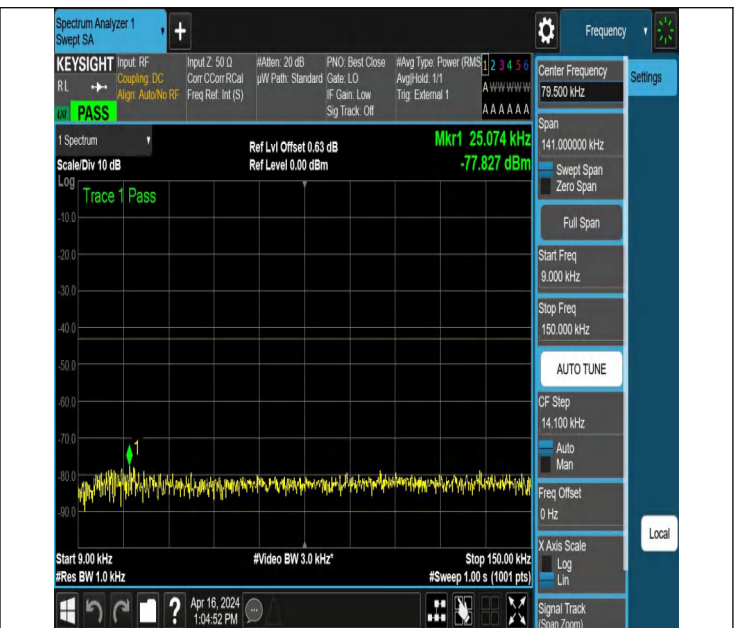
NTNV_N78-3450-3550_PC2_30_30_L_TID6_NS_01_0.009_0.15
