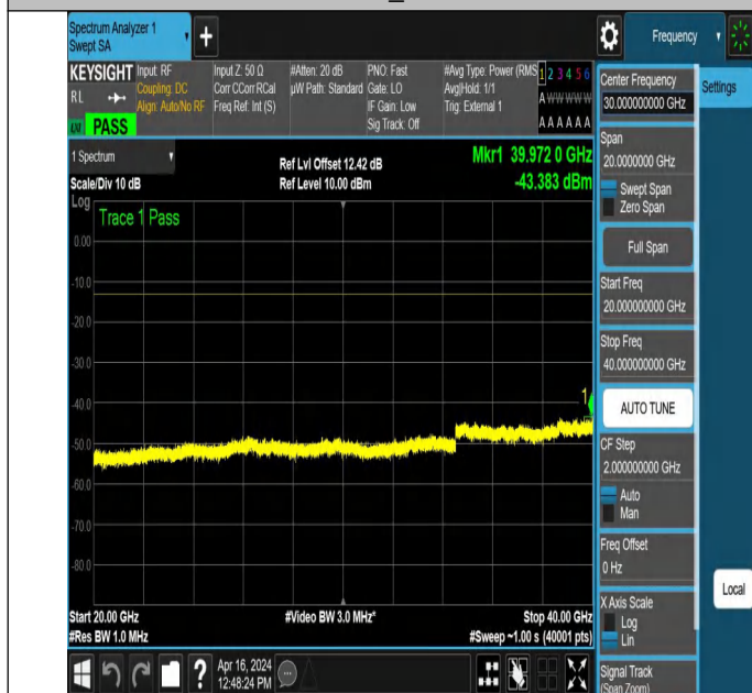
NTNV_N78-3450-3550_PC2_30_30_L_TID2_NS_01_20000_400
