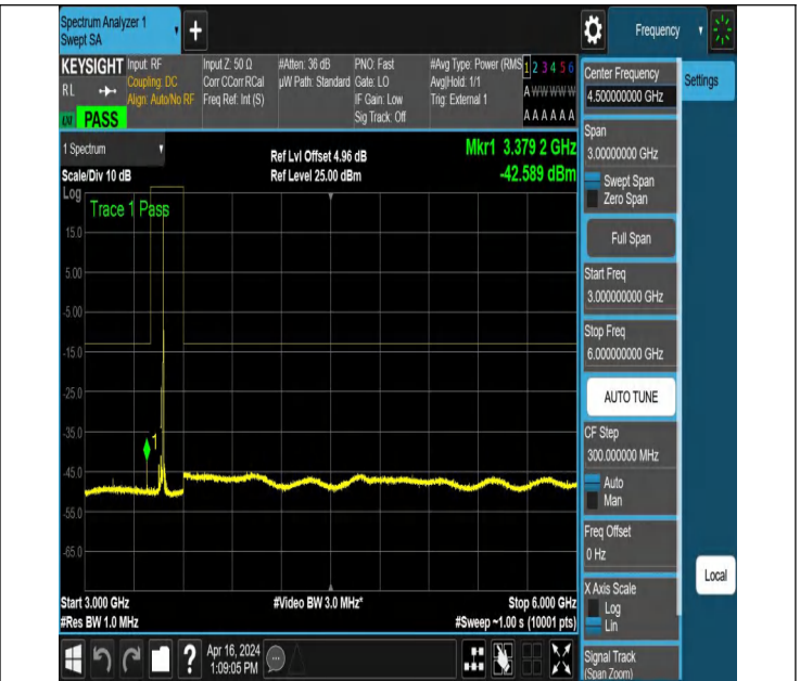
NTNV_N78-3450-3550_PC2_30_30_L_TID6_NS_01_3000_6000
