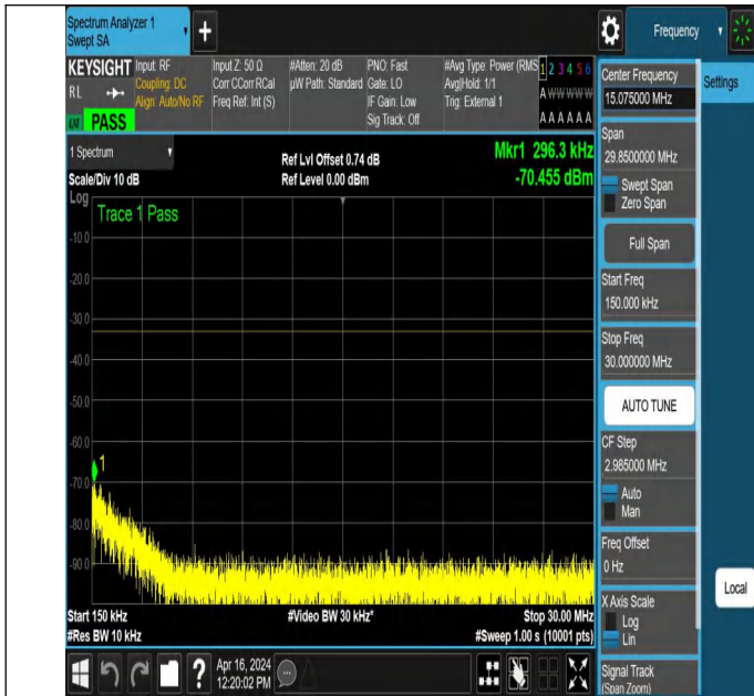
NTNV_N78-3450-3550_PC2_30_20_H_TID3_NS_01_0.15_30_#
