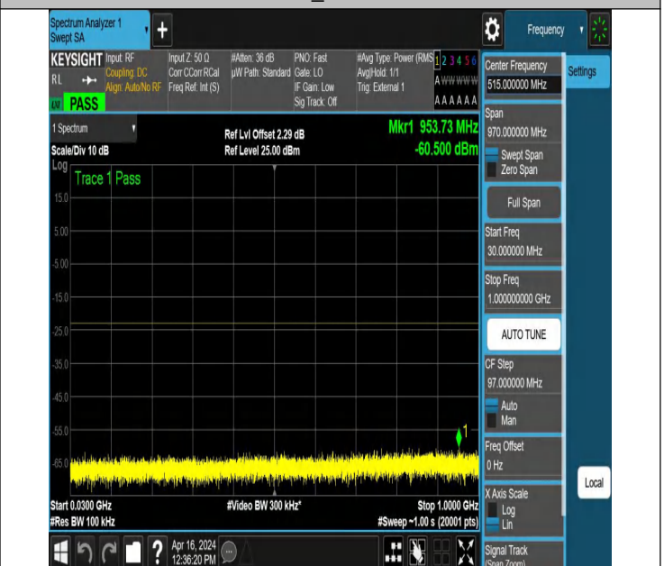
NTNV_N78-3450-3550_PC2_30_20_H_TID6_NS_01_30_1000_# 1
