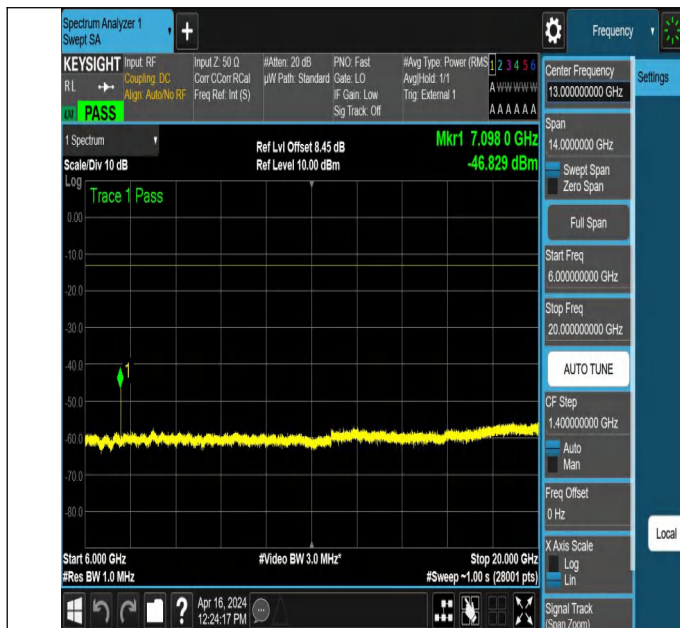
NTNV_N78-3450-3550_PC2_30_20_H_TID3_NS_01_6000_2000
