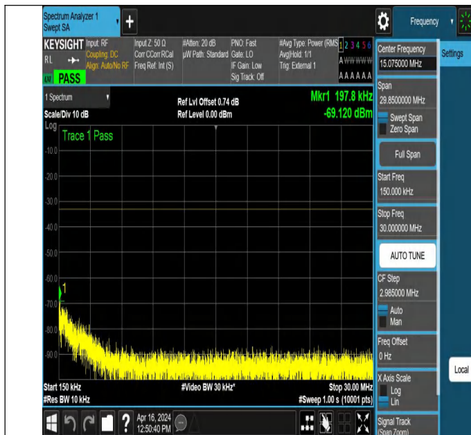
NTNV_N78-3450-3550_PC2_30_30_L_TID3_NS_01_0.15_30_#
