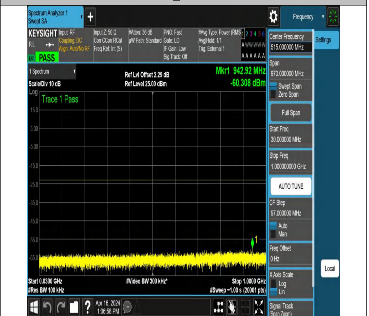
NTNV_N78-3450-3550_PC2_30_30_L_TID6_NS_01_30_1000_#
