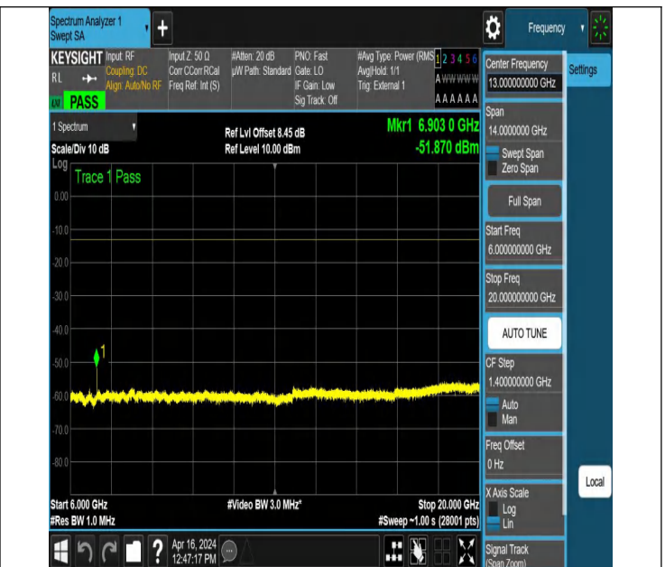
NTNV_N78-3450-3550_PC2_30_30_L_TID2_NS_01_6000_2000
