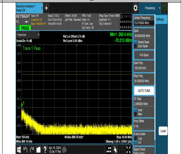
NTNV_N78-3450-3550_PC2_30_30_L_TID5_NS_01_0.15_30_# 1
