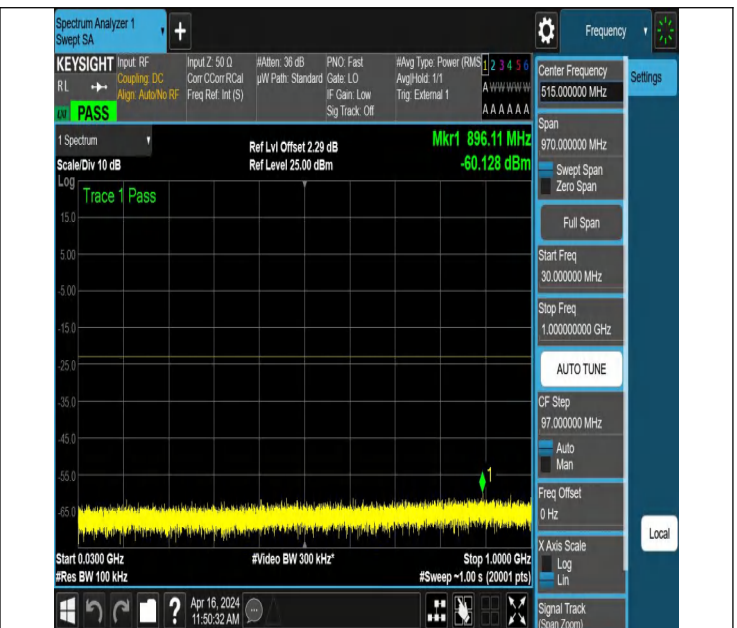
NTNV_N78-3450-3550_PC2_30_20_M_TID3_NS_01_30_1000_
