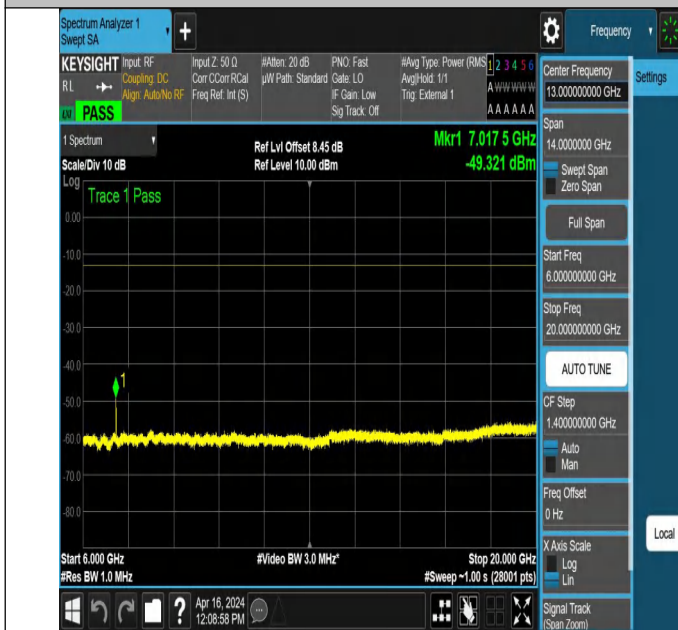
NTNV_N78-3450-3550_PC2_30_20_M_TID6_NS_01_6000_200
