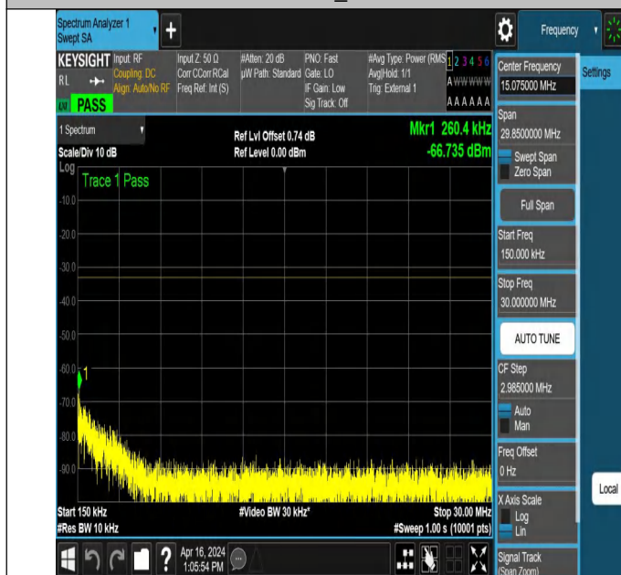
NTNV_N78-3450-3550_PC2_30_30_L_TID6_NS_01_0.15_30_#
