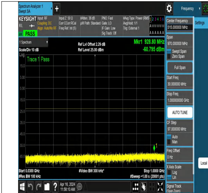
NTNV_N78-3450-3550_PC2_30_20_M_TID5_NS_01_30_1000_
