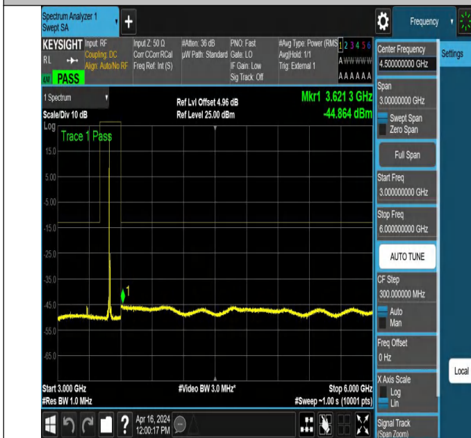
NTNV_N78-3450-3550_PC2_30_20_M_TID5_NS_01_3000_600
