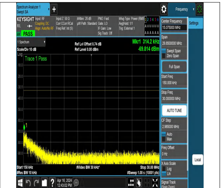
NTNV_N78-3450-3550_PC2_30_30_L_TID2_NS_01_0.15_30_#
