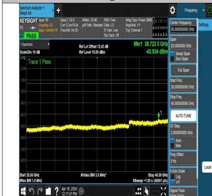
NTNV_N78-3450-3550_PC2_30_20_H_TID2_NS_01_20000_400
