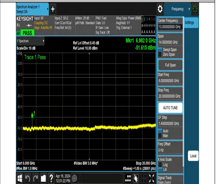
NTNV_N78-3450-3550_PC2_30_20_M_TID5_NS_01_6000_200
