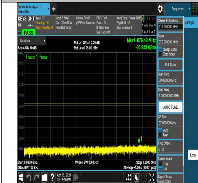
NTNV_N78-3450-3550_PC2_30_20_H_TID2_NS_01_30_1000_#
