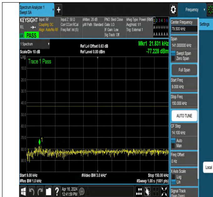
NTNV_N78-3450-3550_PC2_30_30_L_TID2_NS_01_0.009_0.15
