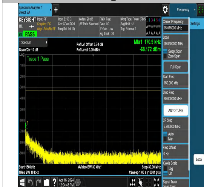
NTNV_N78-3450-3550_PC2_30_20_M_TID6_NS_01_0.15_30_#
