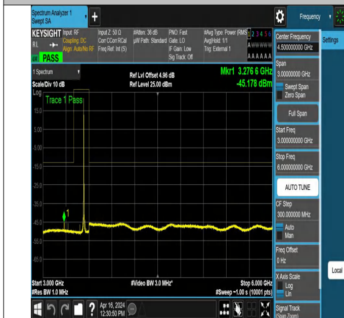
NTNV_N78-3450-3550_PC2_30_20_H_TID5_NS_01_3000_6000
