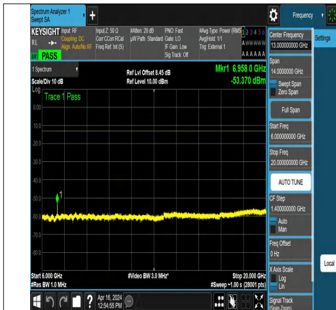
NTNV_N78-3450-3550_PC2_30_30_L_TID3_NS_01_6000_2000
