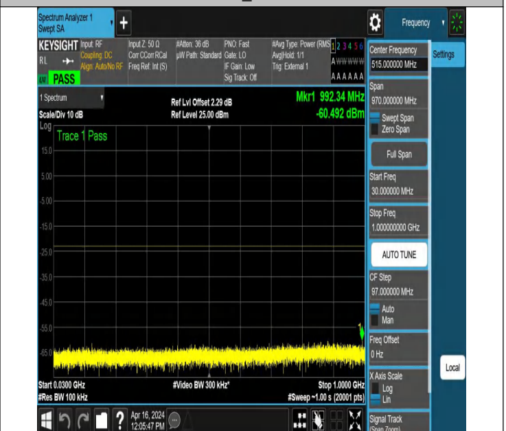
NTNV_N78-3450-3550_PC2_30_20_M_TID6_NS_01_30_1000_ #1
