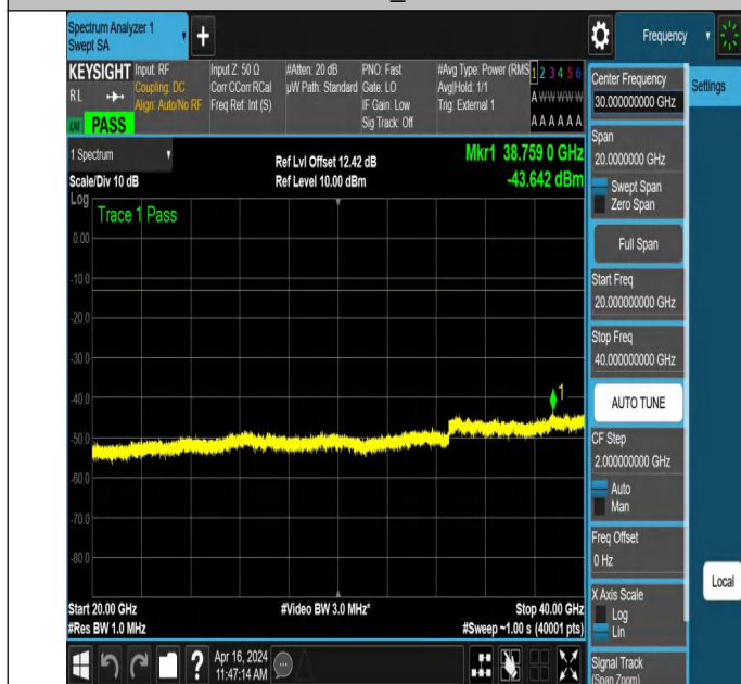
NTNV_N78-3450-3550_PC2_30_20_M_TID2_NS_01_20000_40 000_#1
