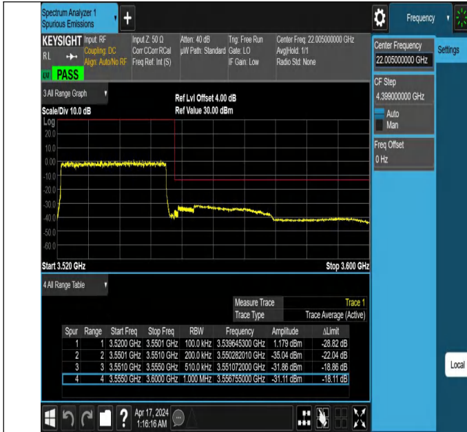
NTNV_N78-3450-3550_PC2_30_30_H_TID1_#1
