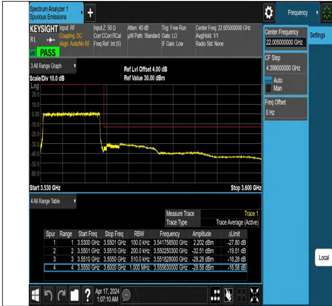
NTNV_N78-3450-3550_PC2_30_20_H_TID1_#1
