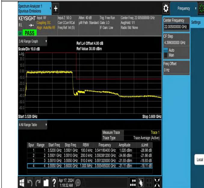
NTNV_N78-3450-3550_PC2_30_30_H_TID4_#1
