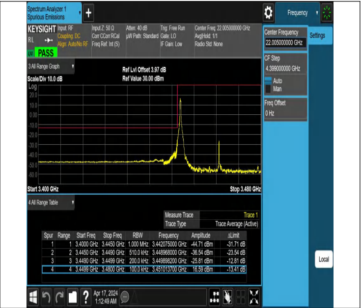
NTNV_N78-3450-3550_PC2_30_30_L_TID2_#1
