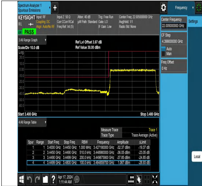
NTNV_N78-3450-3550_PC2_30_30_L_TID1_#1
