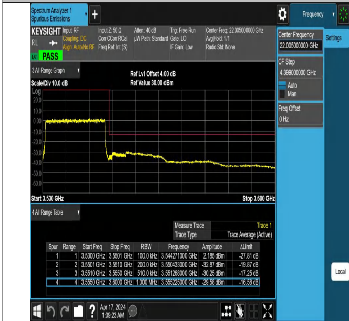
NTNV_N78-3450-3550_PC2_30_20_H_TID4_#1
