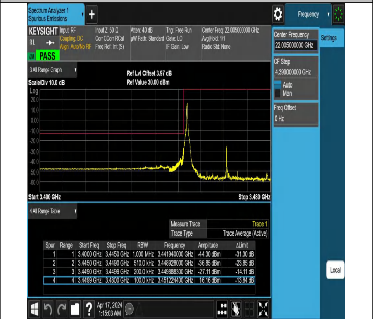
NTNV_N78-3450-3550_PC2_30_30_L_TID5_#1
