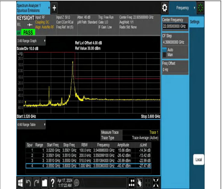
NTNV_N78-3450-3550_PC2_30_30_H_TID3_#1
