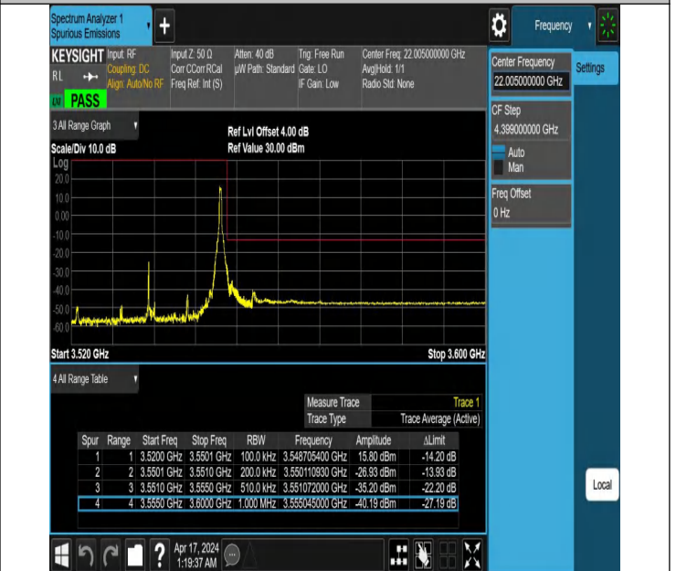
NTNV_N78-3450-3550_PC2_30_30_H_TID6_#1
