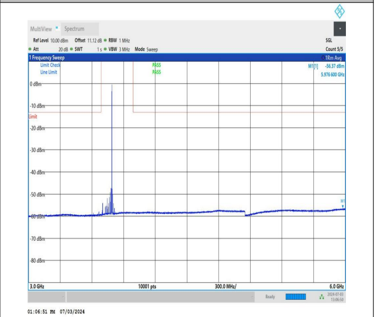
NTNV_DC_26A_n77A-3700-3980_PC2_30_5+90_M+L_TID2_NS_01_3000_6000_#1
