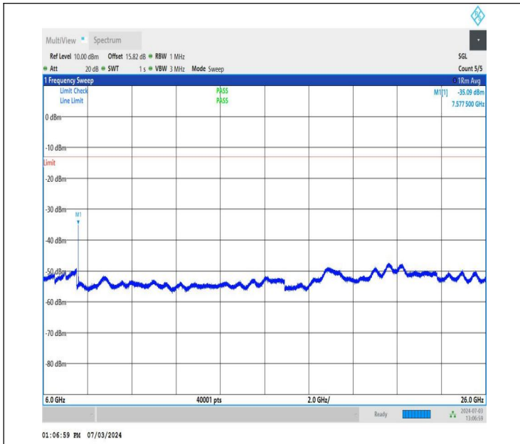
NTNV_DC_26A_n77A-3700-3980_PC2_30_5+90_M+L_TID2_NS_01_6000_26000_#1
