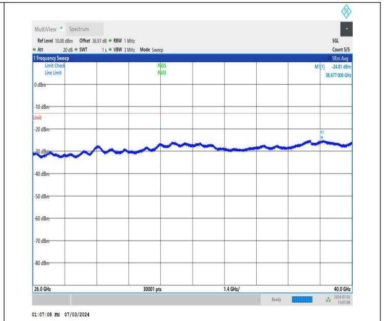
NTNV_DC_26A_n77A-3700-3980_PC2_30_5+90_M+L_TID2_NS_01_26000_40000_#1
