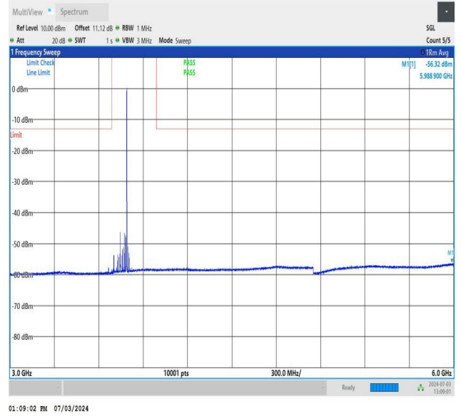
NTNV_DC_26A_n77A-3700-3980_PC2_30_5+90_M+L_TID5_NS_01_3000_6000_#1
