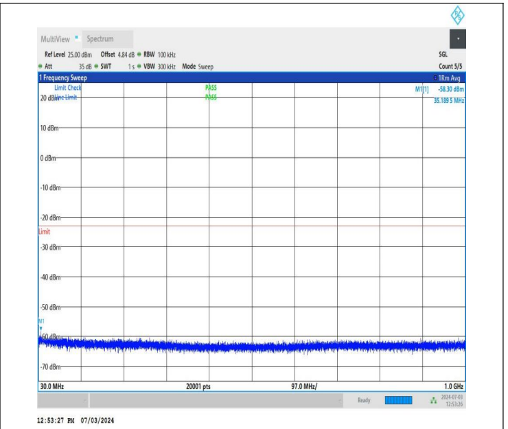
NTNV_DC_26A_n77A-3700-3980_PC2_30_5+80_M+L_TID2_NS_01_30_1000_#1
