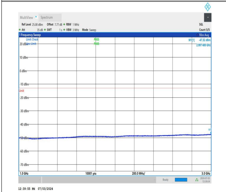
NTNV_DC_26A_n77A-3700-3980_PC2_30_5+60_M+L_TID2_NS_01_1000_3000_#1
