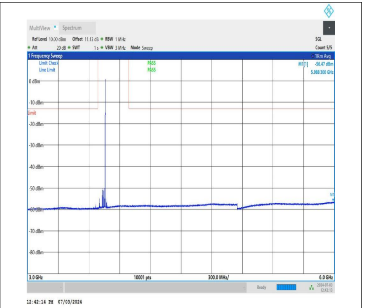
NTNV_DC_26A_n77A-3700-3980_PC2_30_5+60_M+L_TID5_NS_01_3000_6000_#1
