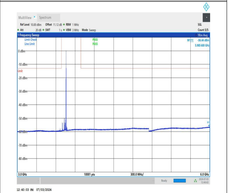
NTNV_DC_26A_n77A-3700-3980_PC2_30_5+60_M+L_TID2_NS_01_3000_6000_#1
