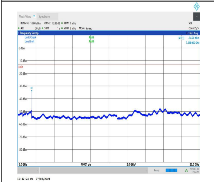
NTNV_DC_26A_n77A-3700-3980_PC2_30_5+60_M+L_TID5_NS_01_6000_26000_#1
