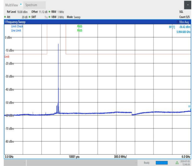
NTNV_DC_26A_n77A-3700-3980_PC2_30_5+60_M+M_TID5_N S_01_3000_6000_#1
