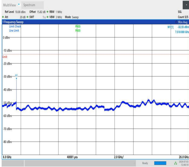
NTNV_DC_26A_n77A-3700-3980_PC2_30_5+60_M+L_TID2_NS_01_6000_26000_#1
