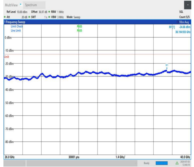
NTNV_DC_26A_n77A-3700-3980_PC2_30_5+60_M+L_TID2_NS_01_26000_40000_#1
