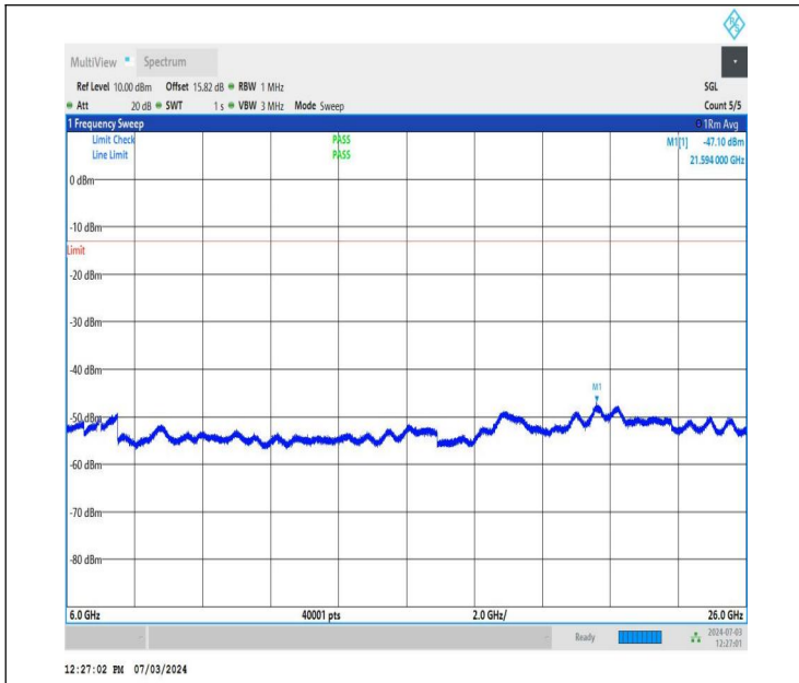
NTNV_DC_26A_n77A-3700-3980_PC2_30_5+50_M+L_TID2_NS_01_6000_26000_#1
