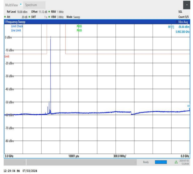
NTNV_DC_26A_n77A-3700-3980_PC2_30_5+50_M+L_TID5_NS_01_3000_6000_#1
