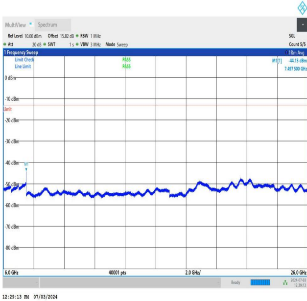
NTNV_DC_26A_n77A-3700-3980_PC2_30_5+50_M+L_TID5_NS_01_6000_26000_#1
