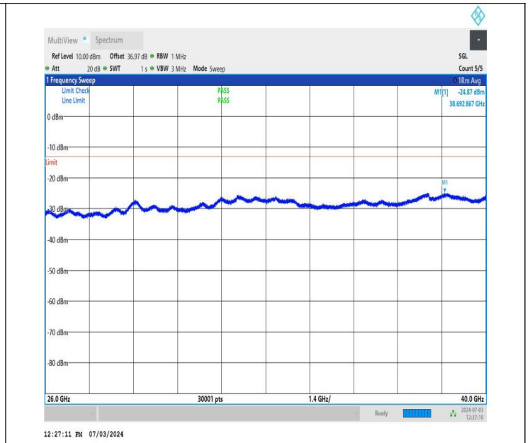
NTNV_DC_26A_n77A-3700-3980_PC2_30_5+50_M+L_TID2_NS_01_26000_40000_#1
