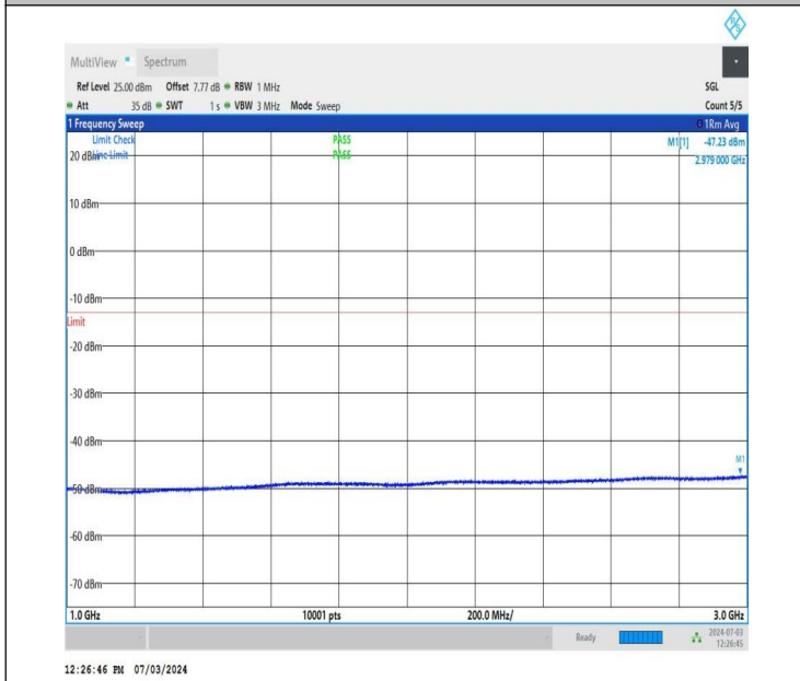
NTNV_DC_26A_n77A-3700-3980_PC2_30_5+50_M+L_TID2_NS_01_1000_3000_#1
