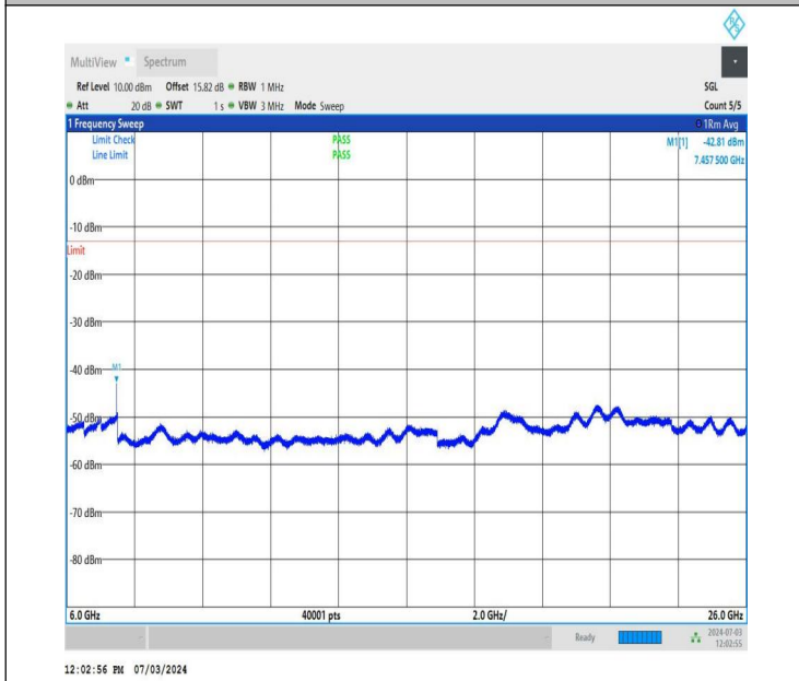
NTNV_DC_26A_n77A-3700-3980_PC2_30_5+30_M+L_TID5_NS_01_6000_26000_#1
