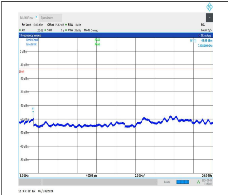
NTNV_DC_26A_n77A-3700-3980_PC2_30_5+20_M+L_TID2_NS_01_6000_26000_#1
