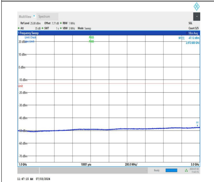
NTNV_DC_26A_n77A-3700-3980_PC2_30_5+20_M+L_TID2_NS_01_1000_3000_#1
