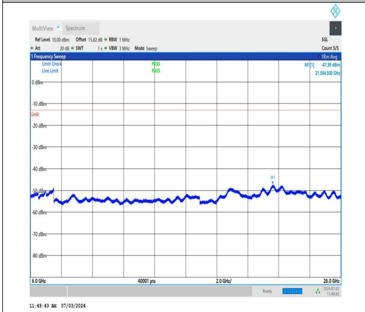
NTNV_DC_26A_n77A-3700-3980_PC2_30_5+20_M+L_TID5_NS_01_6000_26000_#1
