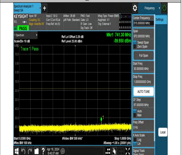
NTNV_N77-3700-3980_PC2_30_90_H_TID6_NS_01_30_1000_# 1
