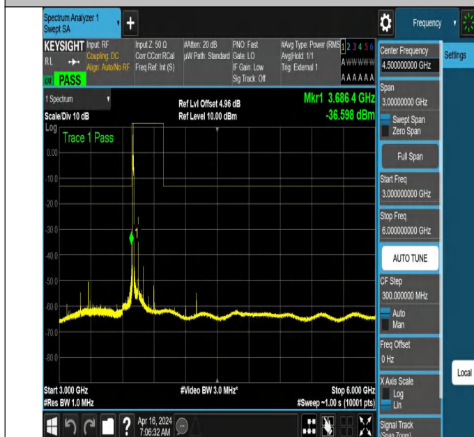
NTNV_N77-3700-3980_PC2_30_100_L_TID5_NS_01_3000_600
