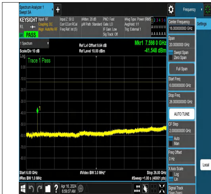
NTNV_N77-3700-3980_PC2_30_100_L_TID3_NS_01_6000_260
