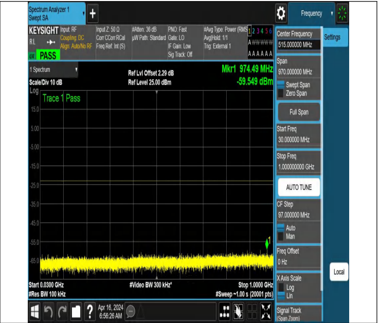
NTNV_N77-3700-3980_PC2_30_100_L_TID3_NS_01_30_1000_
