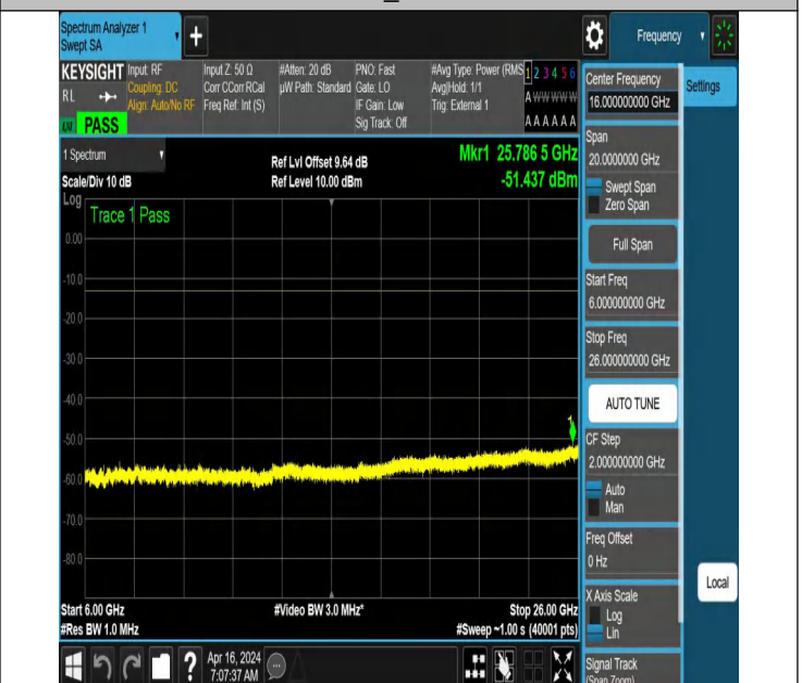
NTNV_N77-3700-3980_PC2_30_100_L_TID5_NS_01_6000_260 00 #1
