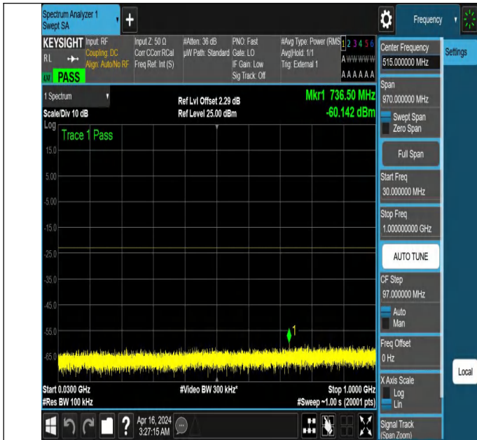
NTNV_N77-3700-3980_PC2_30_60_H_TID5_NS_01_30_1000_#
