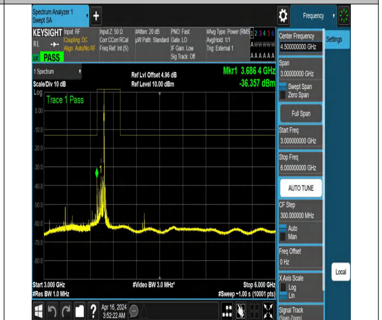
NTNV_N77-3700-3980_PC2_30_80_L_TID3_NS_01_3000_6000
