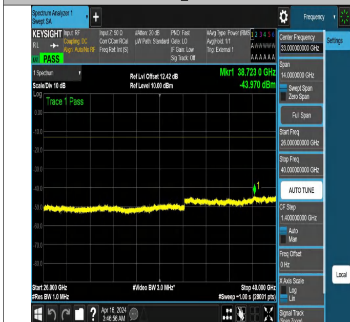
NTNV_N77-3700-3980_PC2_30_80_L_TID2_NS_01_26000_400
