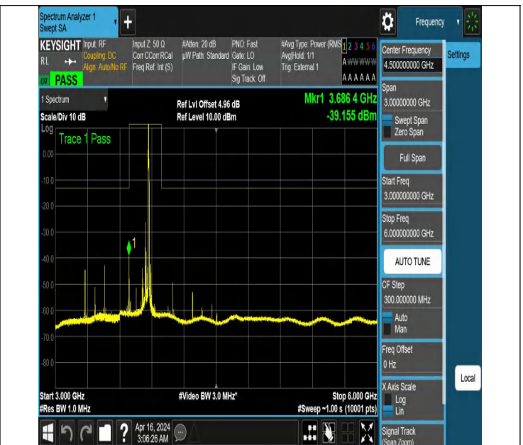
NTNV_N77-3700-3980_PC2_30_60_M_TID6_NS_01_3000_600
