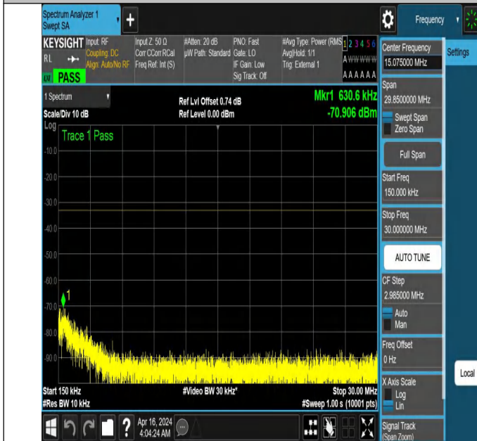
NTNV_N77-3700-3980_PC2_30_80_L_TID6_NS_01_0.15_30_#
