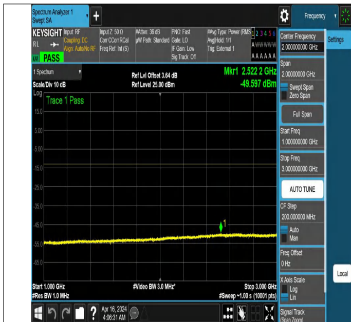
NTNV_N77-3700-3980_PC2_30_80_L_TID6 NS_01_1000_3000
