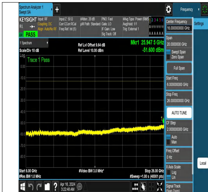
NTNV_N77-3700-3980_PC2_30_60_H_TID3_NS_01_6000_2600
