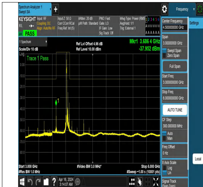
NTNV_N77-3700-3980_PC2_30_60_H_TID2_NS_01_3000_6000
