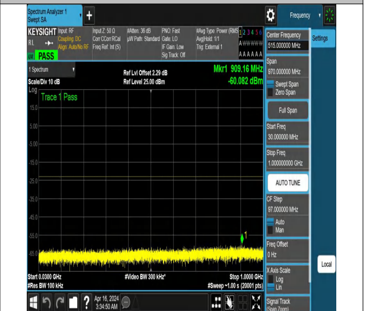
NTNV_N77-3700-3980_PC2_30_60_H_TID6_NS_01_30_1000_#
