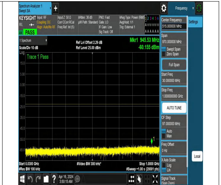
NTNV_N77-3700-3980_PC2_30_80_L_TID3_NS_01_30_1000_#
