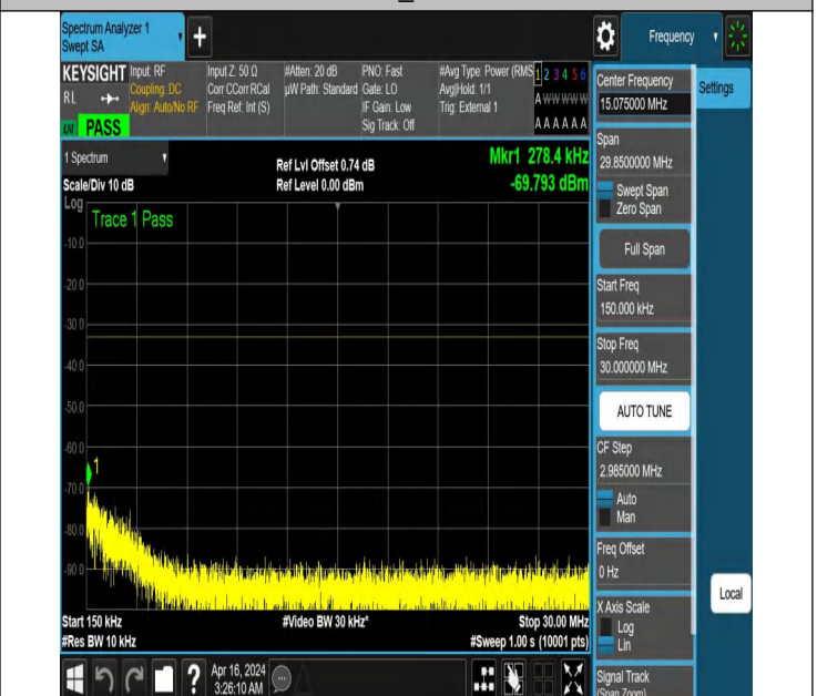
NTNV_N77-3700-3980_PC2_30_60_H_TID5_NS_01_0.15_30_# 1
