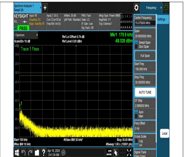
NTNV_N77-3700-3980_PC2_30_80_L_TID2_NS_01_0.15_30_#
