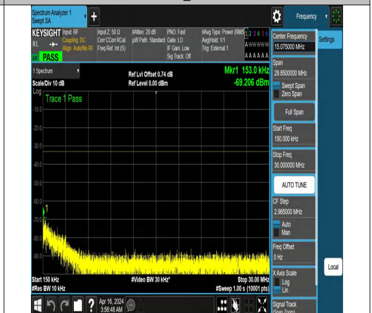
NTNV_N77-3700-3980_PC2_30_80_L_TID5_NS_01_0.15_30_#
