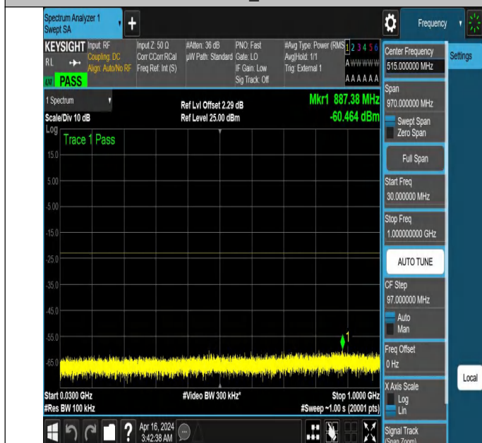
NTNV_N77-3700-3980_PC2_30_80_L_TID2_NS_01_30_1000_#
