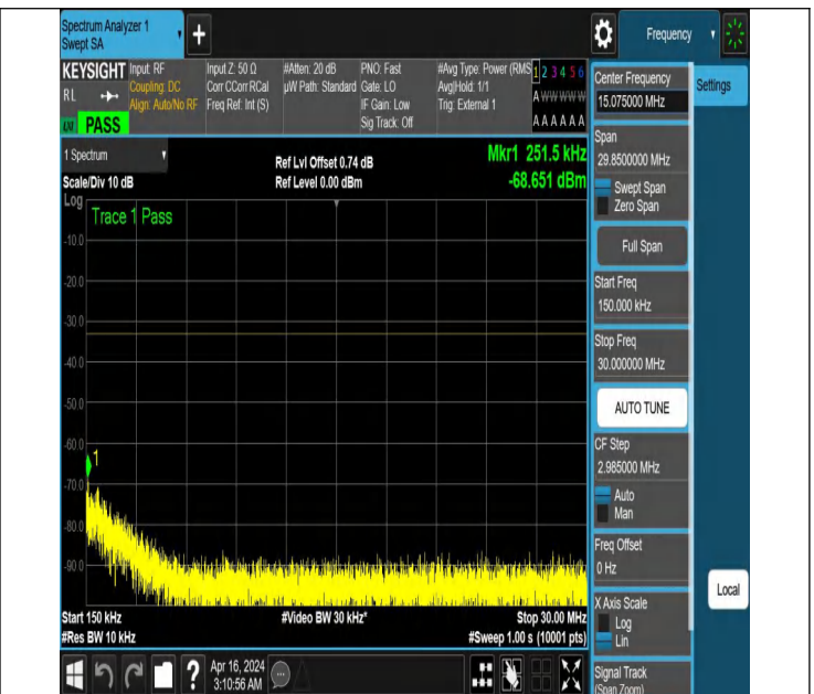
NTNV_N77-3700-3980_PC2_30_60_H_TID2_NS_01_0.15_30_#
