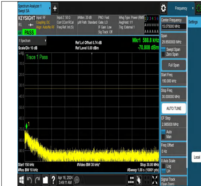
NTNV_N77-3700-3980_PC2_30_80_L_TID3_NS_01_0.15_30_#
