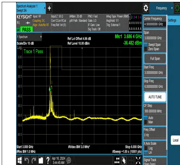
NTNV_N77-3700-3980_PC2_30_80_L_TID2_NS_01_3000_6000
