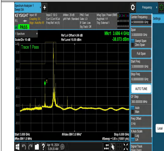
NTNV_N77-3700-3980_PC2_30_60_H_TID5_NS_01_3000_6000
