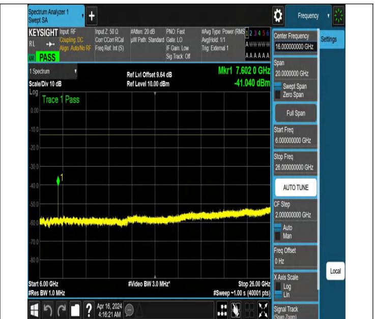
NTNV_N77-3700-3980_PC2_30_80_M_TID2_NS_01_6000_260
