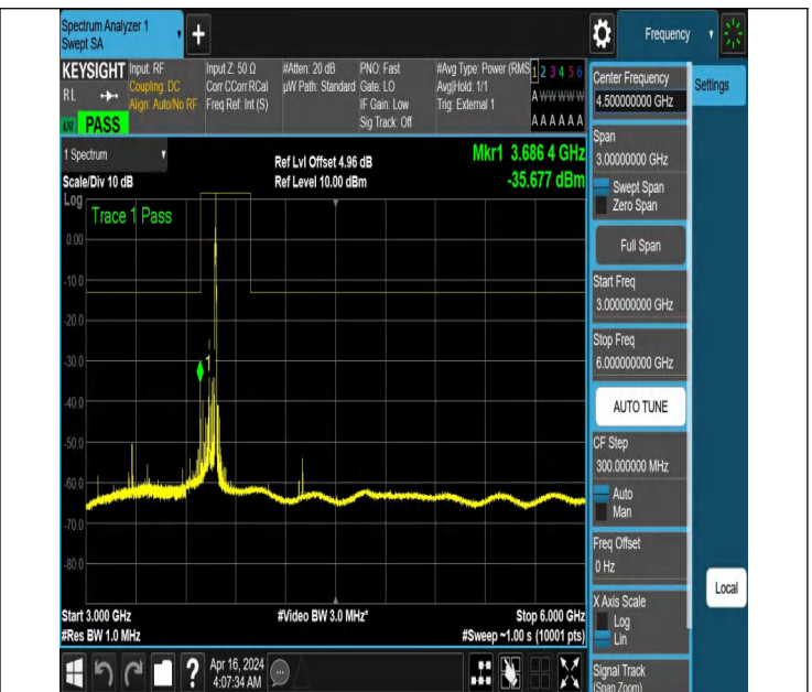
NTNV_N77-3700-3980_PC2_30_80_L_TID6_NS_01_3000_6000
