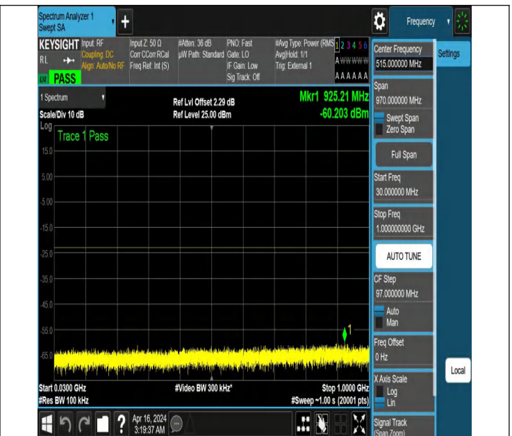
NTNV_N77-3700-3980_PC2_30_60_H_TID3_NS_01_30_1000_#
