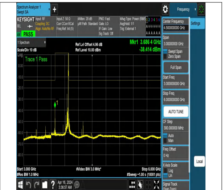
NTNV_N77-3700-3980_PC2_30_60_H_TID6_NS_01_3000_6000
