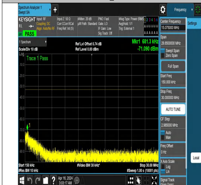
NTNV_N77-3700-3980_PC2_30_60_M_TID6_NS_01_0.15_30_#
