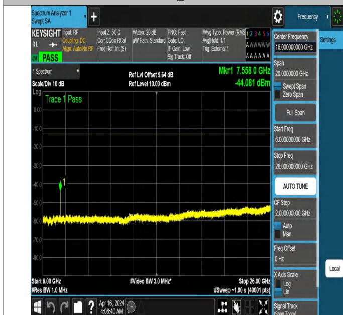
NTNV_N77-3700-3980_PC2_30_80_L_TID6_NS_01_6000_2600
