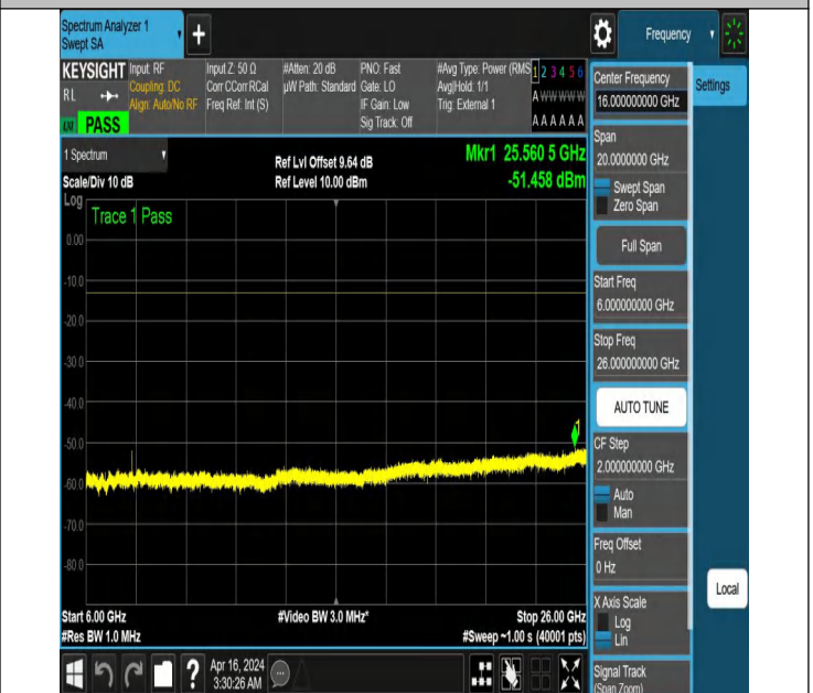
NTNV_N77-3700-3980_PC2_30_60_H_TID5_NS_01_6000_2600
