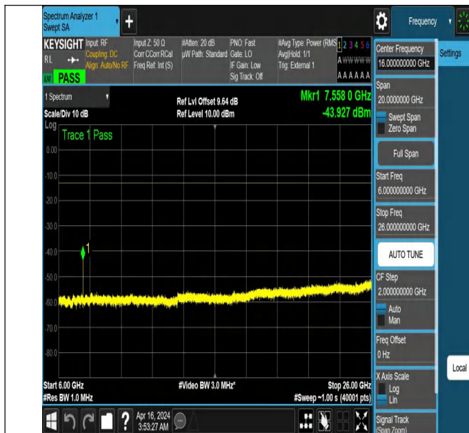
NTNV_N77-3700-3980_PC2_30_80_L_TID3_NS_01_6000_2600
