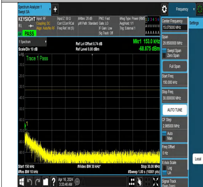
NTNV_N77-3700-3980_PC2_30_60_H_TID6_NS_01_0.15_30_#
