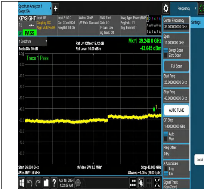
NTNV_N77-3700-3980_PC2_30_80_L_TID5_NS_01_26000_400
