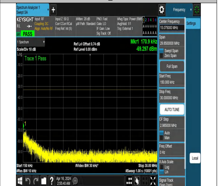
NTNV_N77-3700-3980_PC2_30_60_M_TID5_NS_01_0.15_30_#
