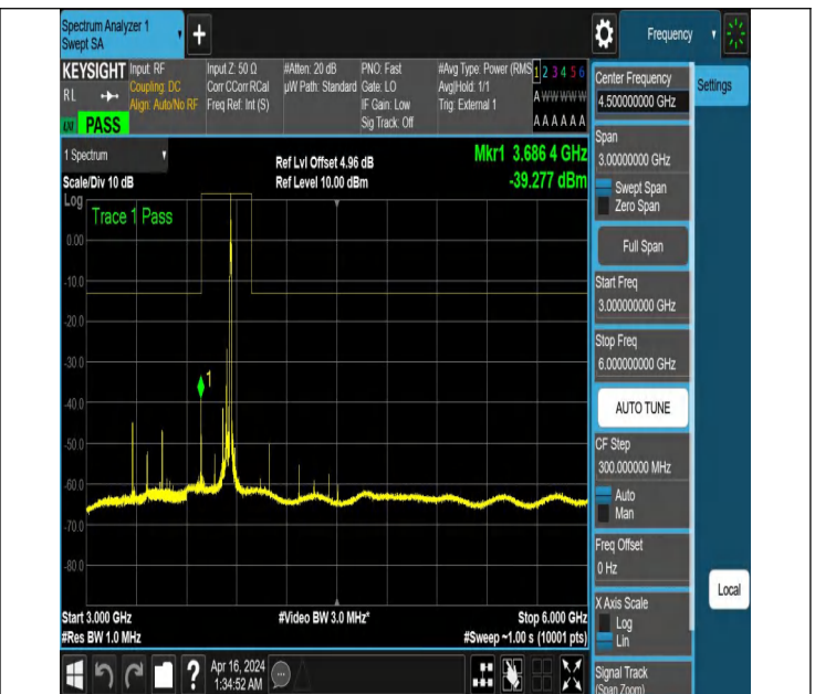
NTNV_N77-3700-3980_PC2_30_50_M_TID6_NS_01_3000_600
