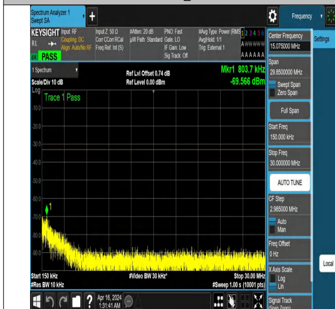
NTNV_N77-3700-3980_PC2_30_50_M_TID6_NS_01_0.15_30_#
