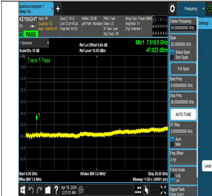
NTNV_N77-3700-3980_PC2_30_60_L_TID6_NS_01_6000_2600
