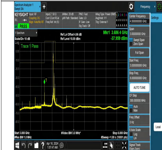
NTNV_N77-3700-3980_PC2_30_50_H_TID5_NS_01_3000_6000
