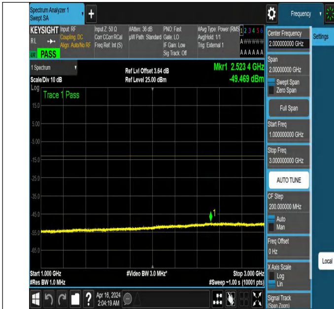
NTNV_N77-3700-3980_PC2_30_50_H_TID6_NS_01_1000_3000
