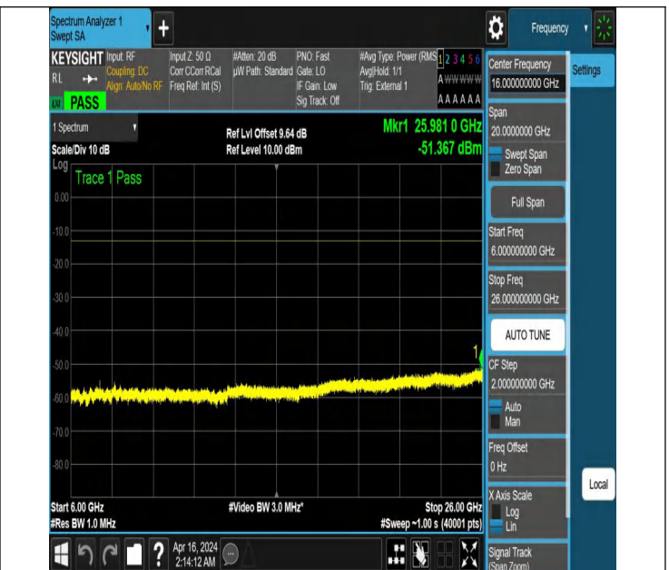
NTNV_N77-3700-3980_PC2_30_60_L_TID2_NS_01_6000_2600
