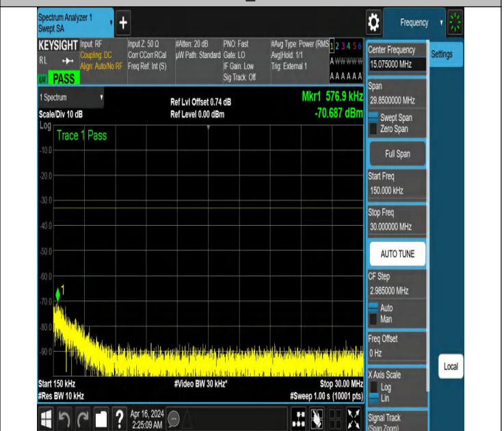
NTNV_N77-3700-3980_PC2_30_60_L_TID5_NS_01_0.15_30_#
