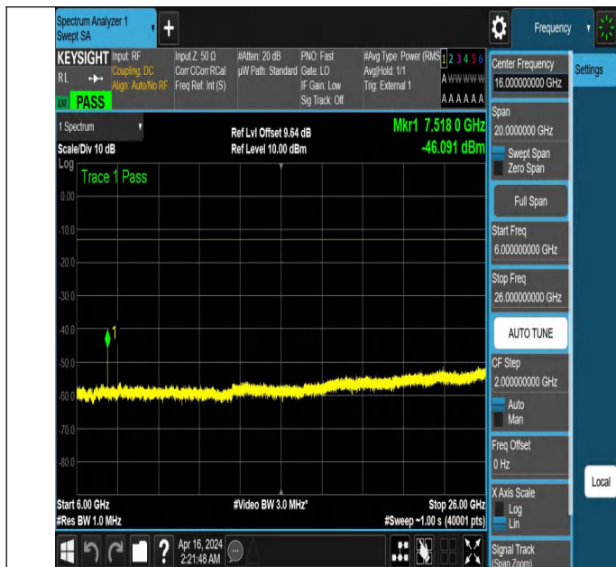
NTNV_N77-3700-3980_PC2_30_60_L_TID3_NS_01_6000_2600
