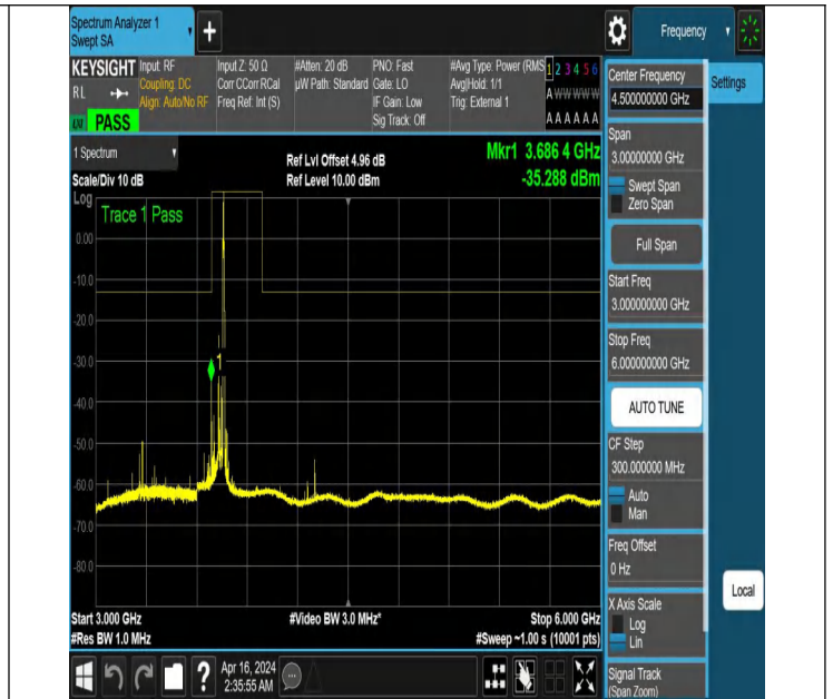
NTNV_N77-3700-3980_PC2_30_60_L_TID6_NS_01_3000_6000
