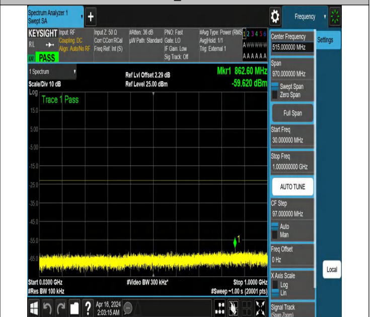
NTNV_N77-3700-3980_PC2_30_50_H_TID6_NS_01_30_1000_#
