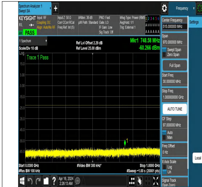
NTNV_N77-3700-3980_PC2_30_60_L_TID5_NS_01_30_1000_#
