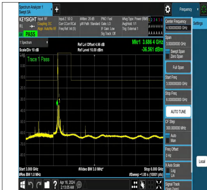
NTNV_N77-3700-3980_PC2_30_60_L_TID2_NS_01_3000_6000
