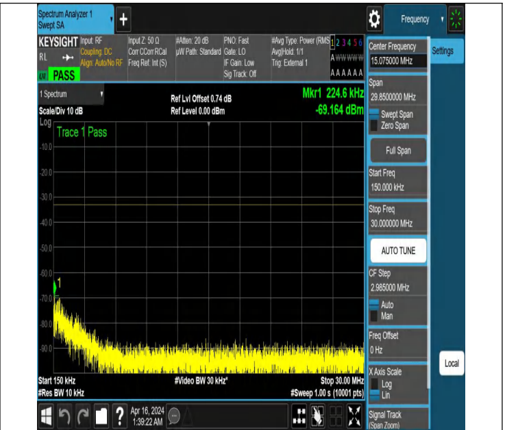
NTNV_N77-3700-3980_PC2_30_50_H_TID2_NS_01_0.15_30_#
