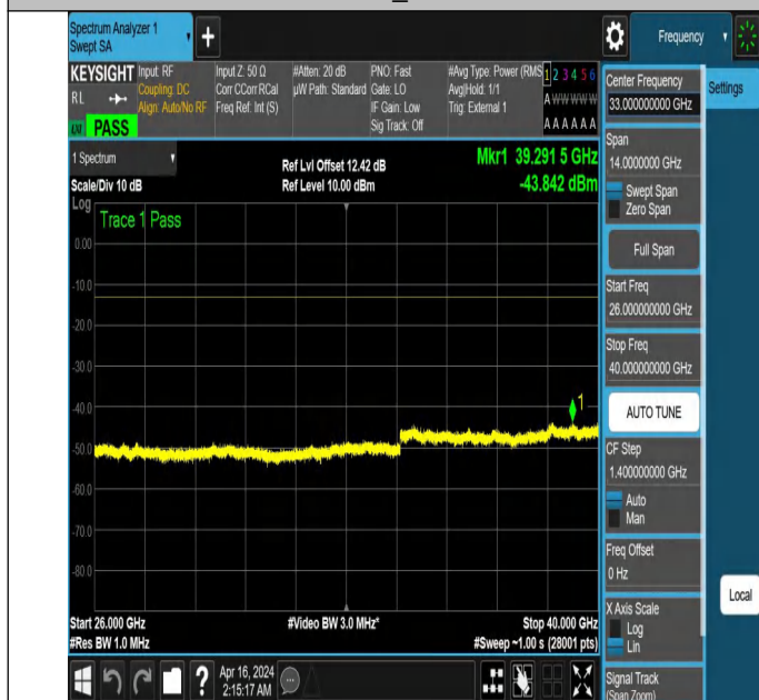
NTNV_N77-3700-3980_PC2_30_60_L_TID2_NS_01_26000_400
