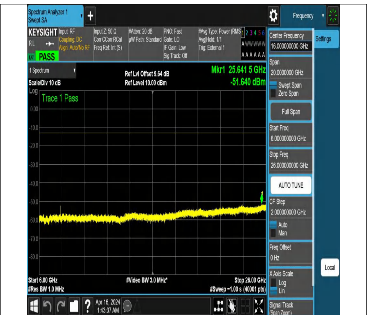
NTNV_N77-3700-3980_PC2_30_50_H_TID2_NS_01_6000_2600
