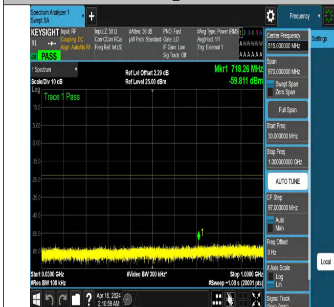
NTNV_N77-3700-3980_PC2_30_60_L_TID2_NS_01_30_1000_#
