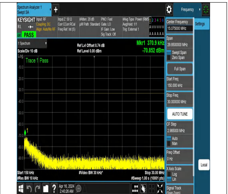
NTNV_N77-3700-3980_PC2_30_60_M_TID2_NS_01_0.15_30_#
