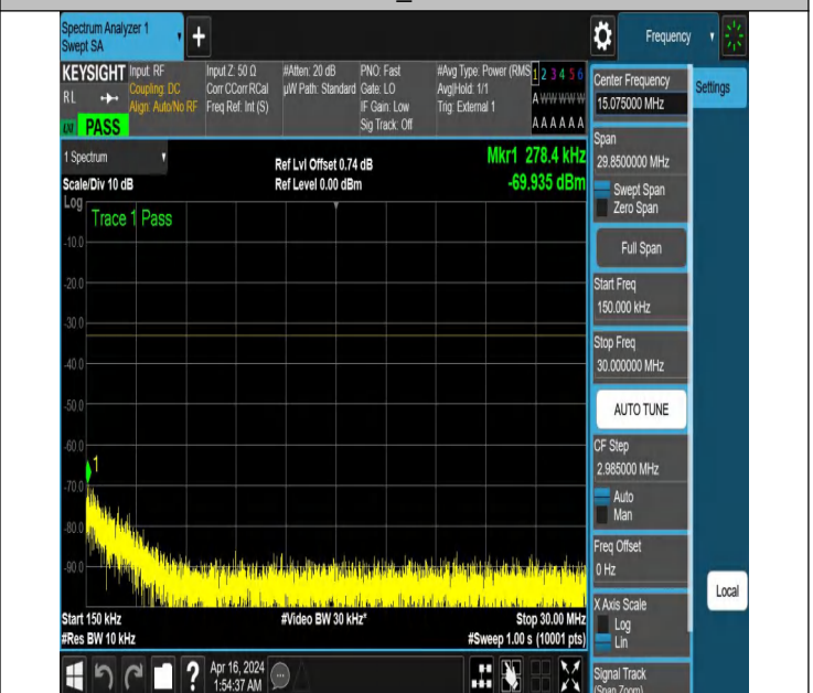
NTNV_N77-3700-3980_PC2_30_50_H_TID5_NS_01_0.15_30_# 1
