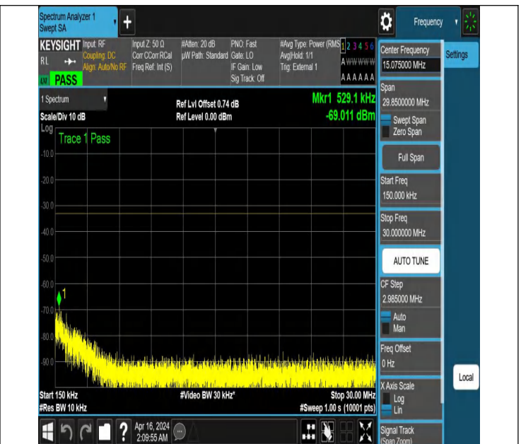
NTNV_N77-3700-3980_PC2_30_60_L_TID2_NS_01_0.15_30_#
