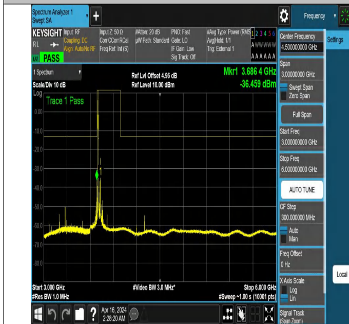
NTNV_N77-3700-3980_PC2_30_60_L_TID5_NS_01_3000_6000
