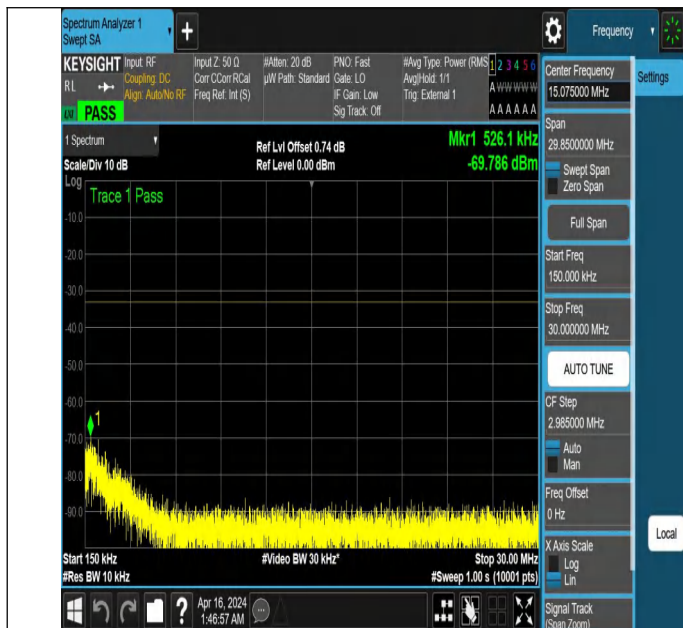
NTNV_N77-3700-3980_PC2_30_50_H_TID3_NS_01_0.15_30_#
