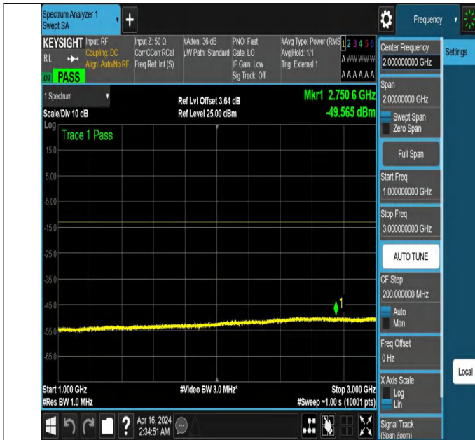
NTNV_N77-3700-3980_PC2_30_60_L_TID6_NS_01_1000_3000
