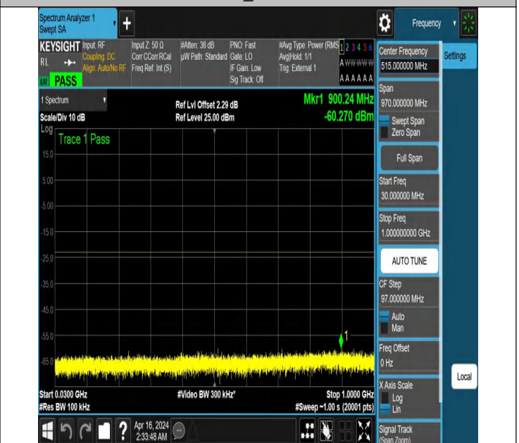
NTNV_N77-3700-3980_PC2_30_60_L_TID6_NS_01_30_1000_#
