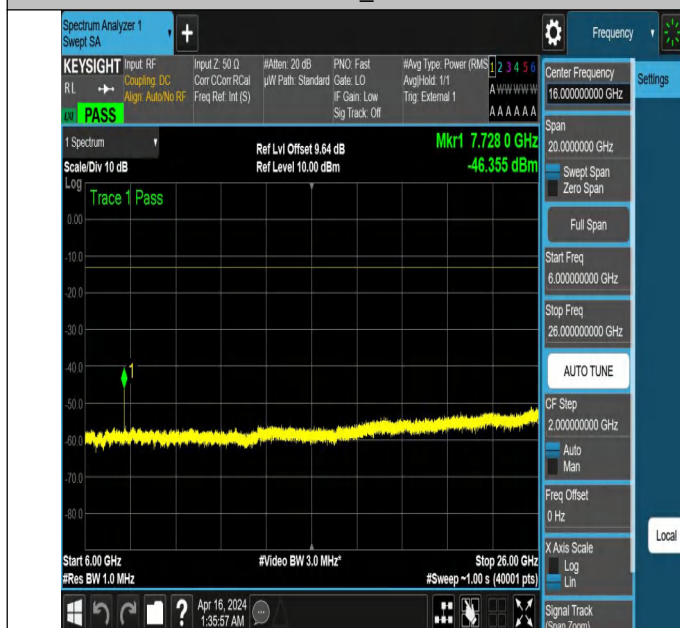
NTNV_N77-3700-3980_PC2_30_50_M_TID6_NS_01_6000_260
