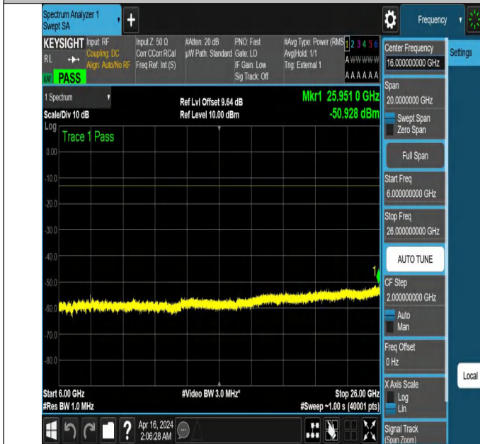
NTNV_N77-3700-3980_PC2_30_50_H_TID6_NS_01_6000_2600
