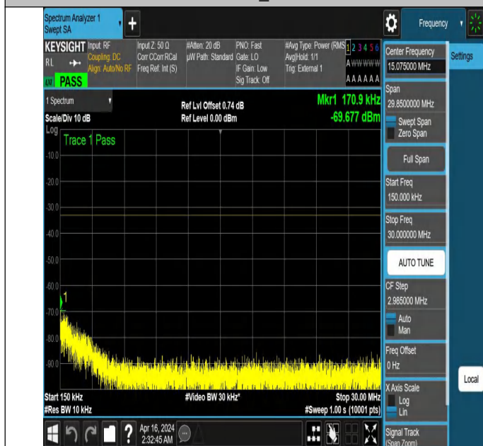
NTNV_N77-3700-3980_PC2_30_60_L_TID6_NS_01_0.15_30_#
