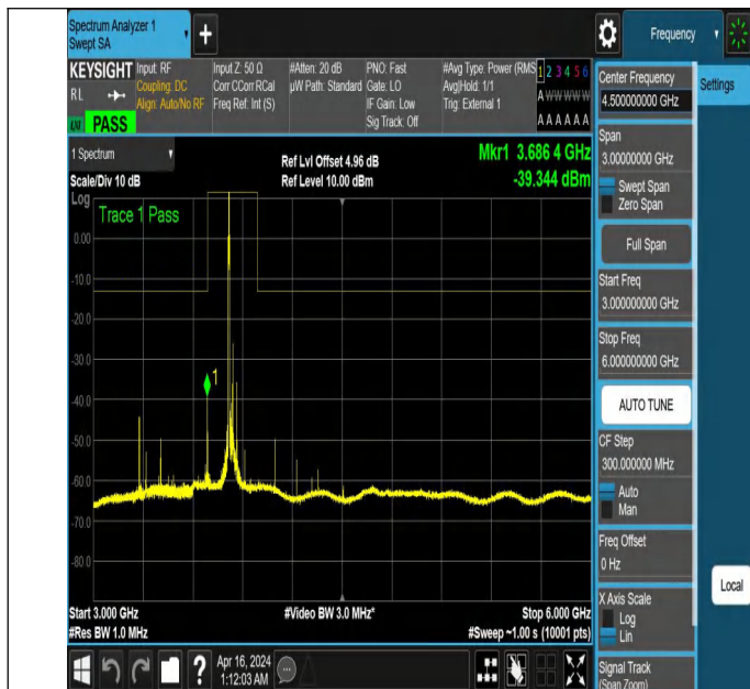
NTNV_N77-3700-3980_PC2_30_50_M_TID2_NS_01_3000_600
