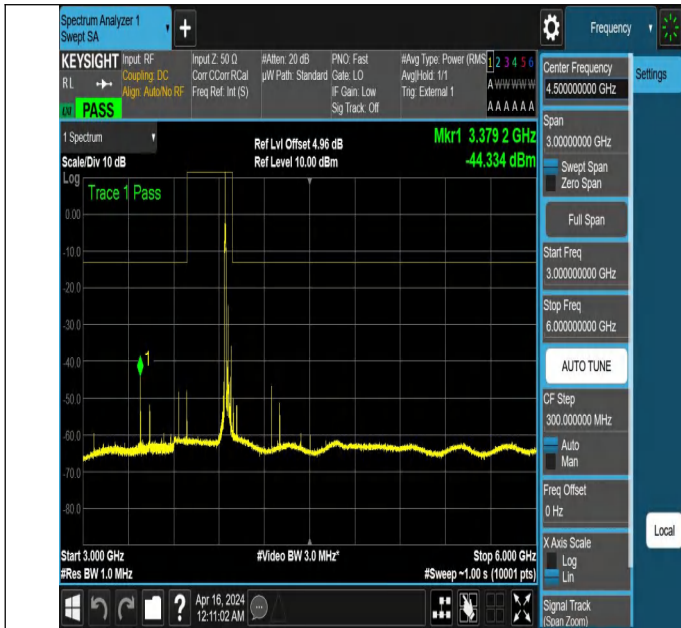
NTNV_N77-3700-3980_PC2_30_40_H_TID2_NS_01_3000_6000
