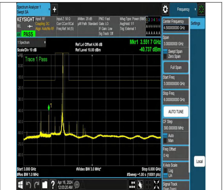
NTNV_N77-3700-3980_PC2_30_40_M_TID6_NS_01_3000_600
