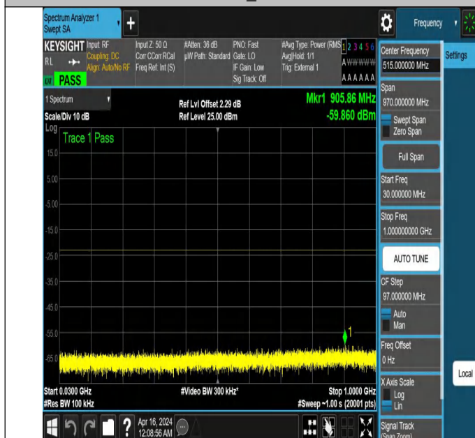
NTNV_N77-3700-3980_PC2_30_40_H_TID2_NS_01_30_1000_#
