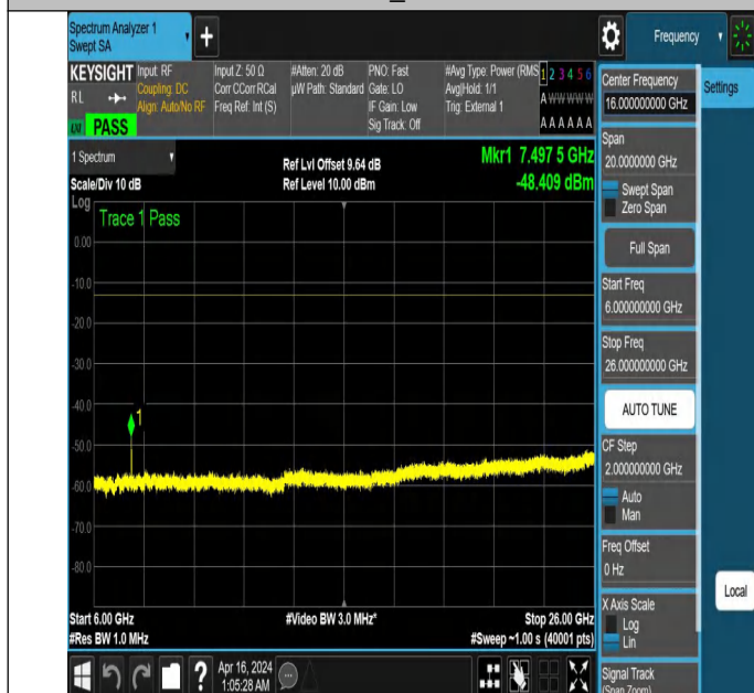
NTNV_N77-3700-3980_PC2_30_50_L_TID6_NS_01_6000_2600
