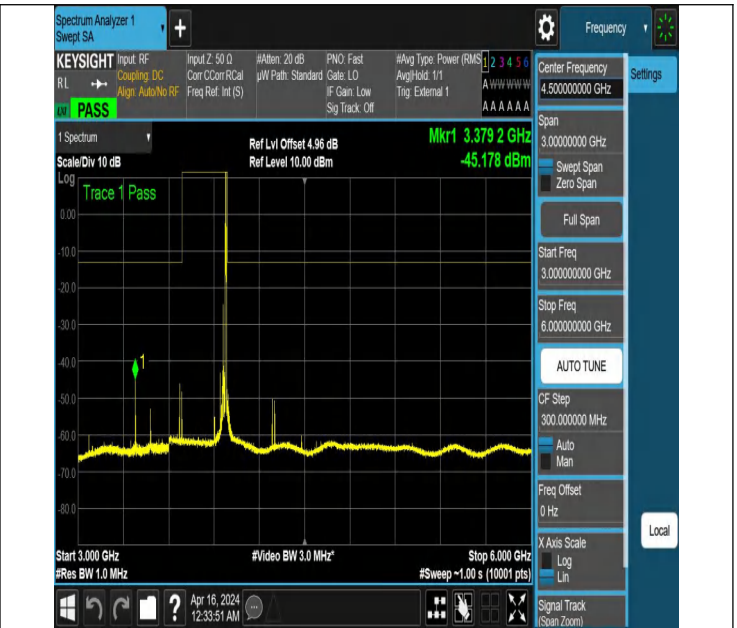
NTNV_N77-3700-3980_PC2_30_40_H_TID6_NS_01_3000_6000
