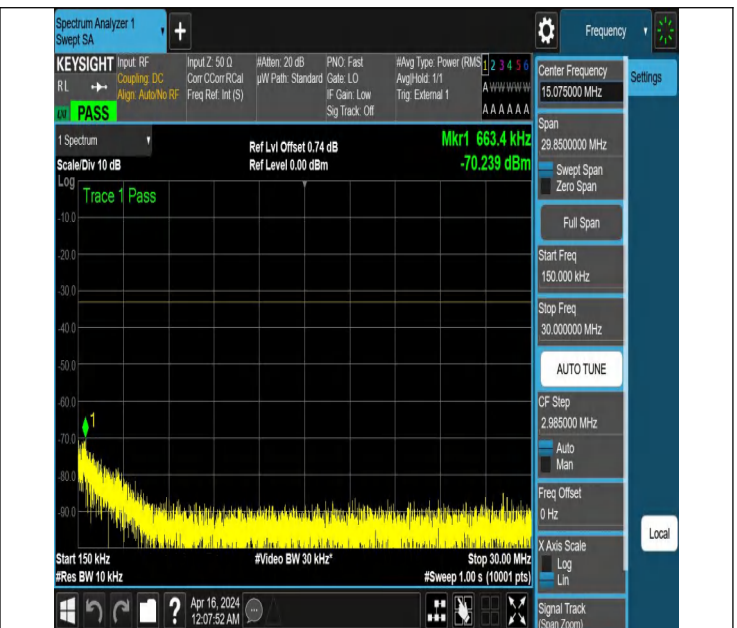
NTNV_N77-3700-3980_PC2_30_40_H_TID2_NS_01_0.15_30_#
