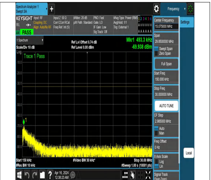
NTNV_N77-3700-3980_PC2_30_50_L_TID2_NS_01_0.15_30_#
