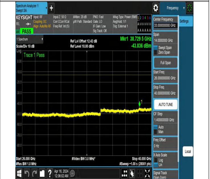
NTNV_N77-3700-3980_PC2_30_40_H_TID6_NS_01_26000_400
