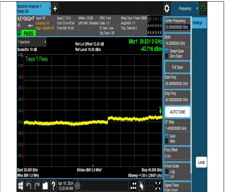
NTNV_N77-3700-3980_PC2_30_40_H_TID3_NS_01_26000_400
