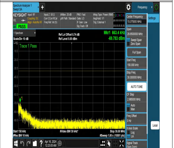
NTNV_N77-3700-3980_PC2_30_40_H_TID5_NS_01_0.15_30_#
