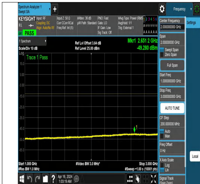
NTNV_N77-3700-3980_PC2_30_50_L_TID6 NS_01_1000_3000
