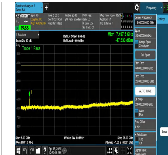
NTNV_N77-3700-3980_PC2_30_50_L_TID3_NS_01_6000_2600
