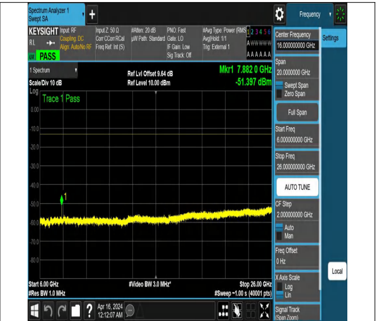
NTNV_N77-3700-3980_PC2_30_40_H_TID2_NS_01_6000_2600
