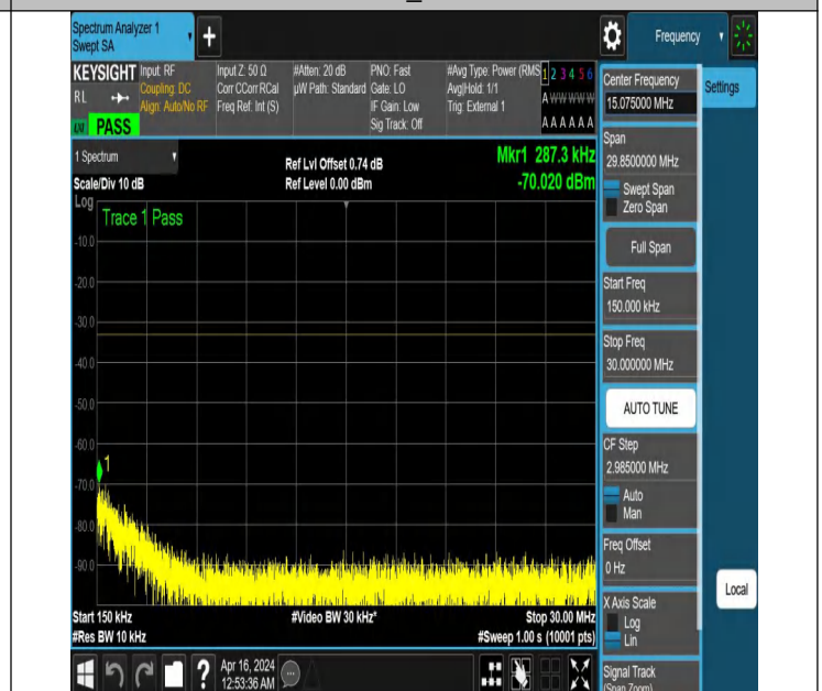
NTNV_N77-3700-3980_PC2_30_50_L_TID5_NS_01_0.15_30_#
