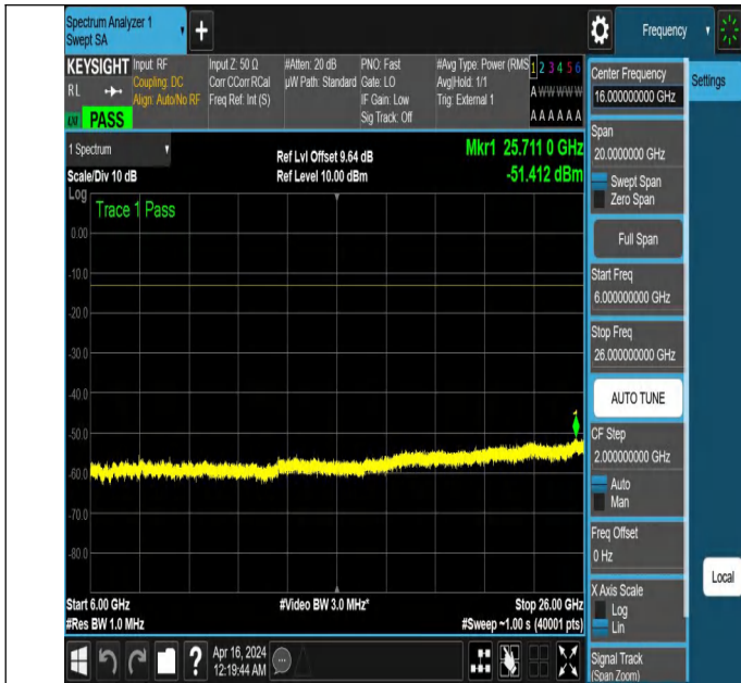
NTNV_N77-3700-3980_PC2_30_40_H_TID3_NS_01_6000_2600
