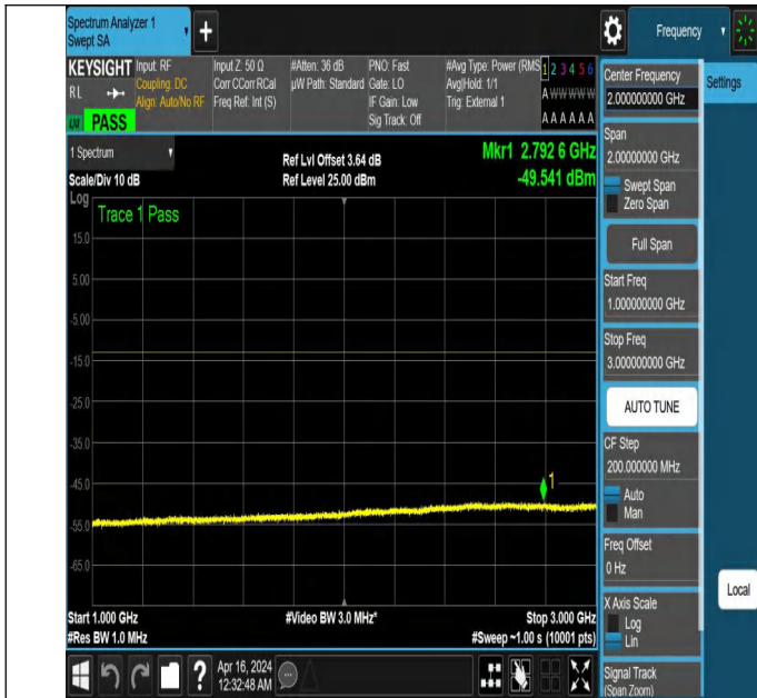
NTNV_N77-3700-3980_PC2_30_40_H_TID6_NS_01_1000_3000
