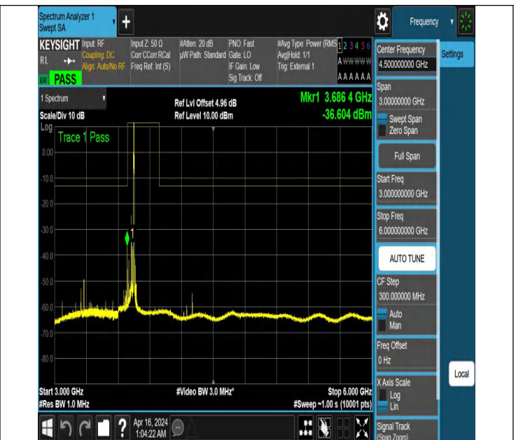
NTNV_N77-3700-3980_PC2_30_50_L_TID6_NS_01_3000_6000
