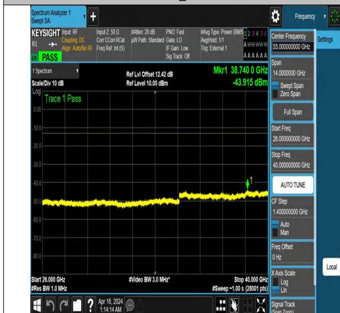
NTNV_N77-3700-3980_PC2_30_50_M_TID2_NS_01_26000_40 000 #1
