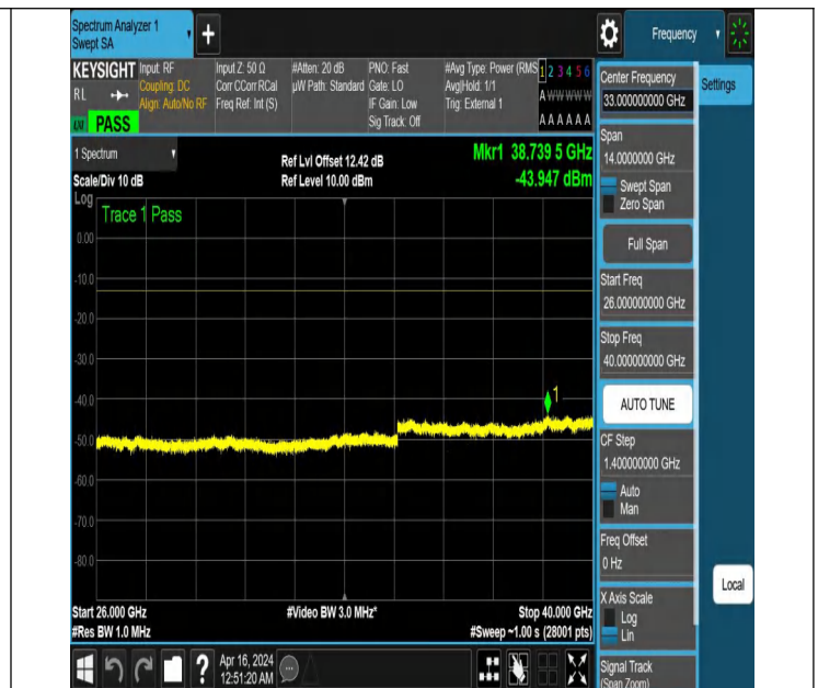
NTNV_N77-3700-3980_PC2_30_50_L_TID3_NS_01_26000_400
