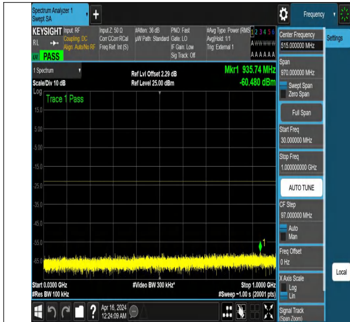
NTNV_N77-3700-3980_PC2_30_40_H_TID5_NS_01_30_1000_#
