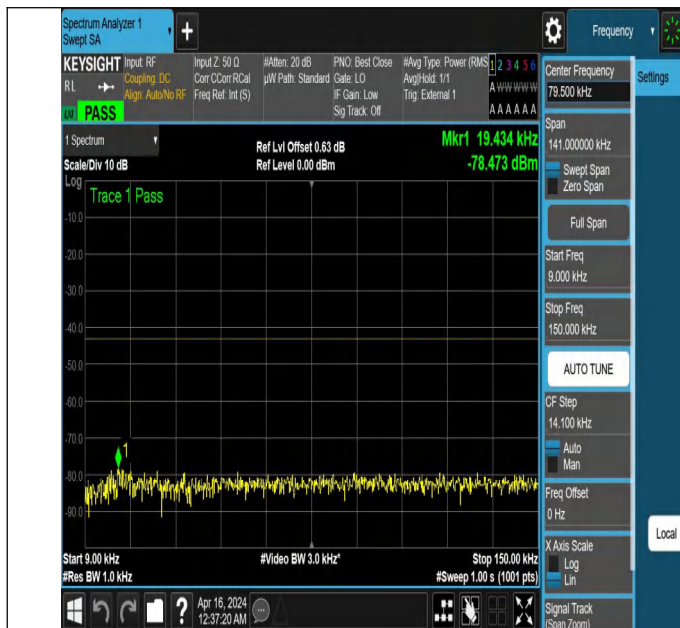
NTNV_N77-3700-3980_PC2_30_50_L_TID2_NS_01_0.009_0.15
