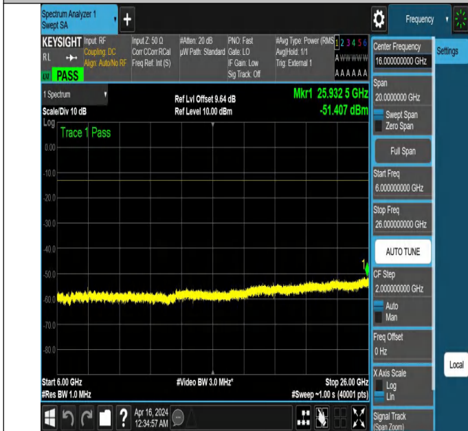
NTNV_N77-3700-3980_PC2_30_40_H_TID6_NS_01_6000_2600
