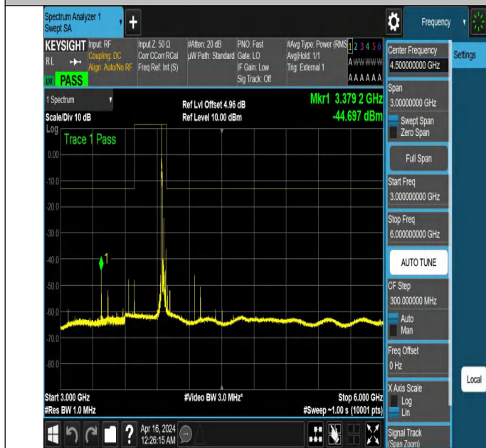
NTNV_N77-3700-3980_PC2_30_40_H_TID5_NS_01_3000_6000
