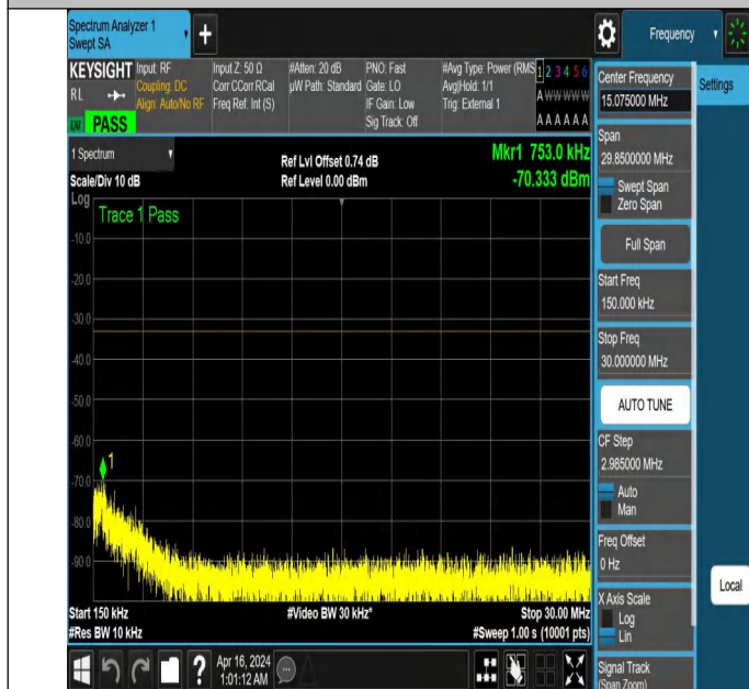
NTNV_N77-3700-3980_PC2_30_50_L_TID6_NS_01_0.15_30_#
