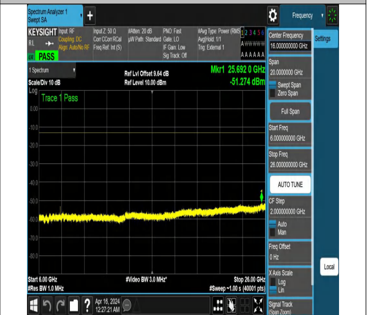
NTNV_N77-3700-3980_PC2_30_40_H_TID5_NS_01_6000_2600
