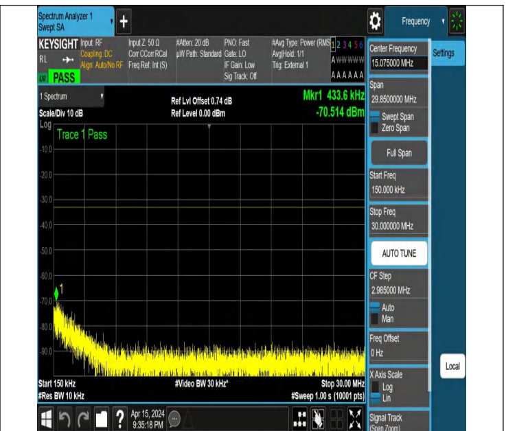
NTNV_N77-3700-3980_PC2_30_30_L_TID2_NS_01_0.15_30_#
