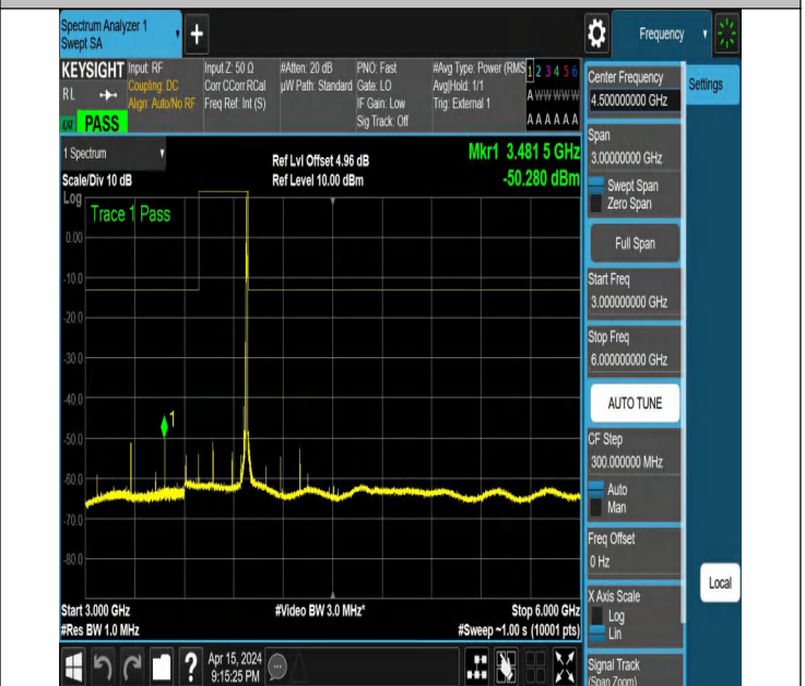
NTNV_N77-3700-3980_PC2_30_20_H_TID3_NS_01_3000_6000
