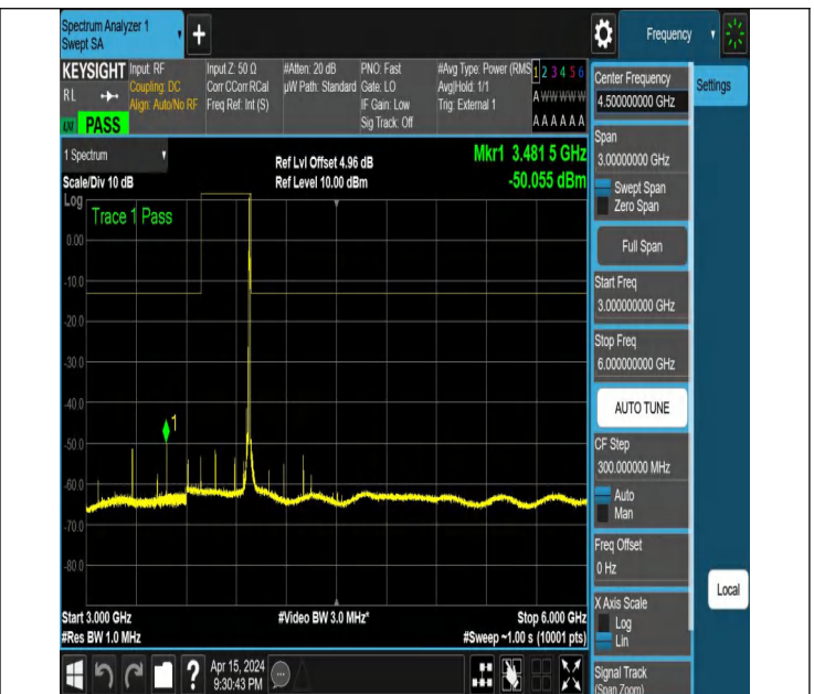
NTNV_N77-3700-3980_PC2_30_20_H_TID6_NS_01_3000_6000
