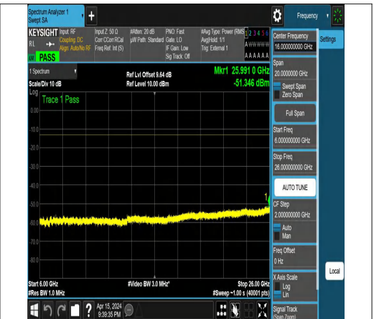
NTNV_N77-3700-3980_PC2_30_30_L_TID2_NS_01_6000_2600
