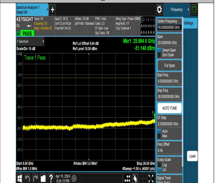
NTNV_N77-3700-3980_PC2_30_20_H_TID5_NS_01_6000_2600
