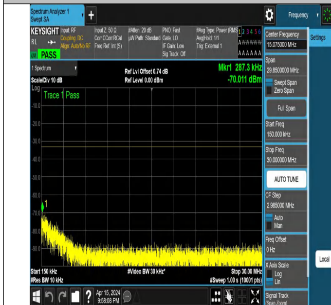
NTNV_N77-3700-3980_PC2_30_30_L_TID6_NS_01_0.15_30_#
