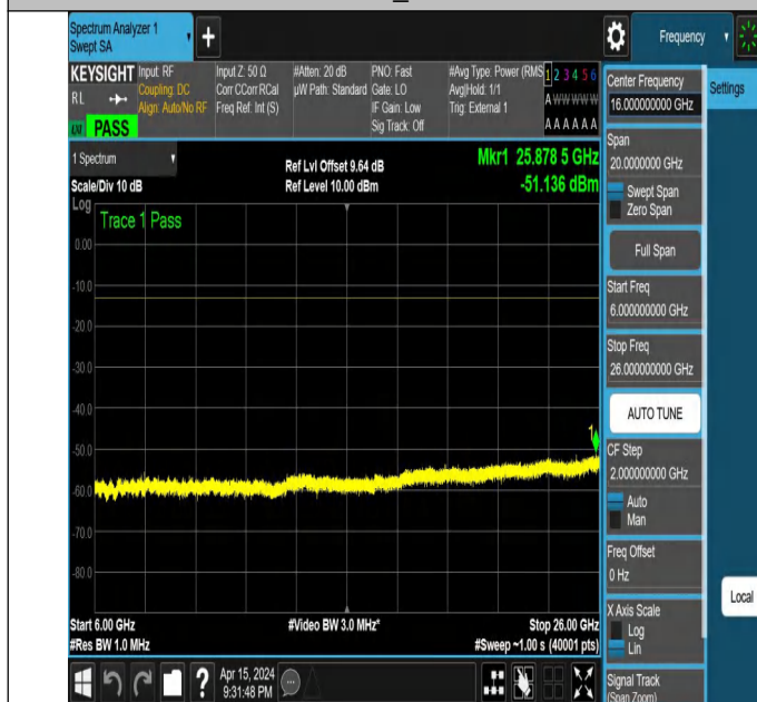
NTNV_N77-3700-3980_PC2_30_20_H_TID6_NS_01_6000_2600
