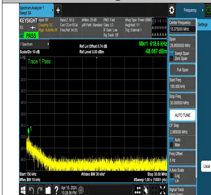
NTNV_N77-3700-3980_PC2_30_30_M_TID6_NS_01_0.15_30_#
