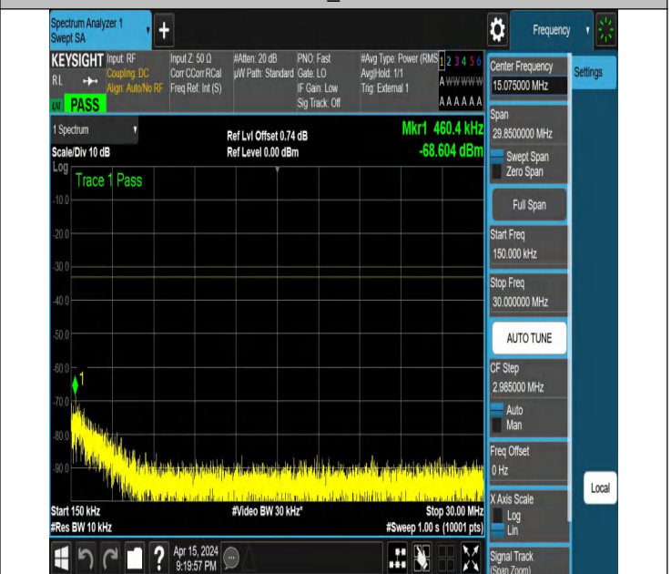
NTNV_N77-3700-3980_PC2_30_20_H_TID5_NS_01_0.15_30_# 1
