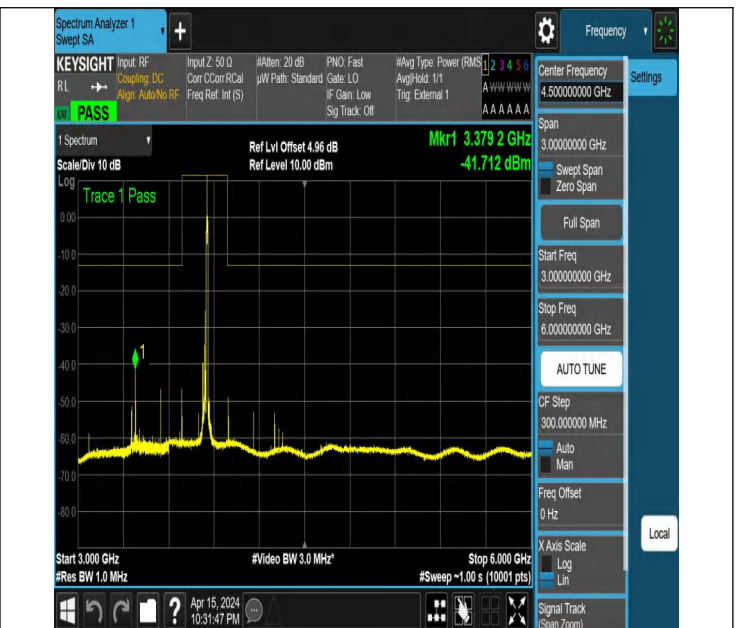
NTNV_N77-3700-3980_PC2_30_30_M_TID6_NS_01_3000_600
