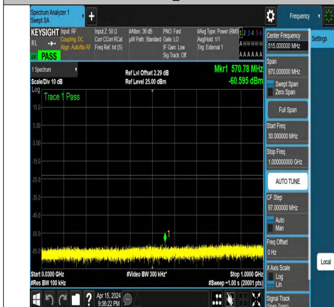
NTNV_N77-3700-3980_PC2_30_30_L_TID2_NS_01_30_1000_#
