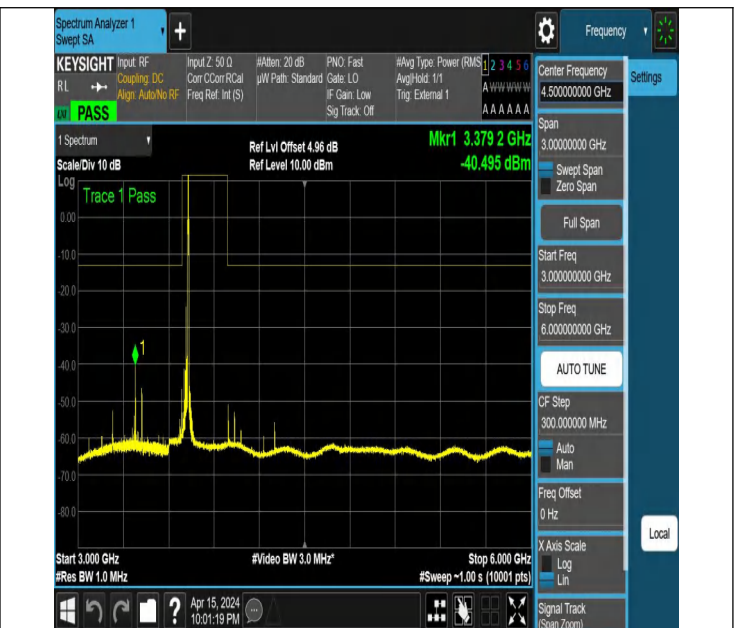
NTNV_N77-3700-3980_PC2_30_30_L_TID6_NS_01_3000_6000
