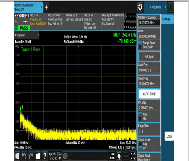
NTNV_N77-3700-3980_PC2_30_30_L_TID5_NS_01_0.15_30_#
