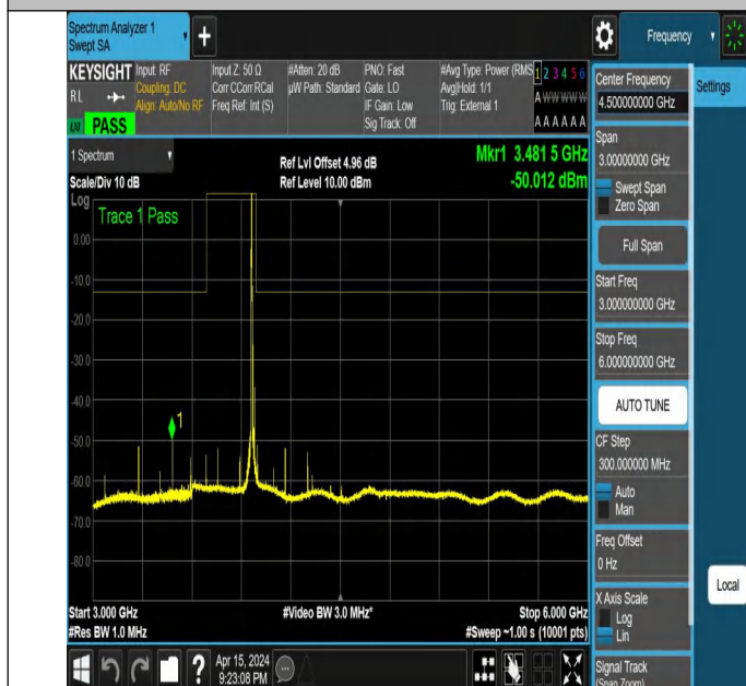
NTNV_N77-3700-3980_PC2_30_20_H_TID5_NS_01_3000_6000
