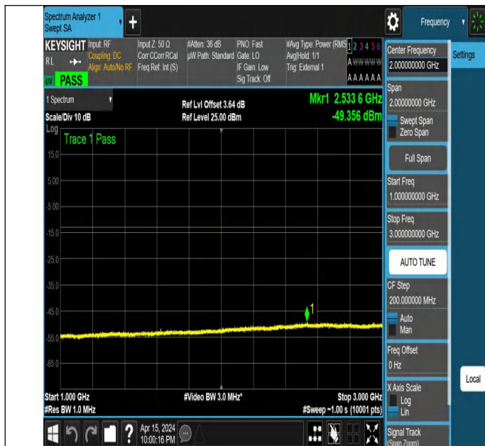
NTNV_N77-3700-3980_PC2_30_30_L_TID6 NS_01_1000_3000
