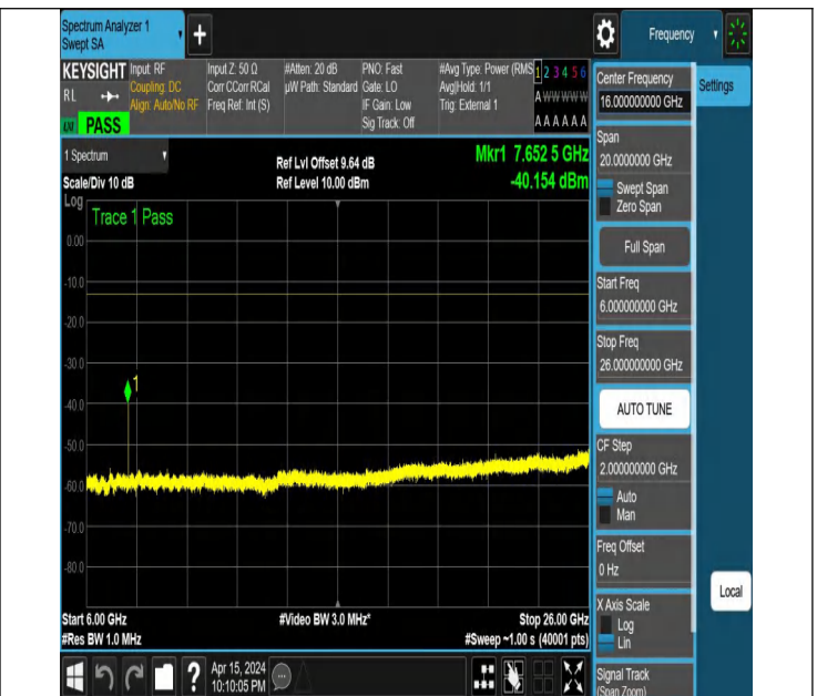
NTNV_N77-3700-3980_PC2_30_30_M_TID2_NS_01_6000_260
