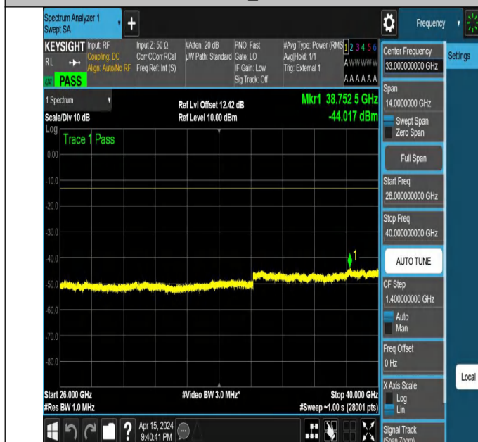
NTNV_N77-3700-3980_PC2_30_30_L_TID2_NS_01_26000_400
