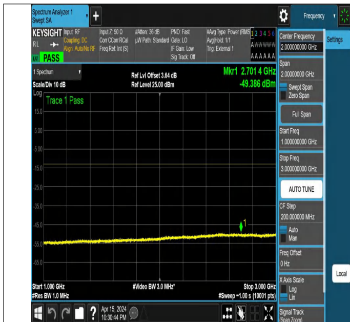
NTNV_N77-3700-3980_PC2_30_30_M_TID6_NS_01_1000_300
