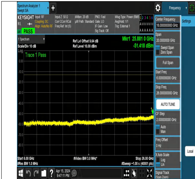
NTNV_N77-3700-3980_PC2_30_30_L_TID3_NS_01_6000_2600
