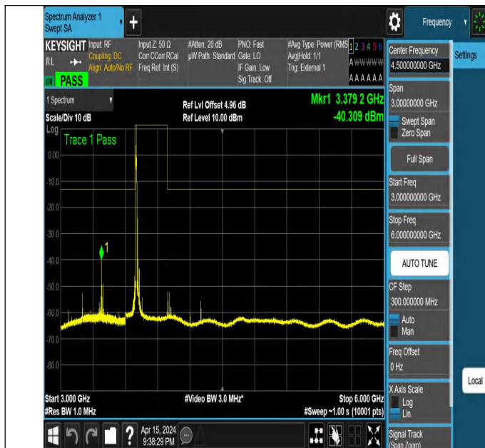
NTNV_N77-3700-3980_PC2_30_30_L_TID2_NS_01_3000_6000
