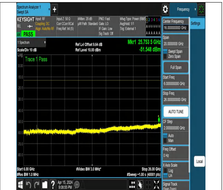
NTNV_N77-3700-3980_PC2_30_20_H_TID2_NS_01_6000_2600
