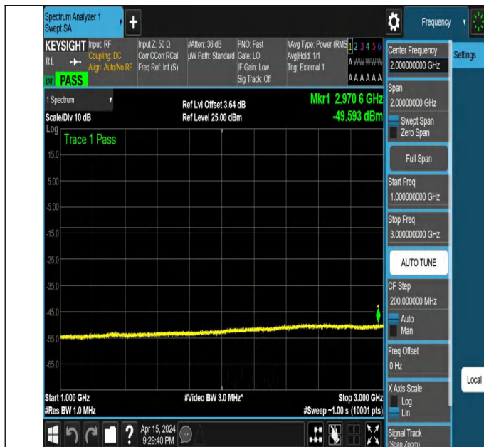
NTNV_N77-3700-3980_PC2_30_20_H_TID6 NS_01_1000_3000
