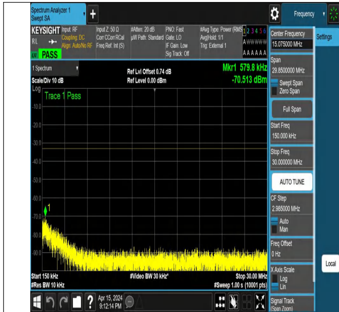
NTNV_N77-3700-3980_PC2_30_20_H_TID3_NS_01_0.15_30_#
