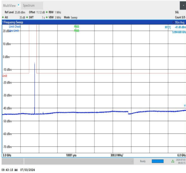
NTNV_DC_26A_n77A-3450-3550_PC2_30_5+80_M+L_TID2_NS_01_3000_6000_#1
