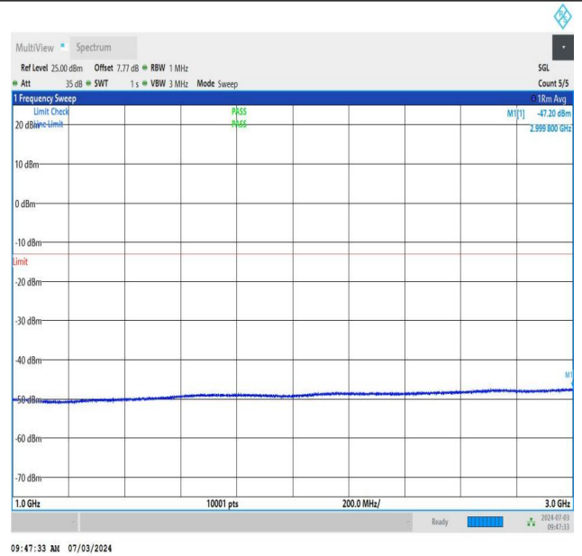
NTNV_DC_26A_n77A-3450-3550_PC2_30_5+80_M+M_TID2_N S_01_1000_3000_#1
