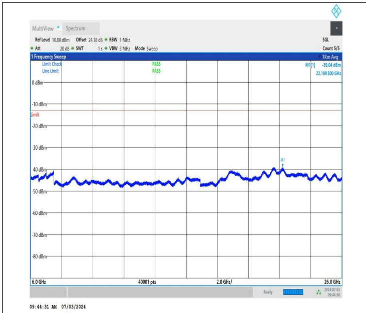
NTNV_DC_26A_n77A-3450-3550_PC2_30_5+80_M+L_TID4_NS _01_6000_26000_#1
