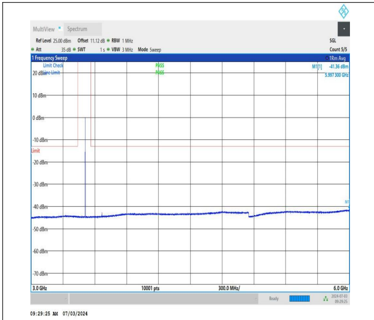
NTNV_DC_26A_n77A-3450-3550_PC2_30_5+60_M+L_TID2_NS_01_3000_6000_#1
