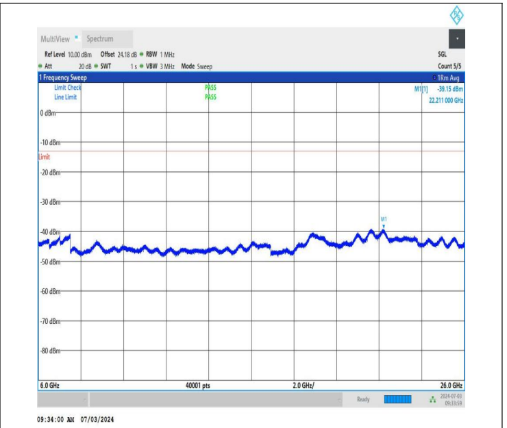
NTNV_DC_26A_n77A-3450-3550_PC2_30_5+60_M+M_TID2_N S_01_6000_26000_#1
