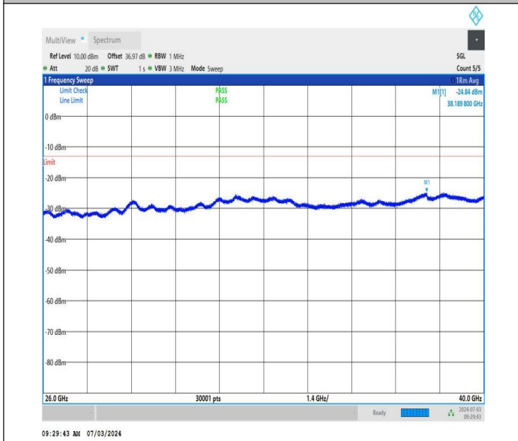
NTNV_DC_26A_n77A-3450-3550_PC2_30_5+60_M+L_TID2_NS_01_26000_40000_#1
