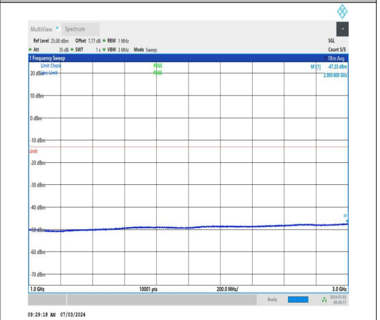
NTNV_DC_26A_n77A-3450-3550_PC2_30_5+60_M+L_TID2_NS_01_1000_3000_#1
