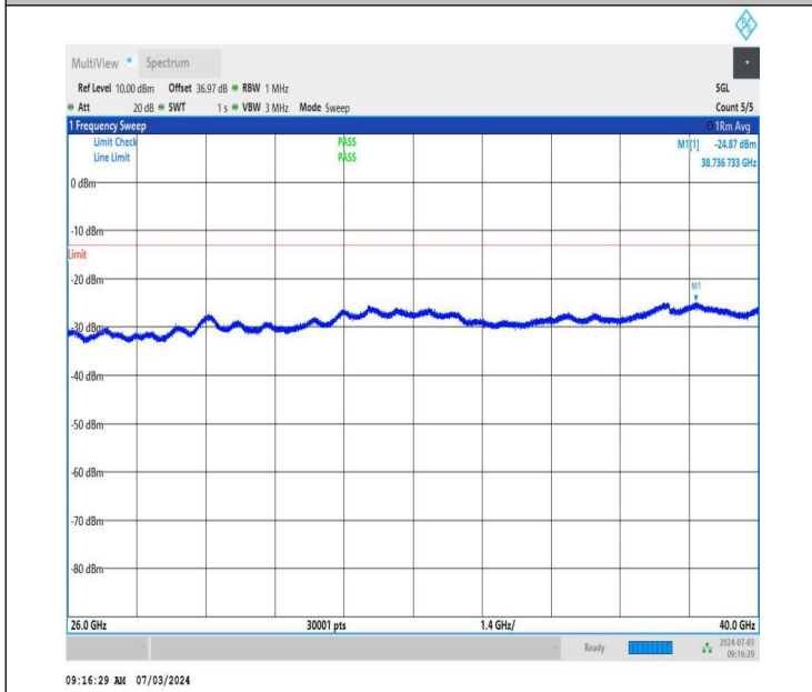
NTNV_DC_26A_n77A-3450-3550_PC2_30_5+50_M+L_TID2_NS_01_26000_40000_#1
