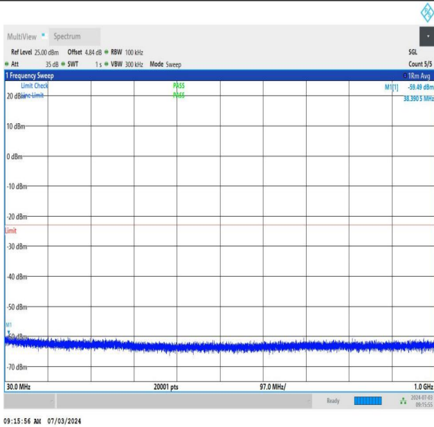
NTNV_DC_26A_n77A-3450-3550_PC2_30_5+50_M+L_TID2_NS_01_30_1000_#1
