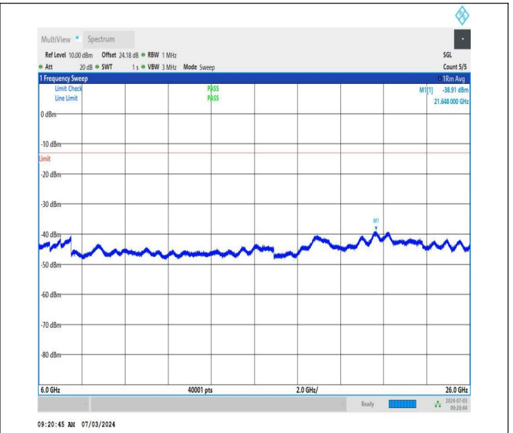
NTNV_DC_26A_n77A-3450-3550_PC2_30_5+50_M+M_TID2_N S_01_6000_26000_#1
