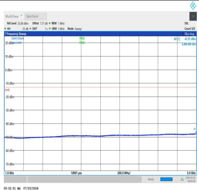
NTNV_DC_26A_n77A-3450-3550_PC2_30_5+40_M+L_TID2_NS_01_1000_3000_#1
