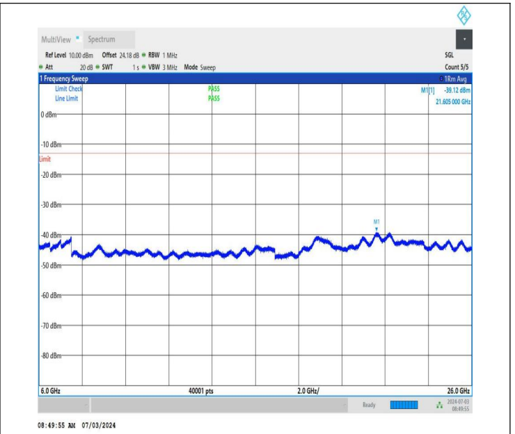
NTNV_DC_26A_n77A-3450-3550_PC2_30_5+30_M+L_TID2_NS_01_6000_26000_#1
