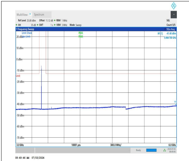
NTNV_DC_26A_n77A-3450-3550_PC2_30_5+30_M+L_TID2_NS_01_3000_6000_#1
