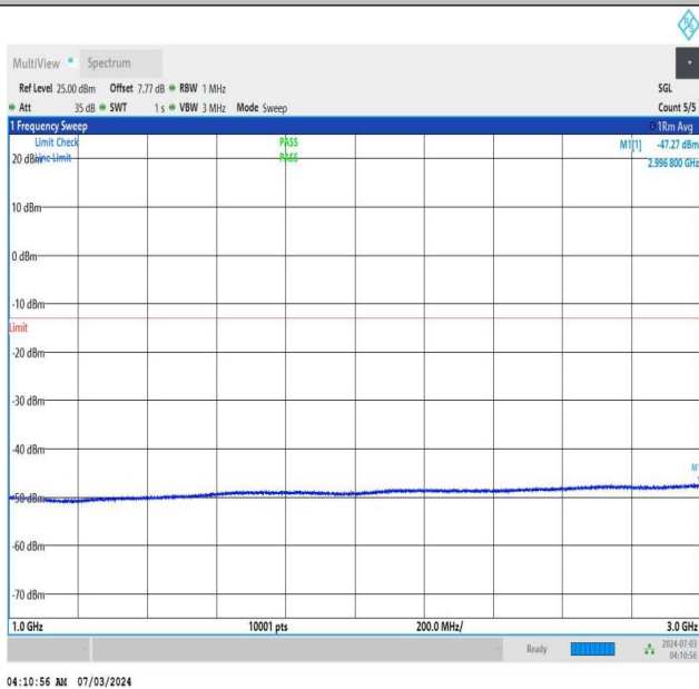
NTNV_DC_26A_n77A-3450-3550_PC2_30_5+20_M+L_TID2_NS _01_1000_3000_#1
