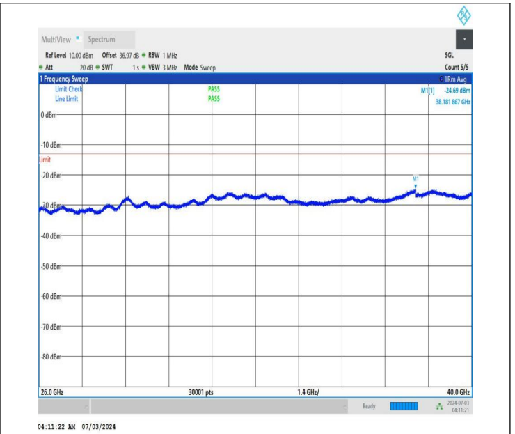
NTNV_DC_26A_n77A-3450-3550_PC2_30_5+20_M+L_TID2_NS_01_26000_40000_#1
