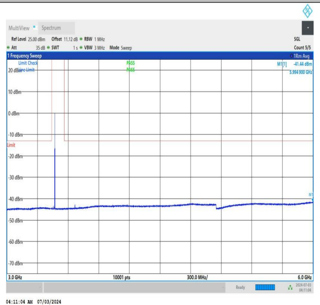
NTNV_DC_26A_n77A-3450-3550_PC2_30_5+20_M+L_TID2_NS _01_3000_6000_#1
