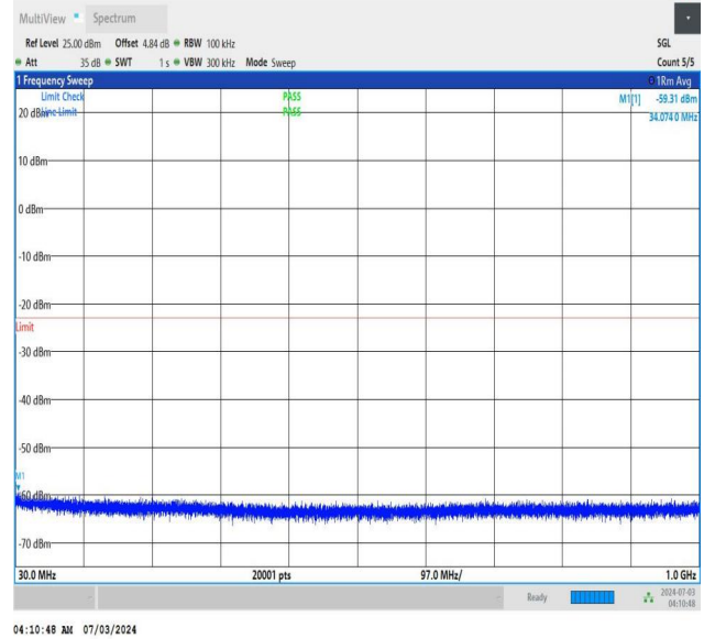
NTNV_DC_26A_n77A-3450-3550_PC2_30_5+20_M+L_TID2_NS _01_30_1000_#1
