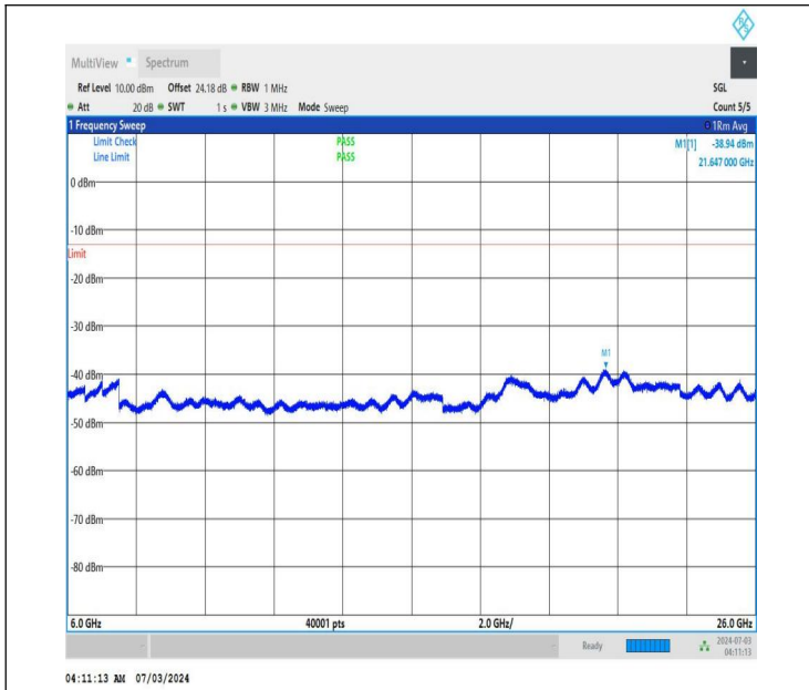
NTNV_DC_26A_n77A-3450-3550_PC2_30_5+20_M+L_TID2_NS_01_6000_26000_#1
