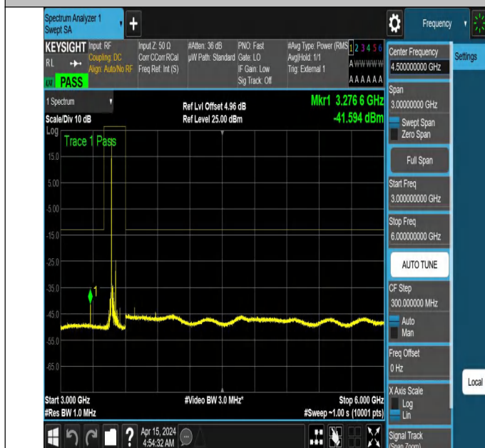
NTNV N77-3450-3550 PC2 30 80 H TID5 NS 01 3000 6000
