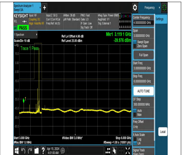
NTNV_N77-3450-3550_PC2_30_80_L_TID6_NS_01_3000_6000
