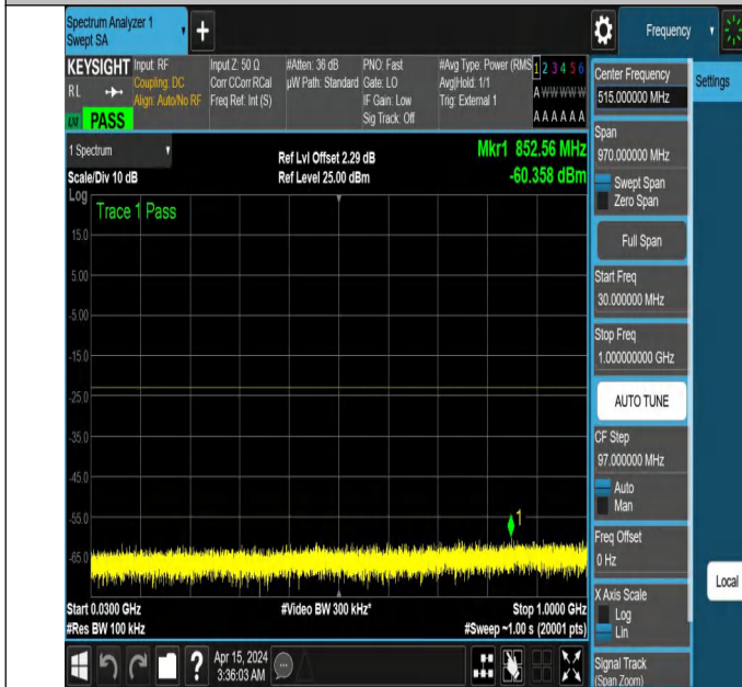
NTNV_N77-3450-3550_PC2_30_80_L_TID2_NS_01_30_1000_#
