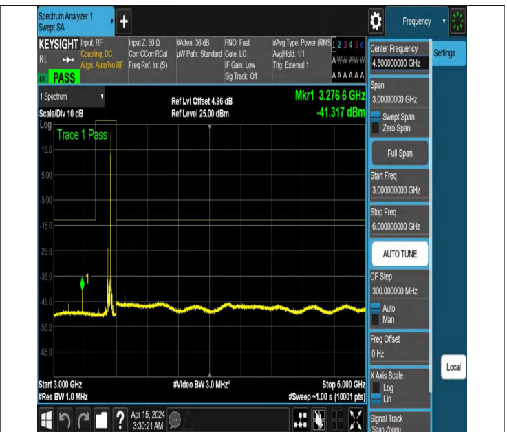
NTNV_N77-3450-3550_PC2_30_60_H_TID6_NS_01_3000_6000
