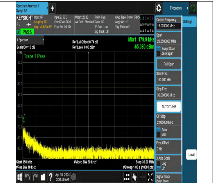
NTNV_N77-3450-3550_PC2_30_80_L_TID2_NS_01_0.15_30_#
