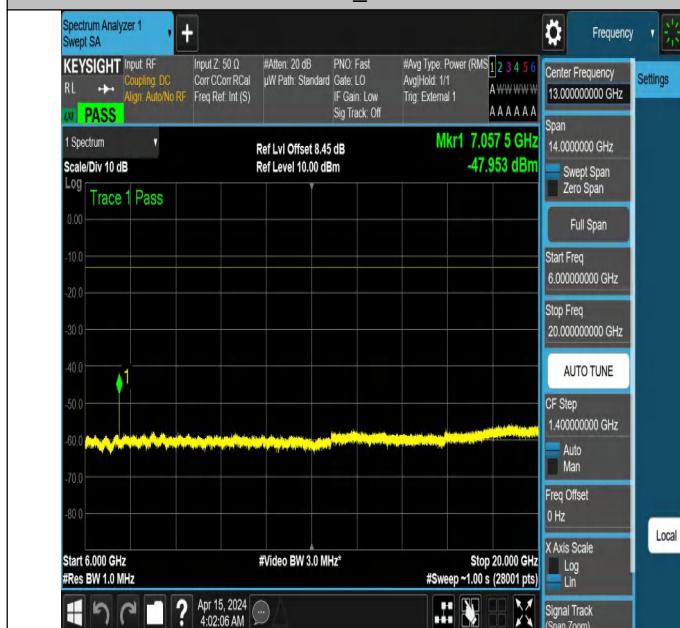
NTNV_N77-3450-3550_PC2_30_80_L_TID6_NS_01_6000_2000
