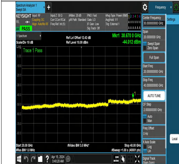
NTNV_N77-3450-3550_PC2_30_80_L_TID2_NS_01_20000_400
