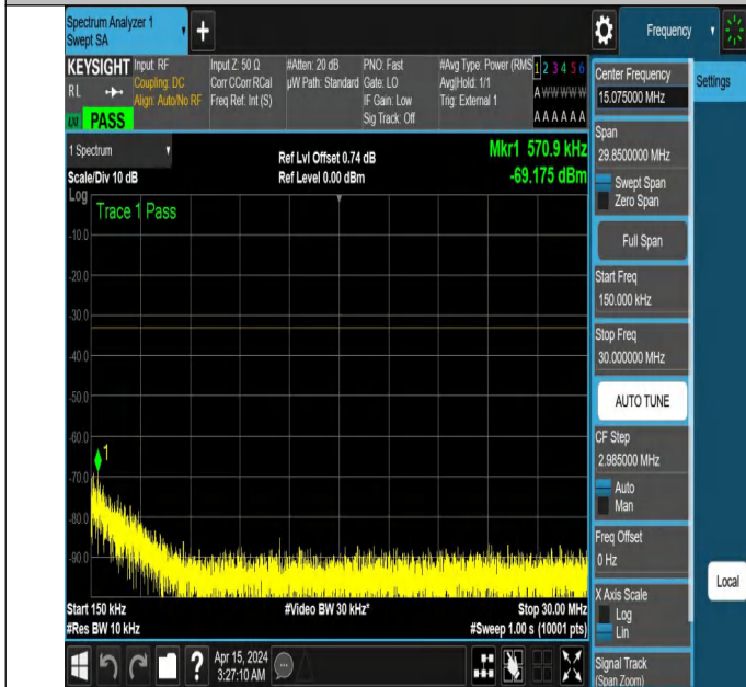
NTNV_N77-3450-3550_PC2_30_60_H_TID6_NS_01_0.15_30_#
