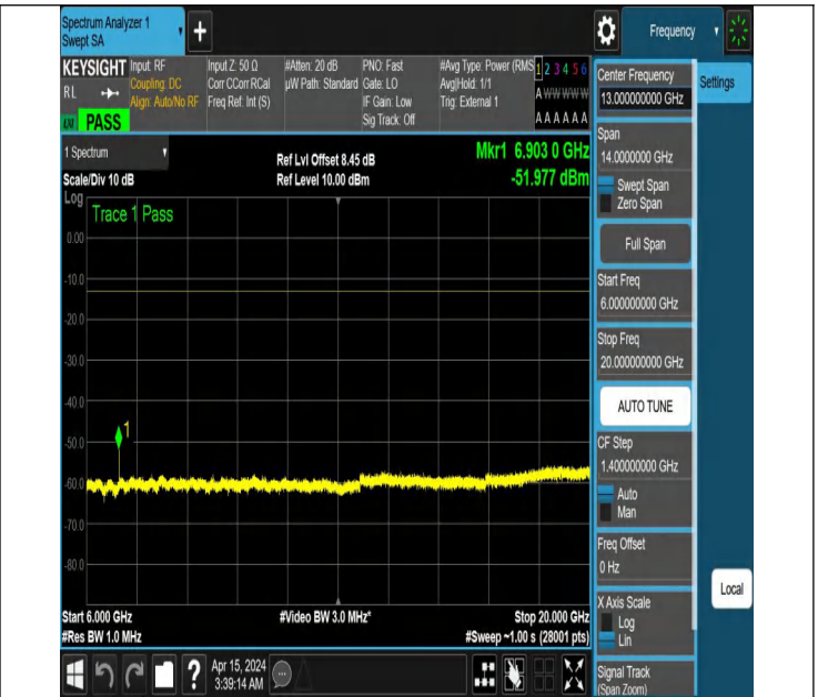
NTNV_N77-3450-3550_PC2_30_80_L_TID2_NS_01_6000_2000
