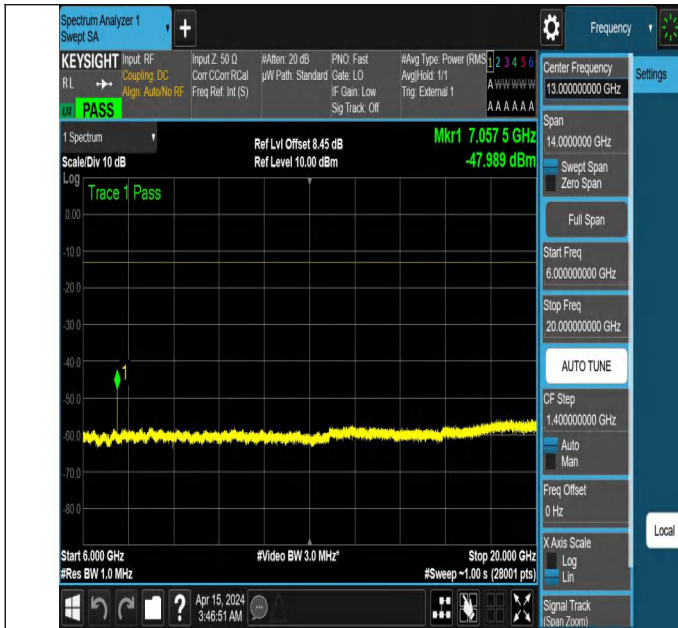
NTNV_N77-3450-3550_PC2_30_80_L_TID3_NS_01_6000_2000
