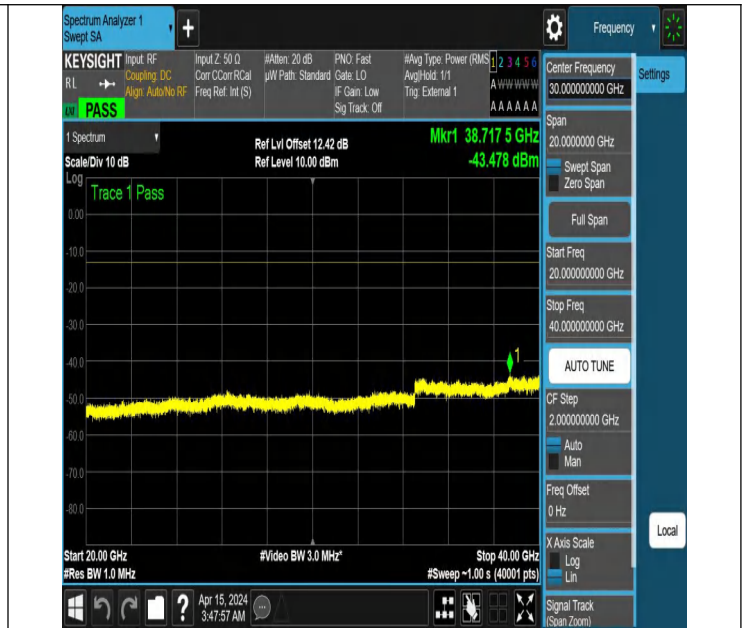
NTNV_N77-3450-3550_PC2_30_80_L_TID3_NS_01_20000_400
