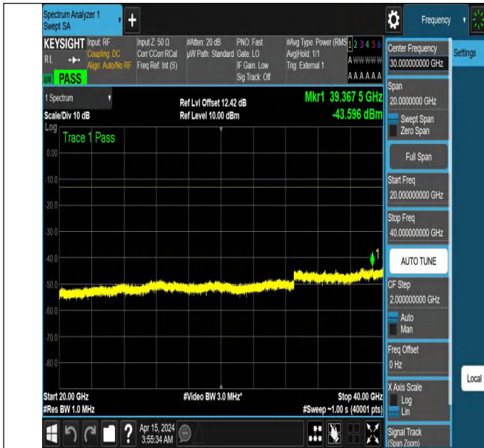
NTNV_N77-3450-3550_PC2_30_80_L_TID5_NS_01_20000_400
