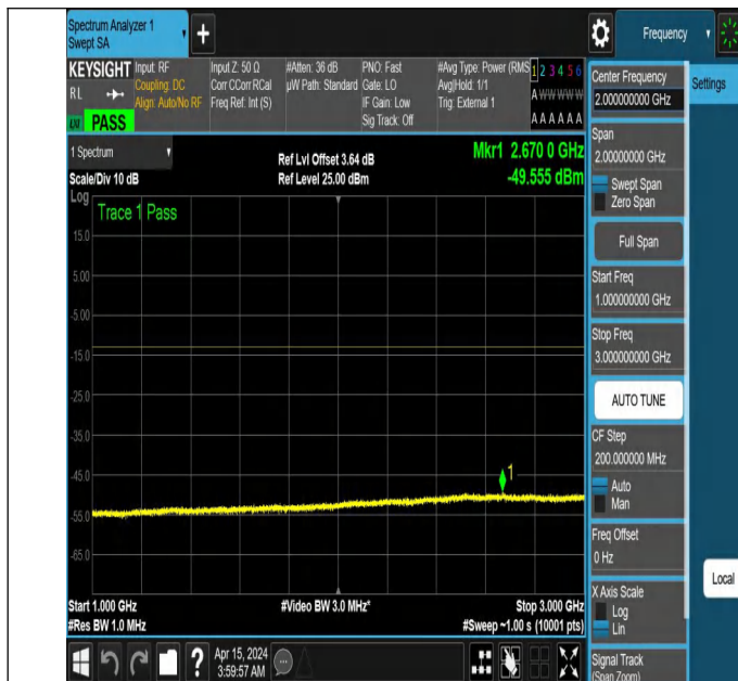
NTNV_N77-3450-3550_PC2_30_80_L_TID6 NS_01_1000_3000
